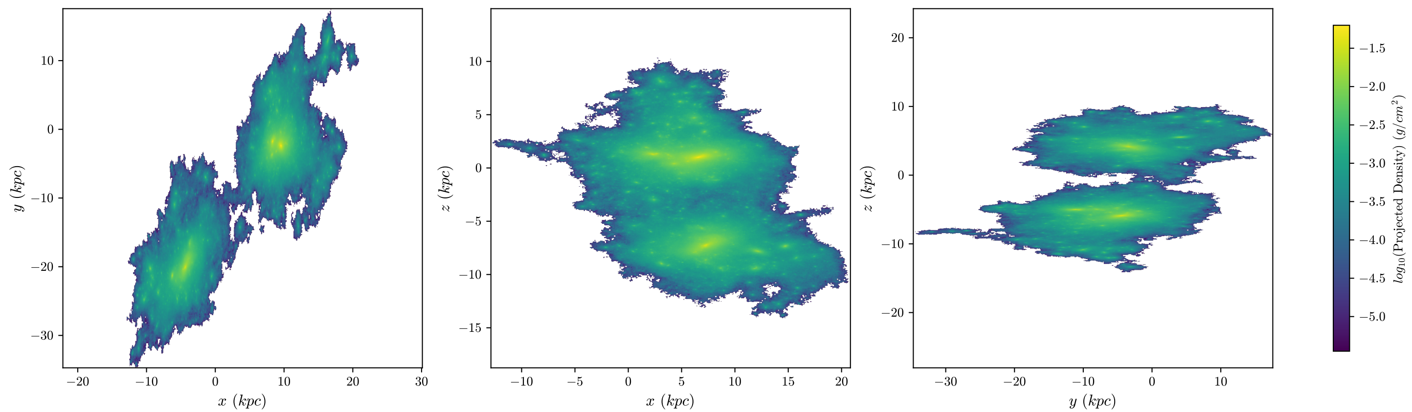
halo8 Stars, z = 2.544 , 512 bins
