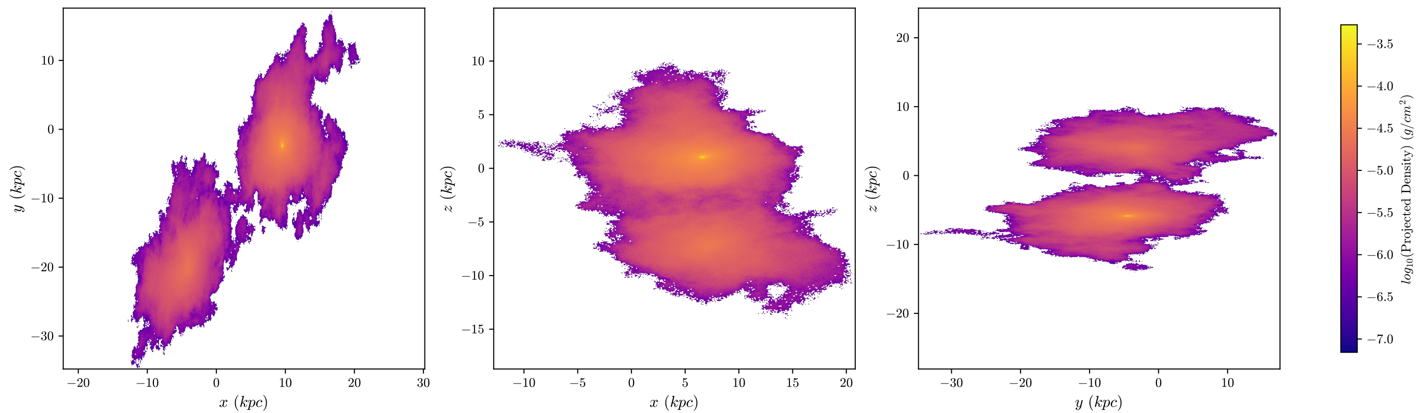
halo8 Dark Matter, z = 2.544 , 512 bins
