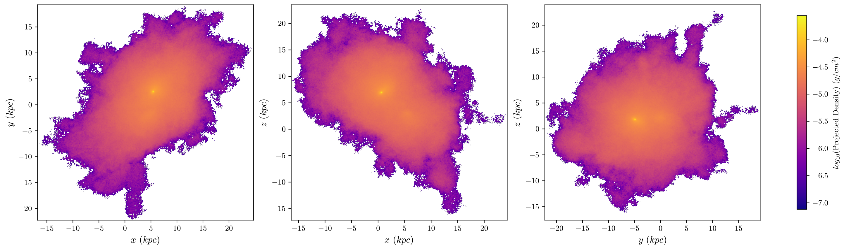
halo8 Dark Matter, z = 1.679 , 512 bins
