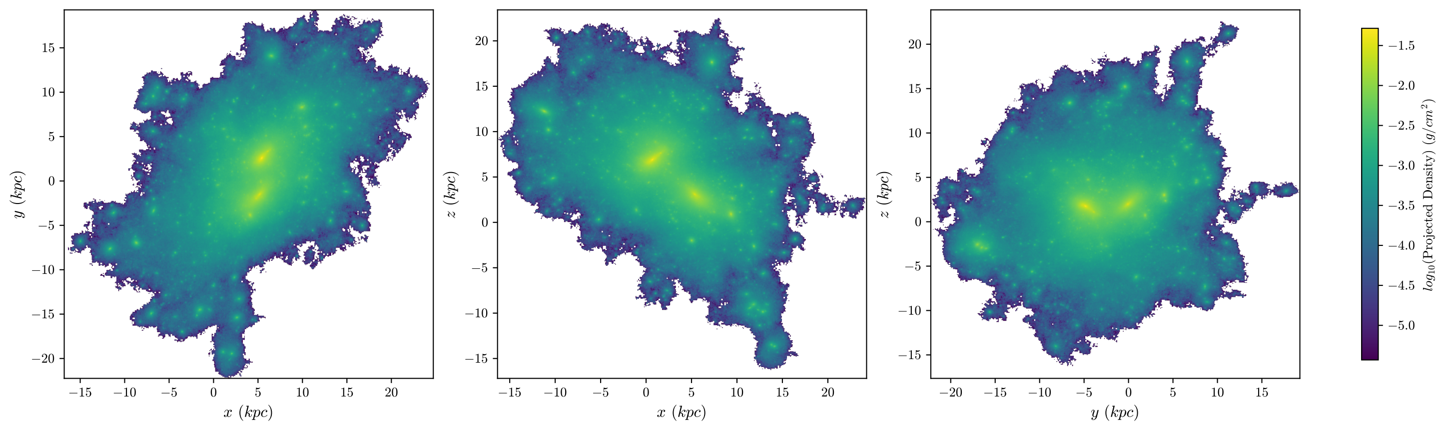
halo8 Stars, z = 1.679 , 512 bins
