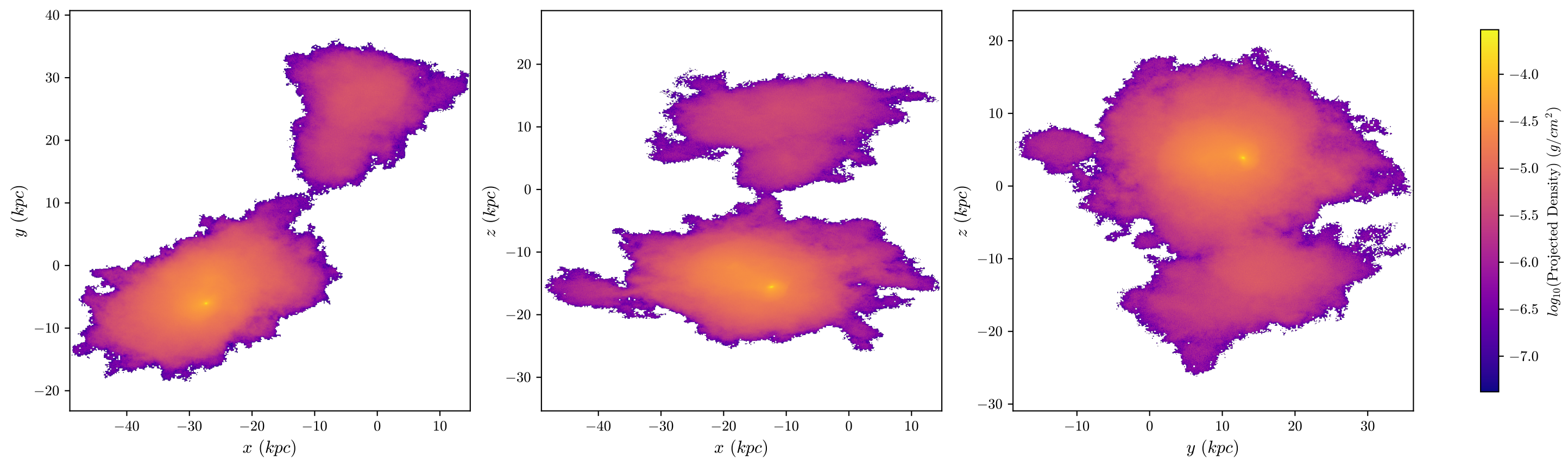
halo8 Dark Matter, z = 1.496 , 512 bins
