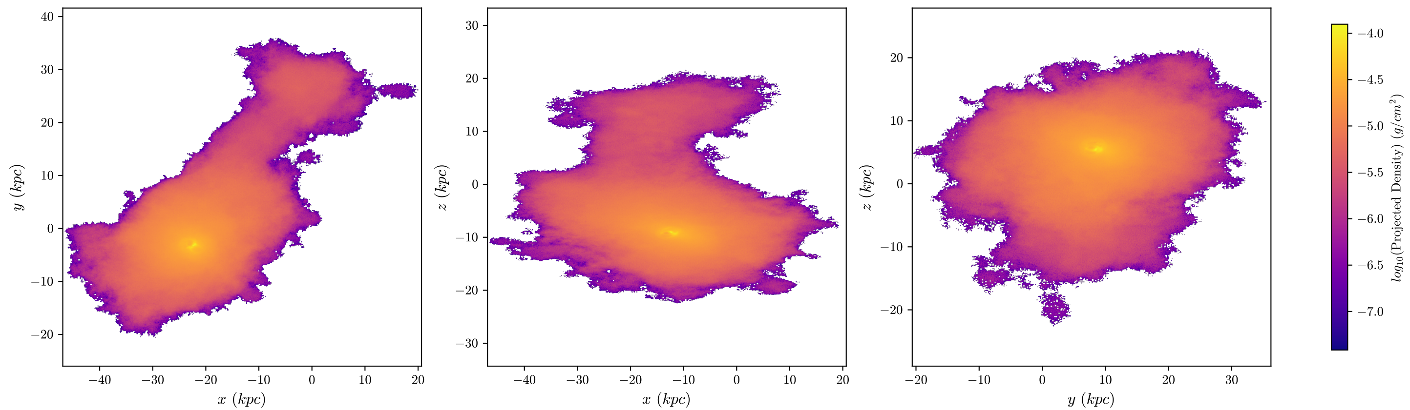
halo8 Dark Matter, z = 1.324 , 512 bins
