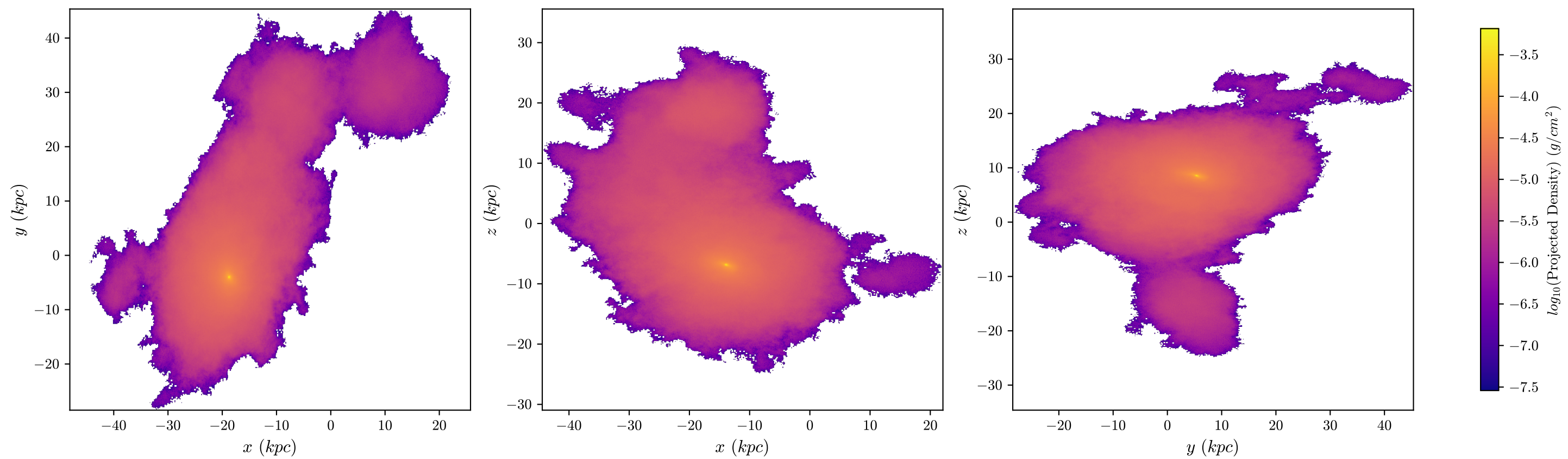
halo8 Dark Matter, z = 1.185 , 512 bins
