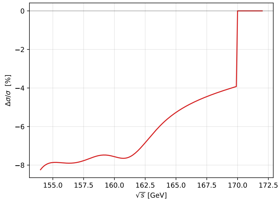
\sigma shift from K_C -safe fix (kcsafe=True vs False)
