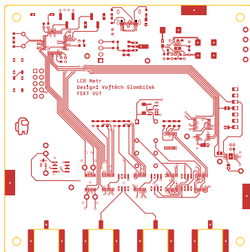
Obr. B.1: Vrstva Top
