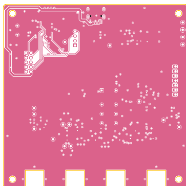
Obr. B.5: Vrstva In4
