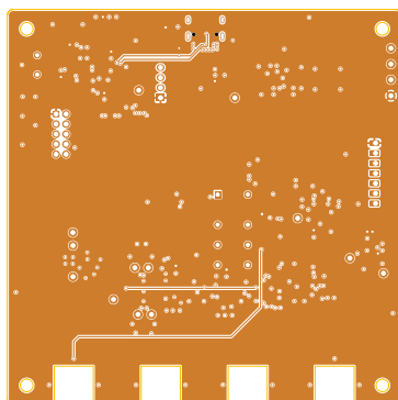
Obr. B.3: Vrstva In2
