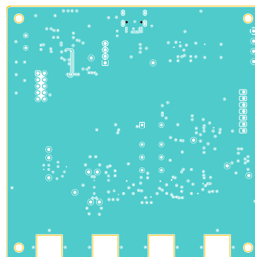
Obr. B.4: Vrstva In3
