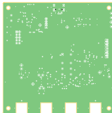
Obr. B.2: Vrstva In1
