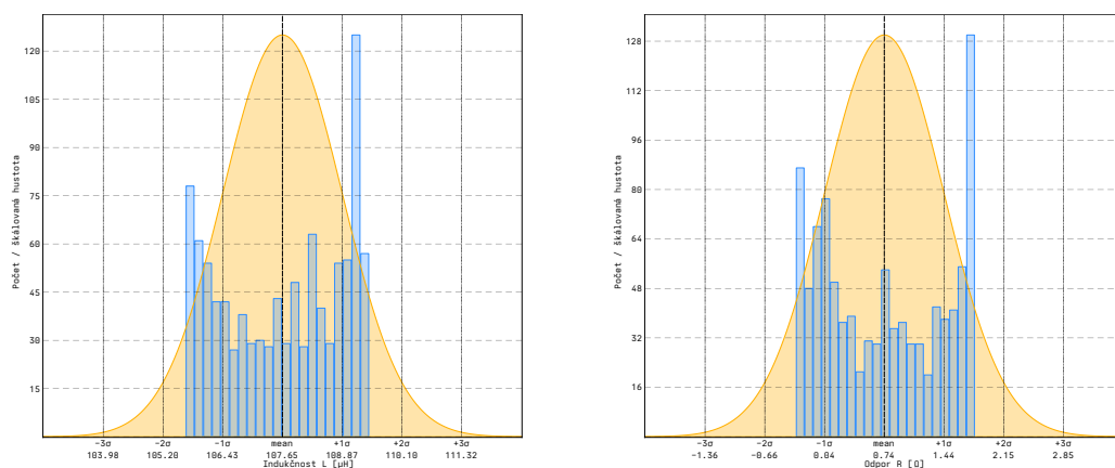
Obr. 7.5: Histogramy hodnot L_{\text{Toroid}} a jeho sériového odporu při 100 kHz
