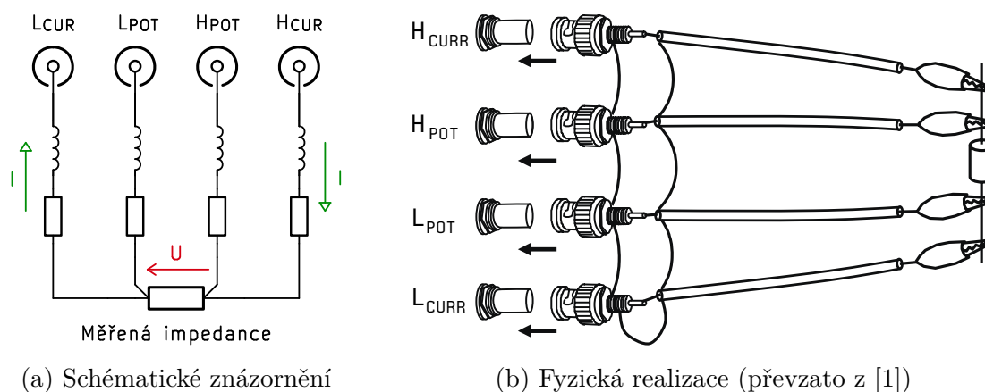
Obr. 4.5: Princip 4-bodového (Kelvinova) připojení měřené impedance.
