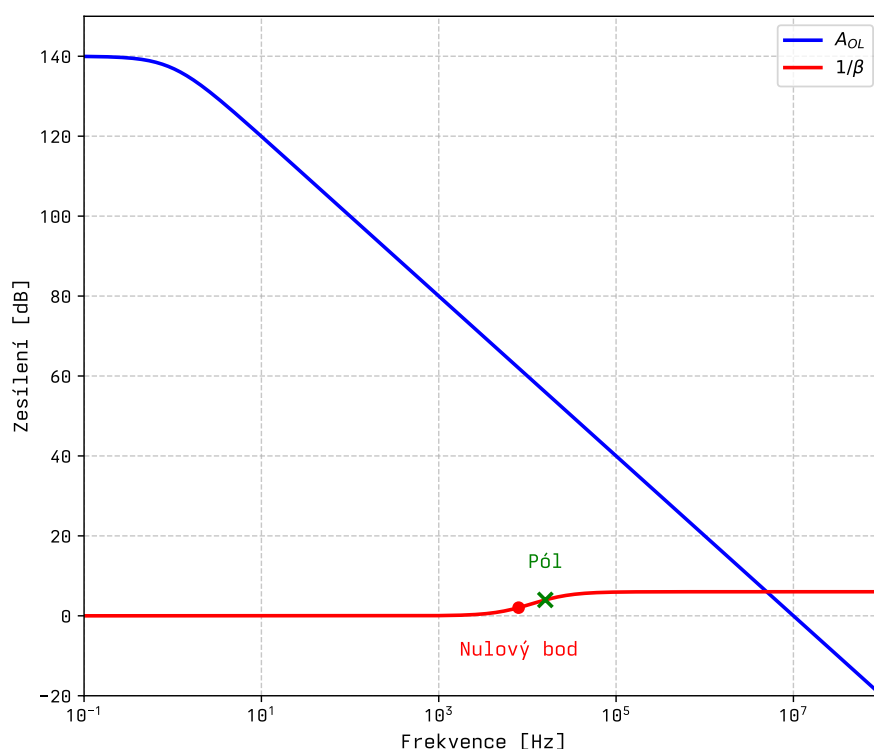
Obr. 2.7: Průběh A_{OL} a 1/\beta pro kompenzované zapojení.
