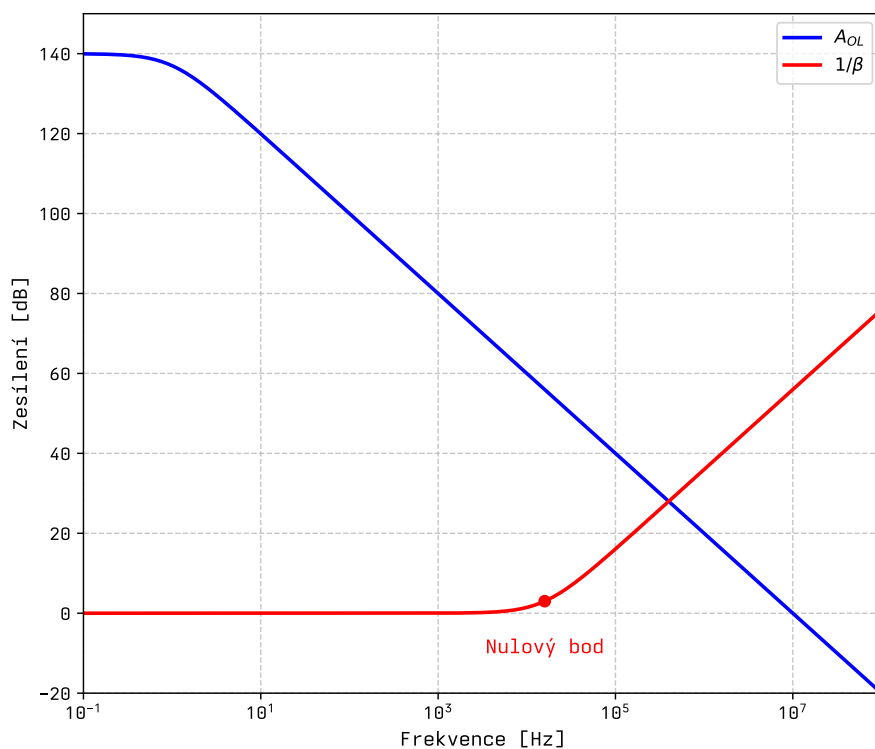
Obr. 2.5: Průběh A_{OL} a 1/\beta pro nekompenzované zapojení.
