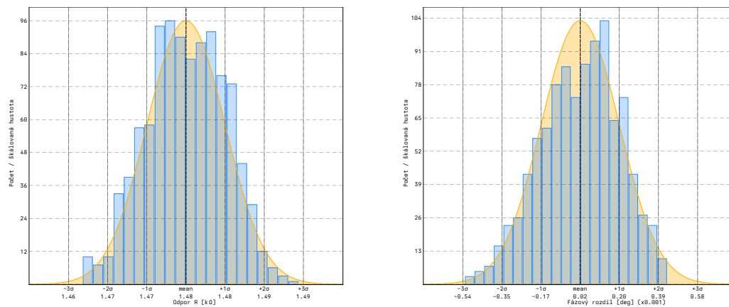
Obr. 8.6: Histogramy hodnot odporu a fázového rozdílu rezistoru při 10 kHz
