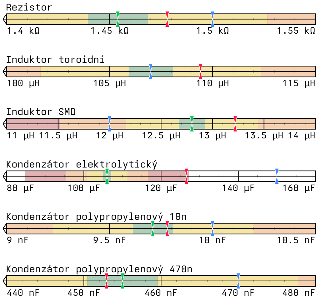
Obr. 8.2: Grafické porovnání hodnot naměřených navrženým LCR metrem a referenčním přístrojem BK Precision 880.
