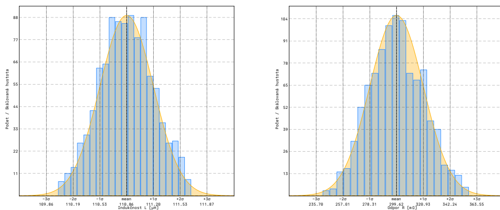
Obr. 8.4: Histogramy hodnot L_{\text{Toroid}} a jeho sériového odporu při 10 kHz
