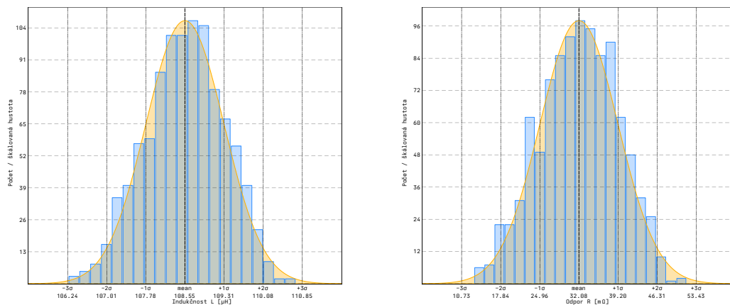
Obr. 8.3: Histogramy hodnot L_{\text{Toroid}} a jeho sériového odporu při 1 kHz
