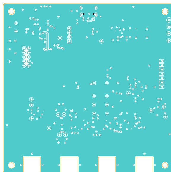
Obr. B.4: Vrstva In3
