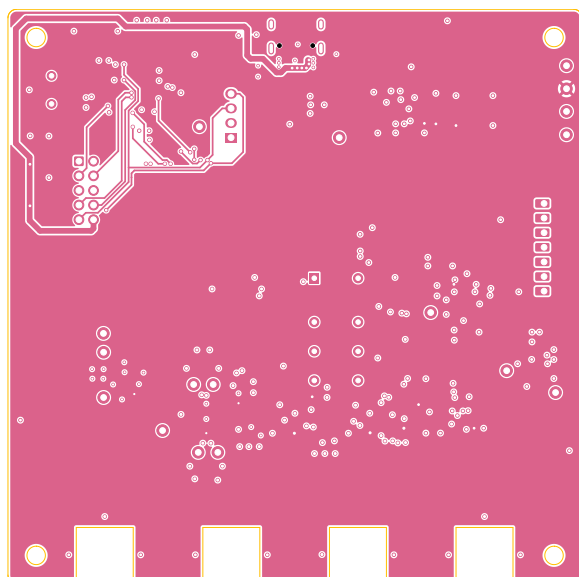
Obr. B.5: Vrstva In4
