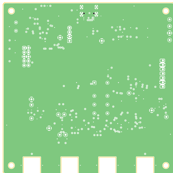
Obr. B.2: Vrstva In1
