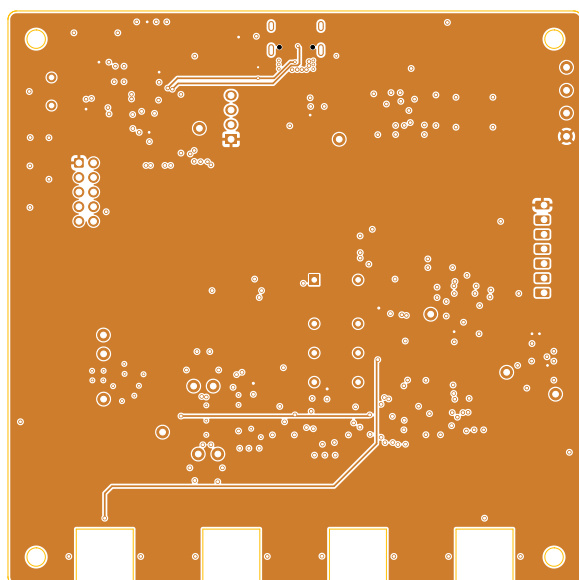
Obr. B.3: Vrstva In2
