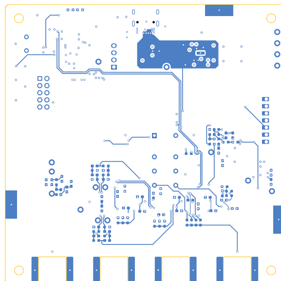
Obr. B.6: Vrstva Bottom
