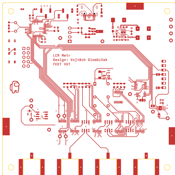
Obr. B.1: Vrstva Top
