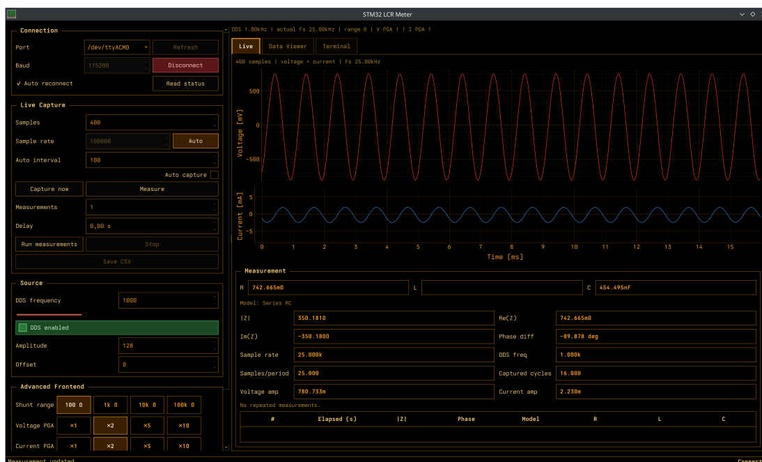
Obr. 6.1: Hlavní okno aplikace při základním měření
