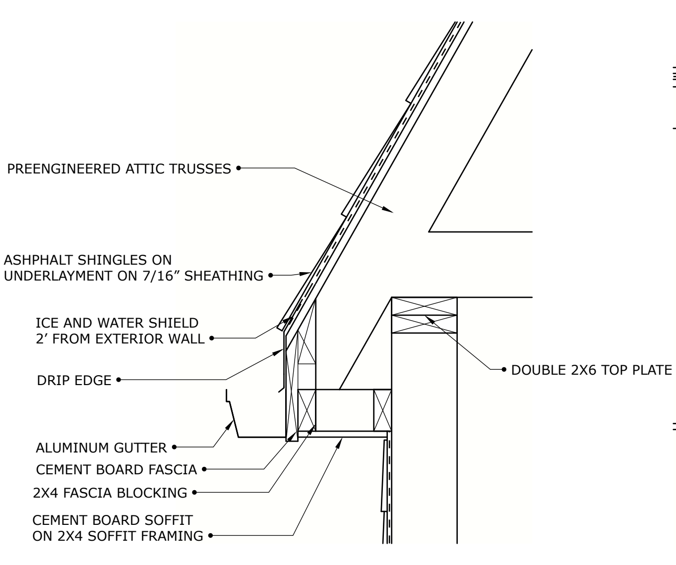
8 GARAGE ROOF EDGE DETAIL A-10 SCALE: 1 1/2" = 1'-0"
