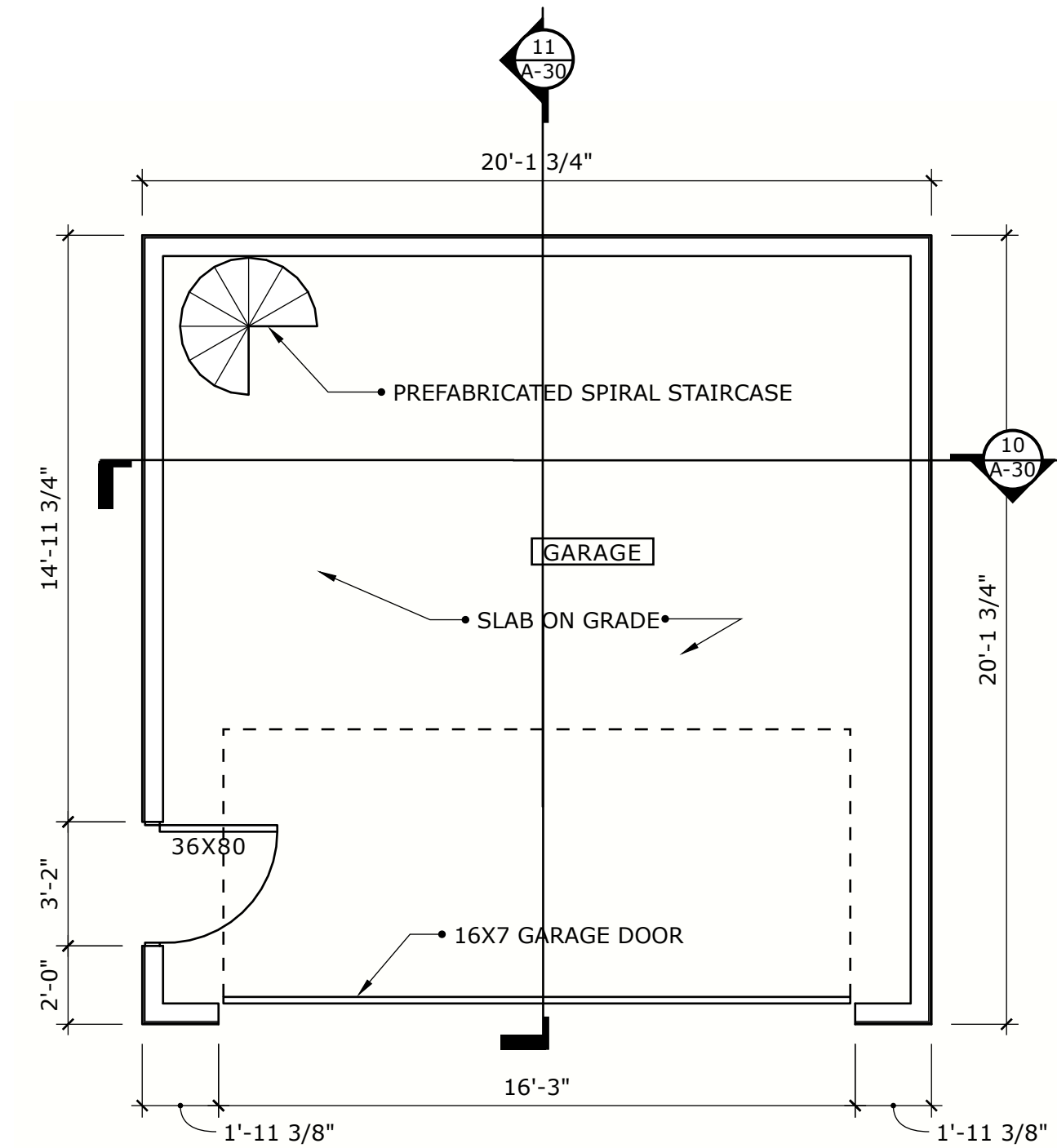
5 GARAGE PLAN A-10 SCALE: 1/4" = 1'-0"
