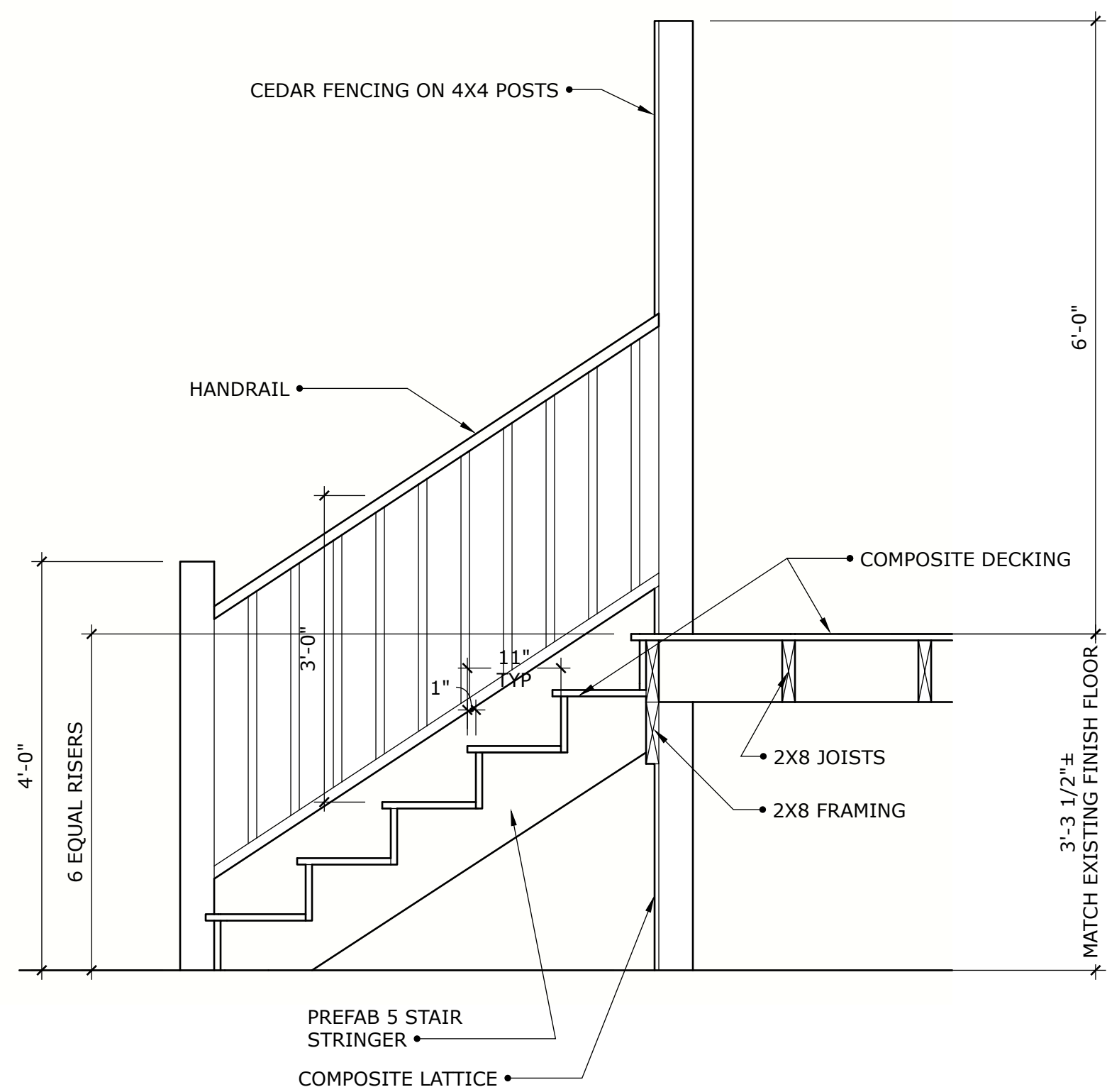
4 DECK STAIR SECTION A-00 SCALE: 3/4" = 1'-0"
