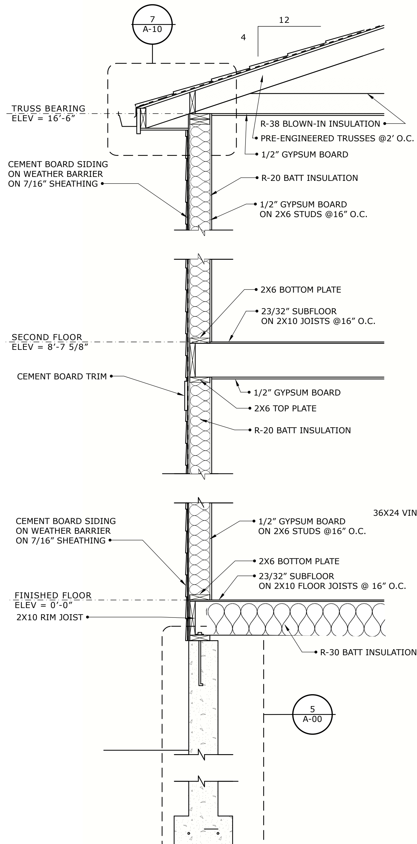
3 WALL SECTION A-10 SCALE: 3/4" = 1'-0"
