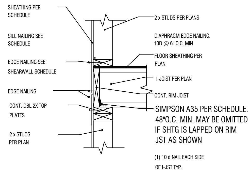
5 PERP. FLR. FRAMING ALT. @ EXT. WALL SCALE: N.T.S.
