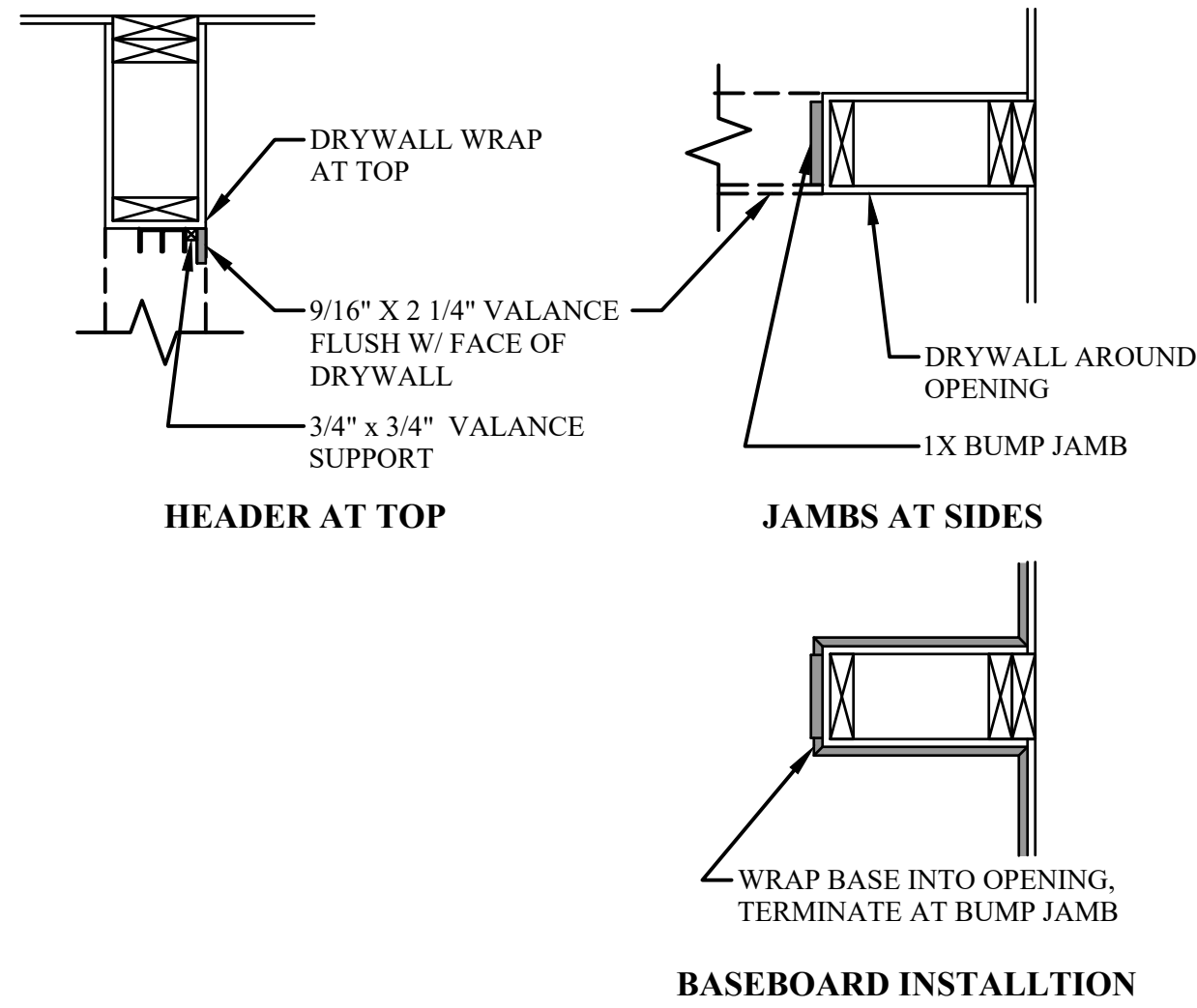
9a BI-PASS CLOSET DOOR STD DRYWALL WRAPPED SCALE: 1" = 1'-0"
