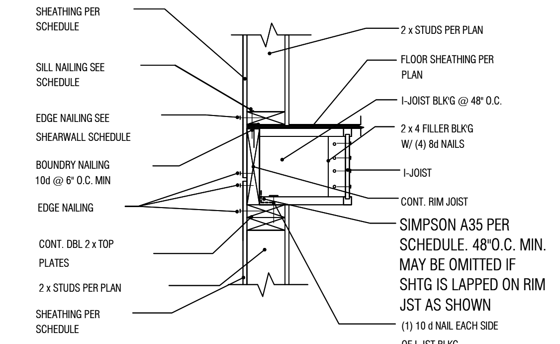
6 PARALLEL FLR. FRAMING ALT. @ EXT. WALL SCALE: N.T.S.
