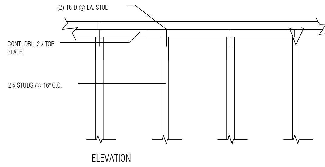
7 TOP PLATE SPLICE SCALE: N.T.S.
