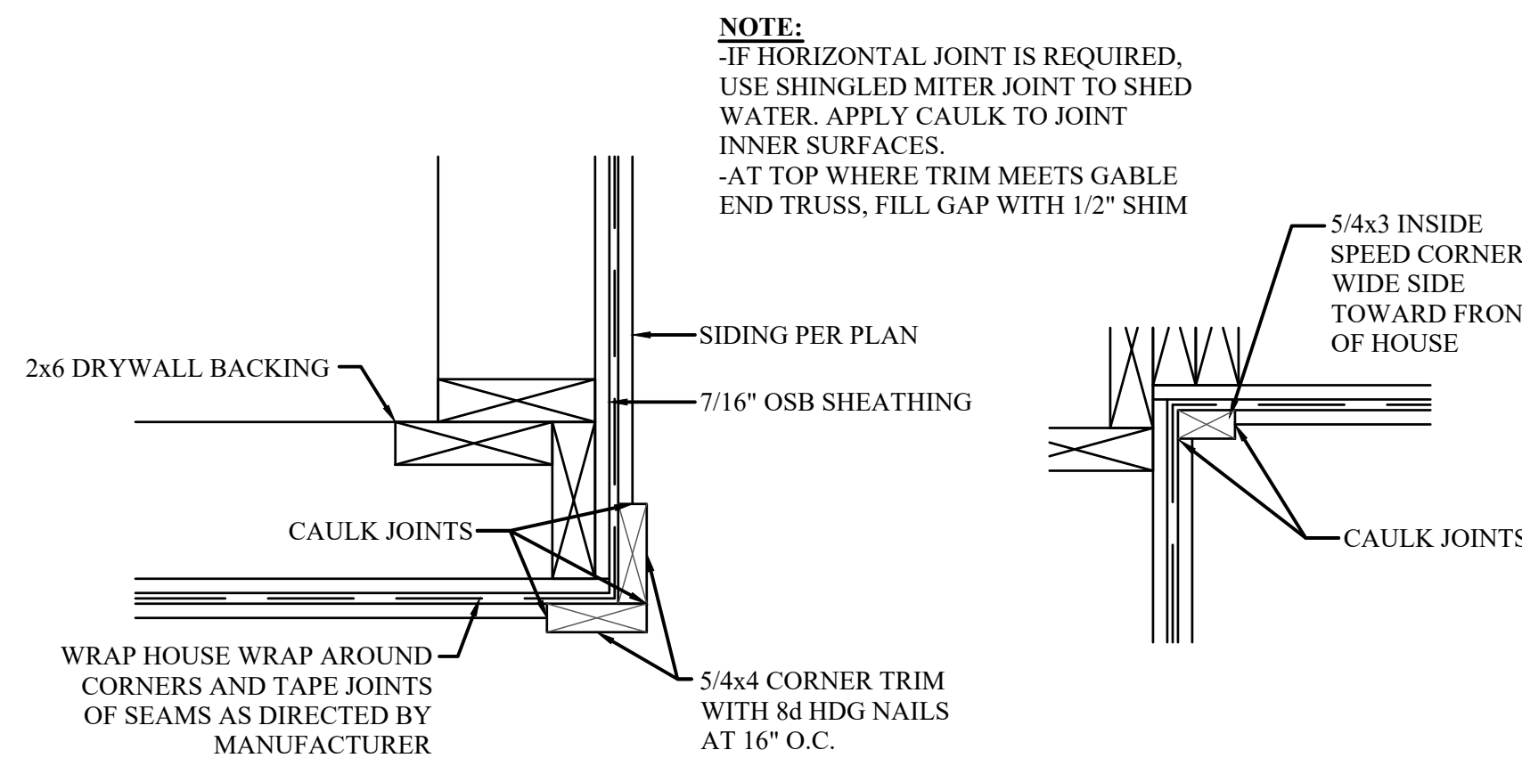
5 CORNERBOARD TRIM SCALE: 2\"/>
