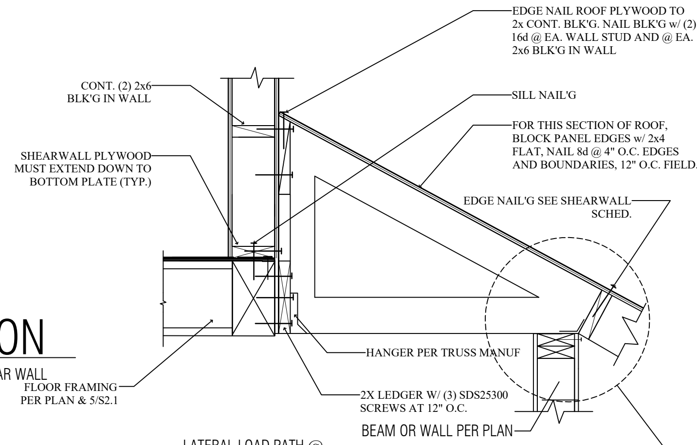
4 ROOF LEDGER SCALE: N.T.S.
