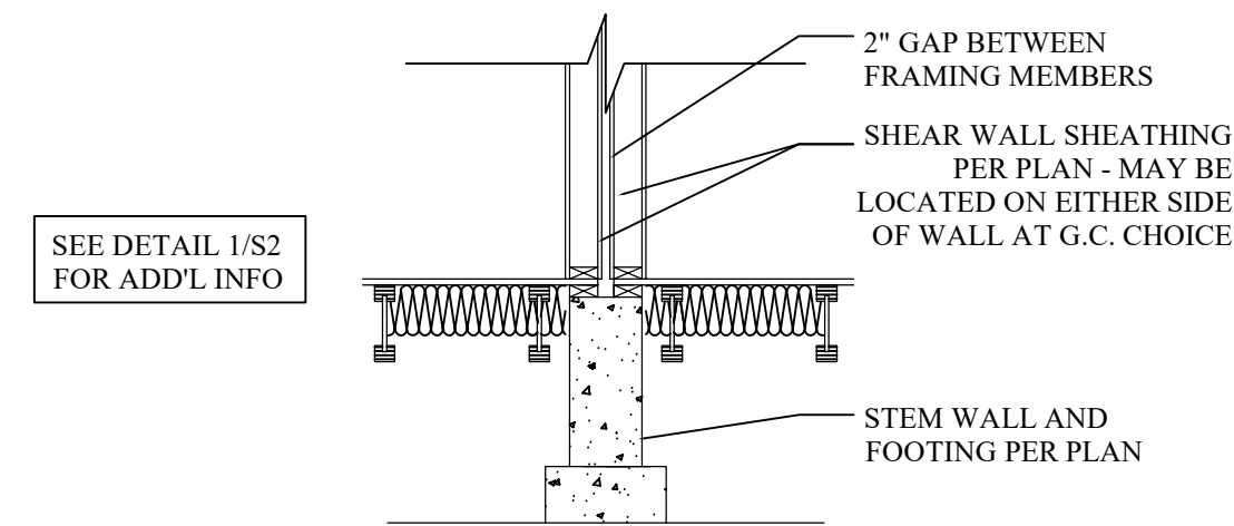
8 FOUNDATION AT PARTY WALL SCALE: N.T.S.
