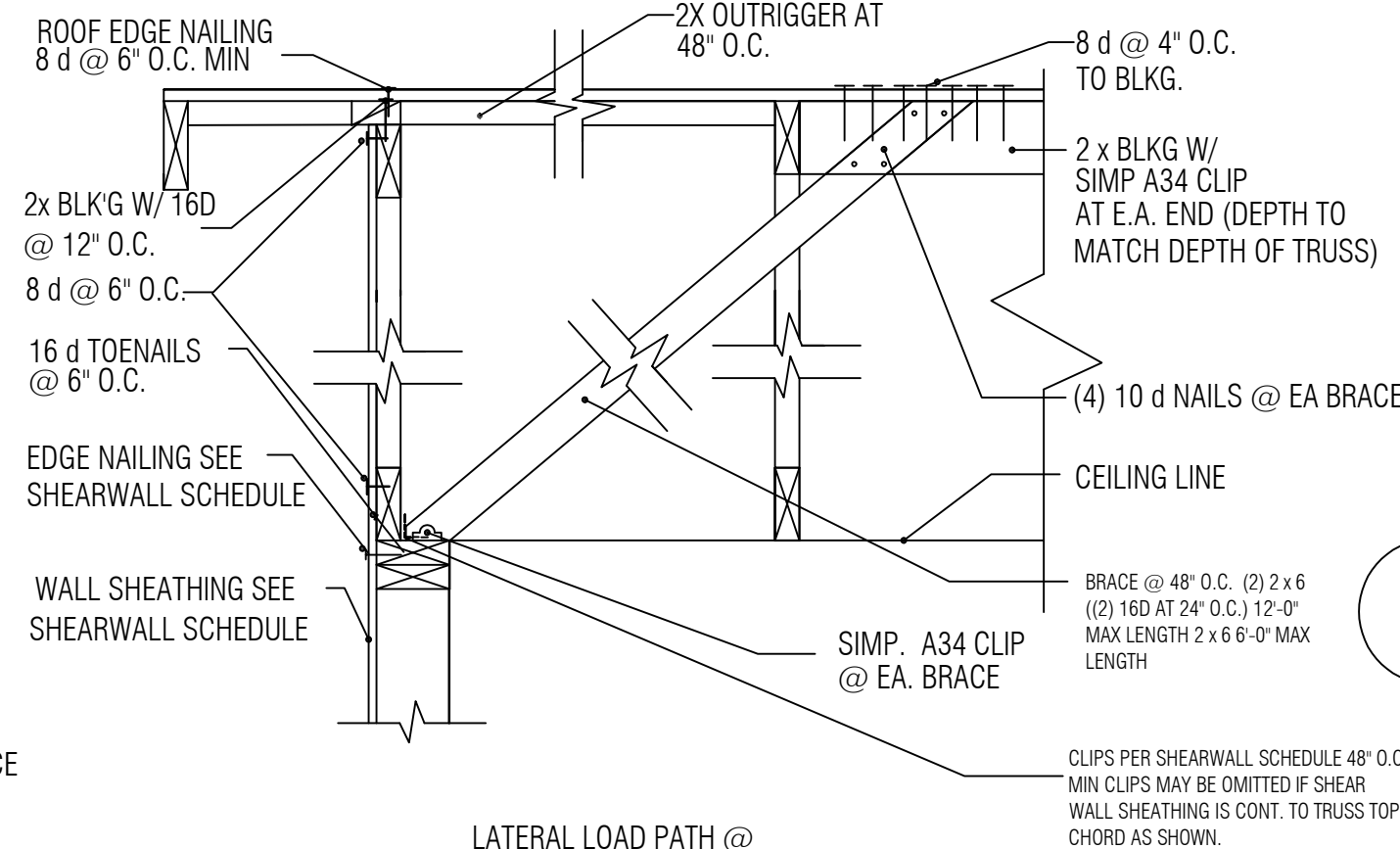
2 PARALLEL TRUSSES TO WALL SCALE: N.T.S.
