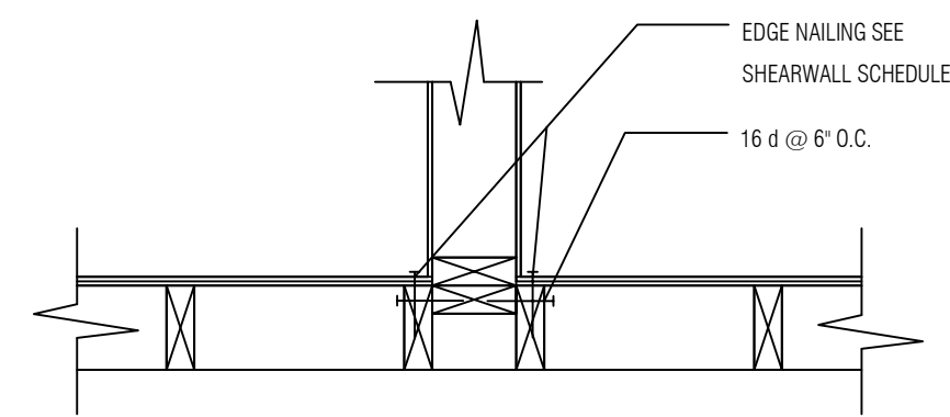
3 THRU WALL INTERRUPTION SCALE: N.T.S.
