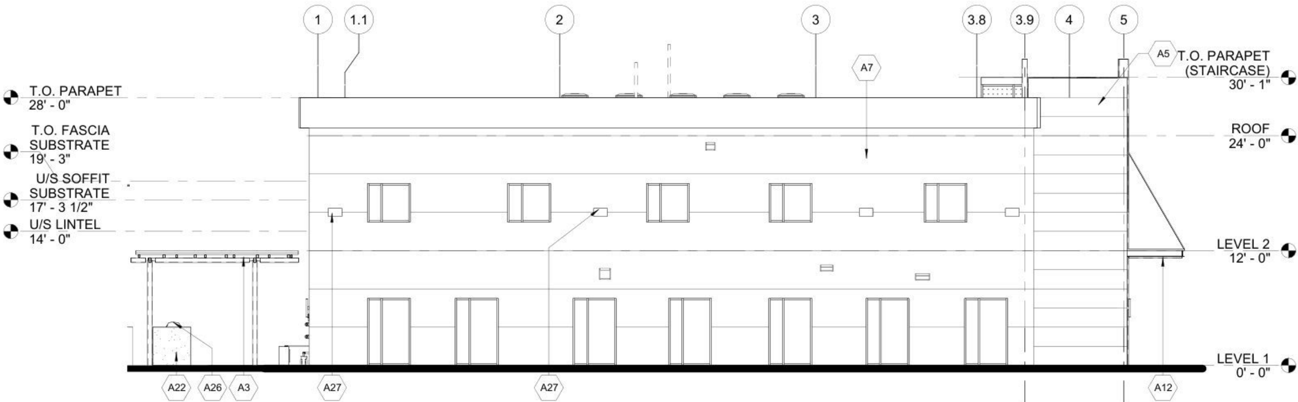
C1 WEST ELEVATION SCALE: 1/8" = 1'-0"
