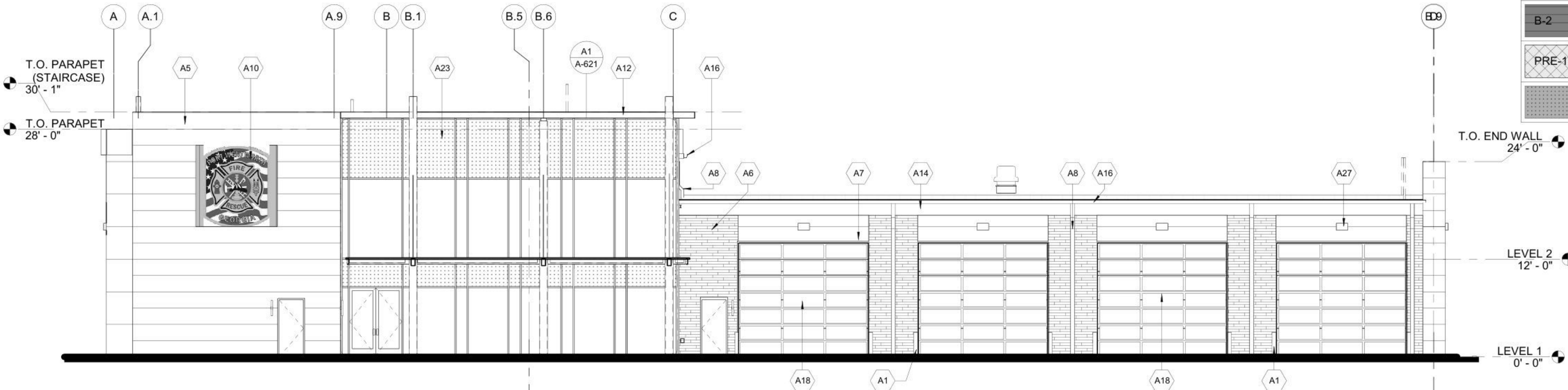
A1 SOUTH ELEVATION SCALE: 1/8" = 1'-0"
