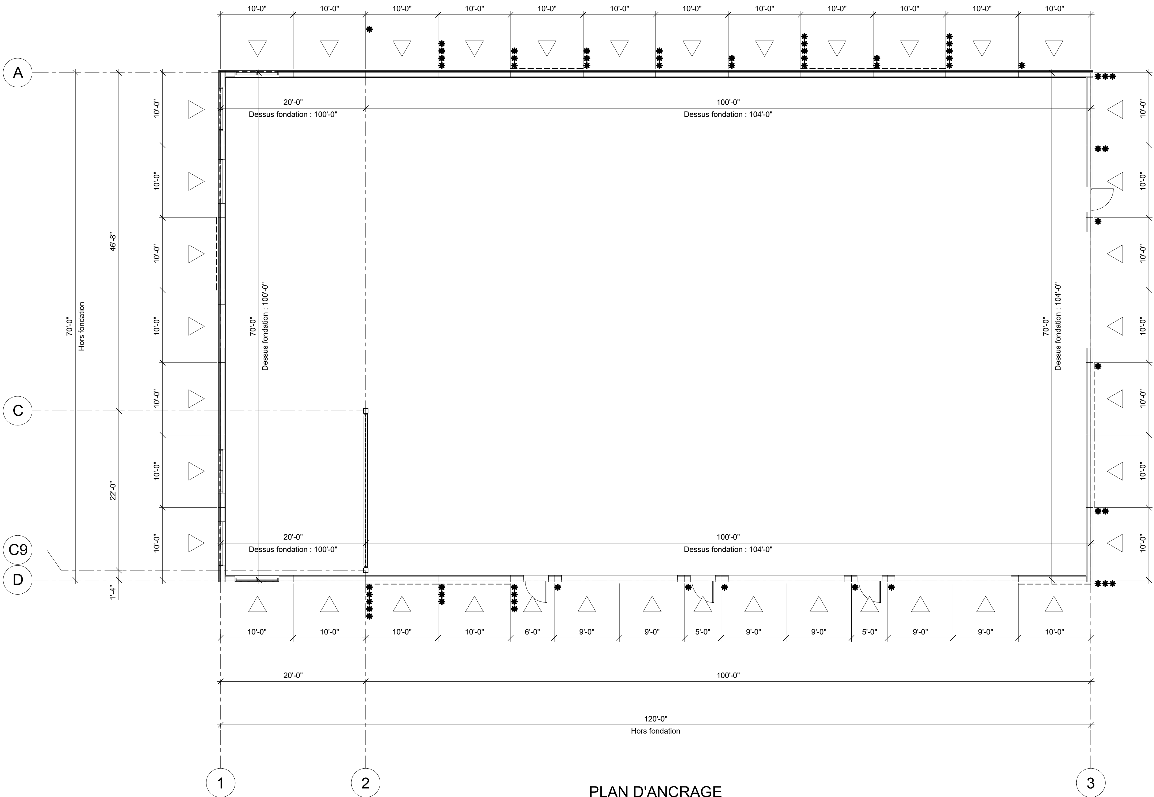
PLAN D'ANCRAGE
