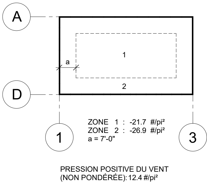
DIAGRAMME DE SOULEVEMENT BRUT (NON PONDÉRÉ)
