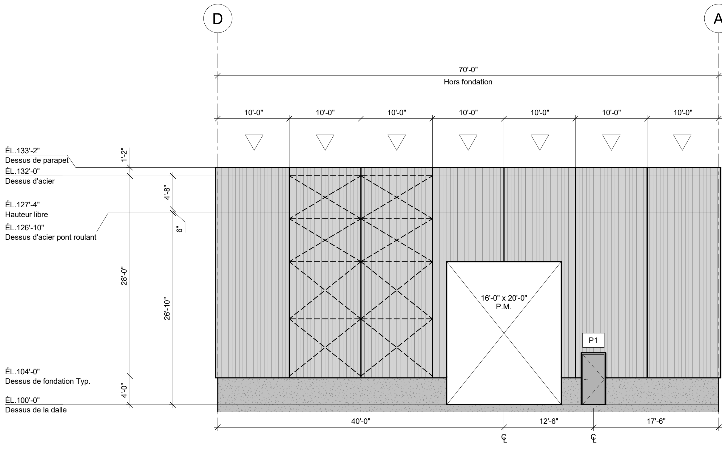
ÉLEVATION AXE 3 (EST) 1/8" = 1'-0"
