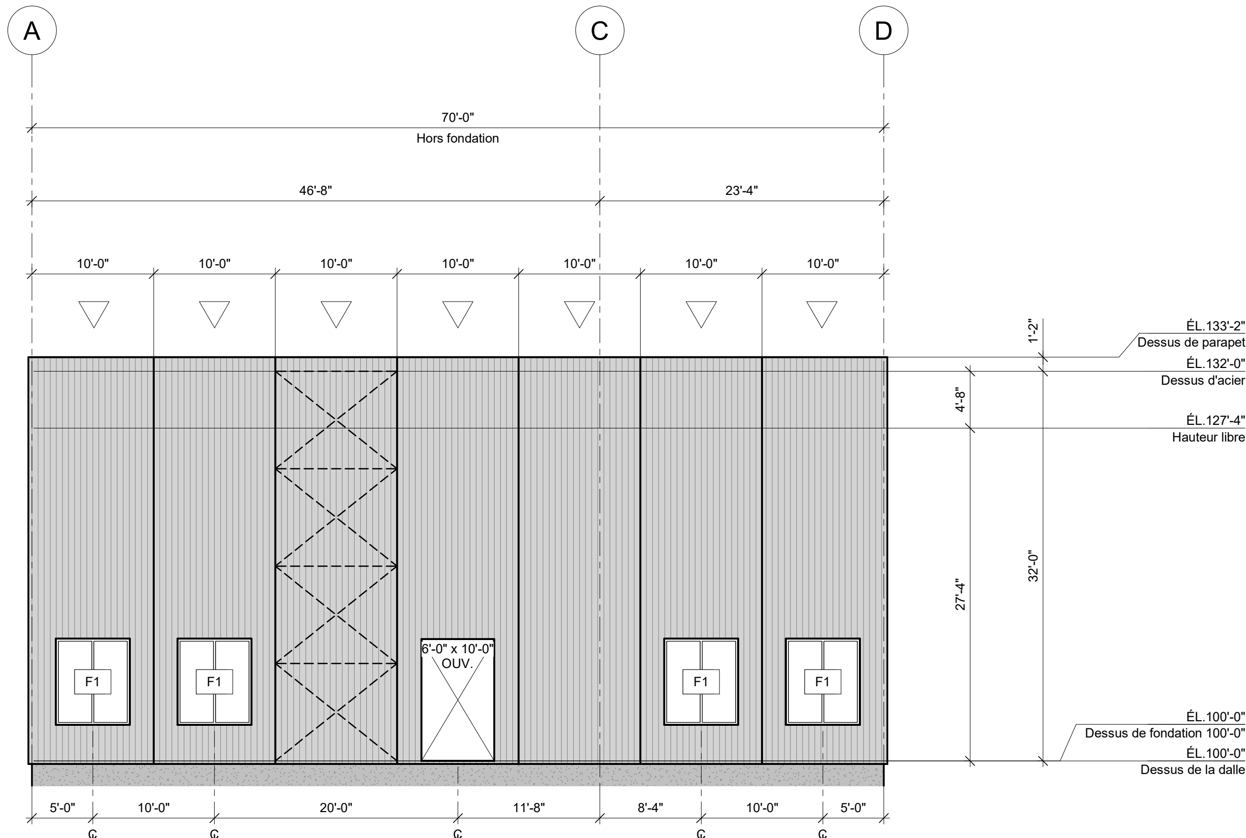
ÉLEVATION AXE 1 (OUEST) 1/8" = 1'-0"
