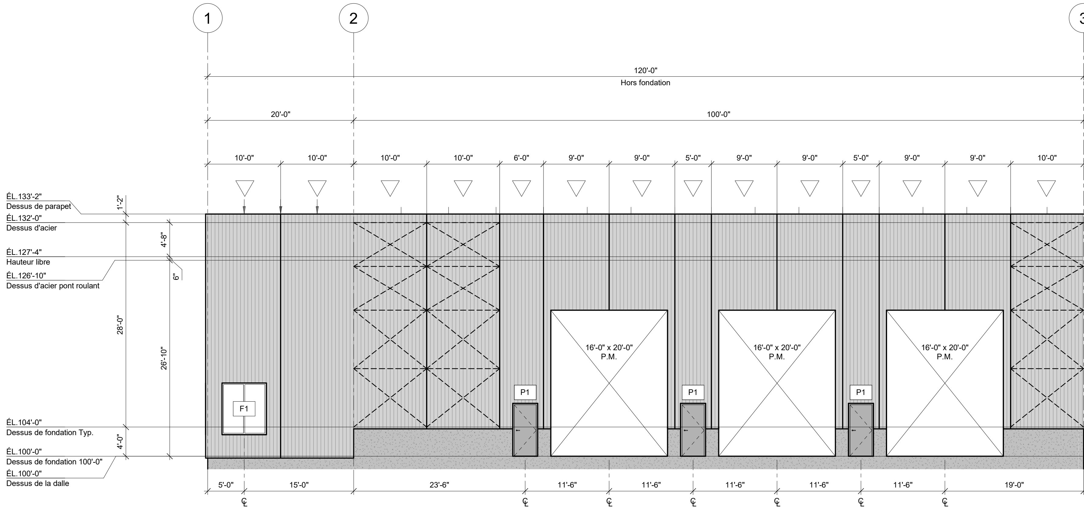
ÉLEVATION AXE D (SUD) 1/8" = 1'-0"
