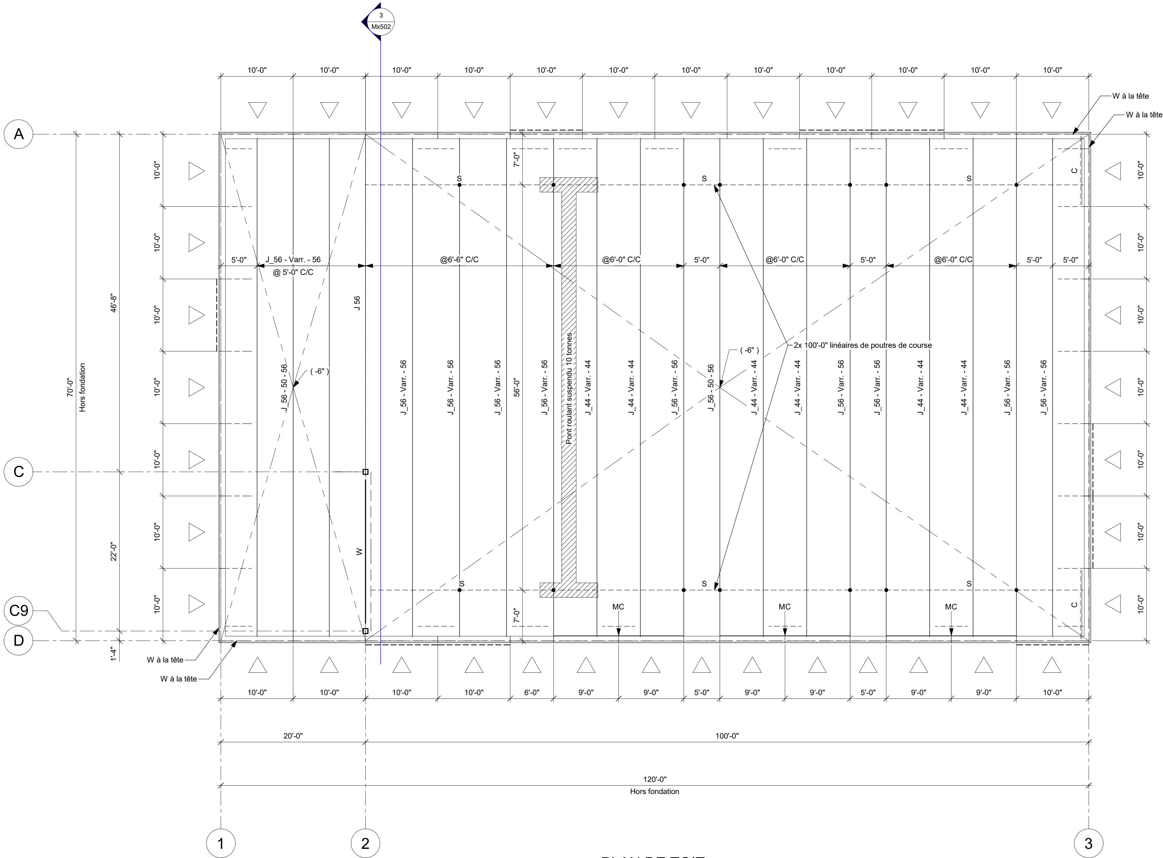
PLAN DE TOIT 1/8" = 1'-0"
