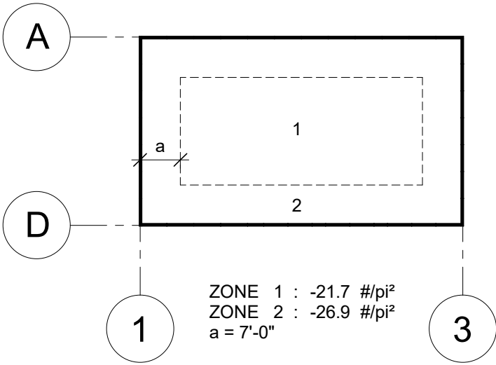
DIAGRAMME DE SOULÈVEMENT BRUT (NON PONDÉRÉ)
