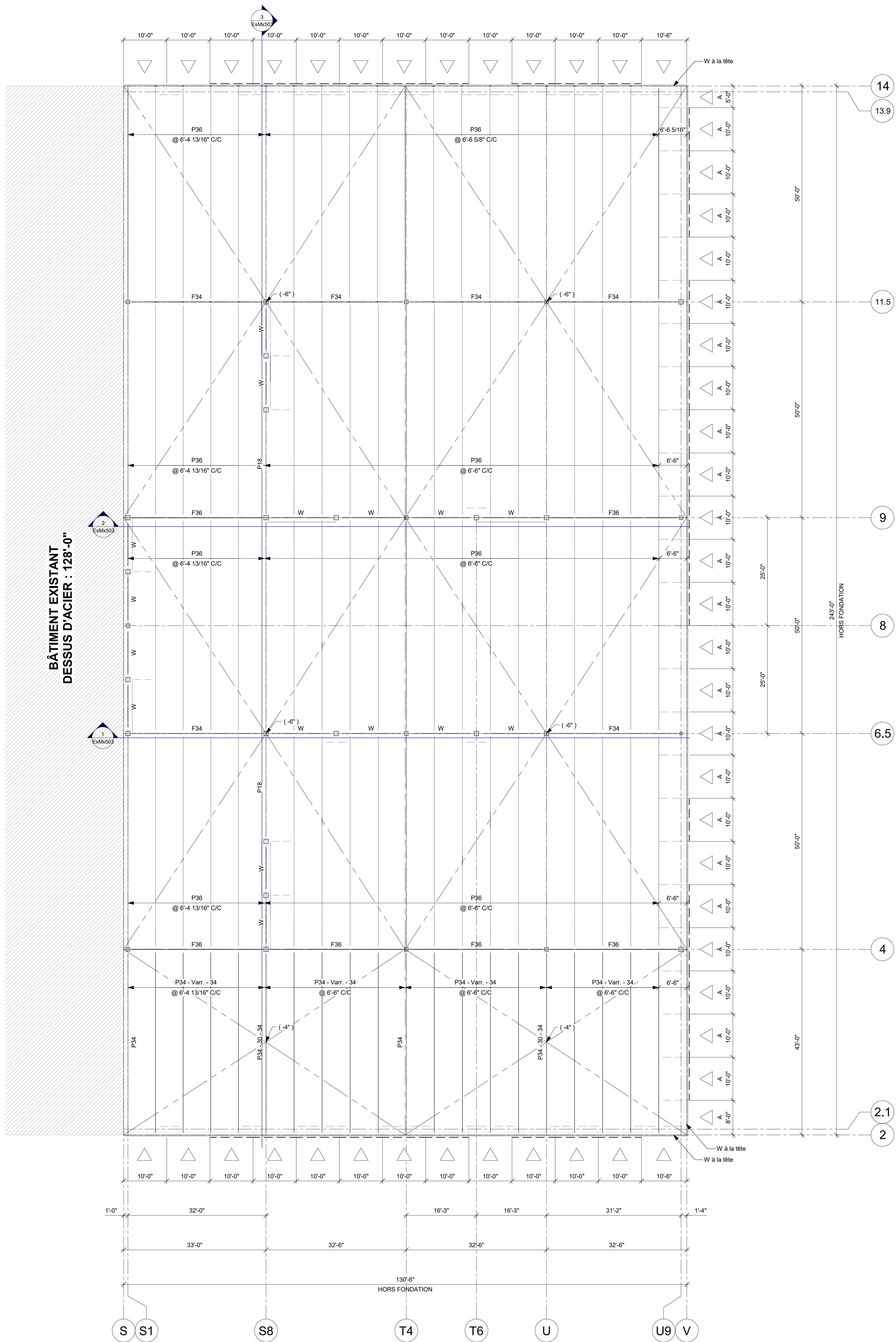
PLAN DE TOIT 3/32" = 1'-0"
