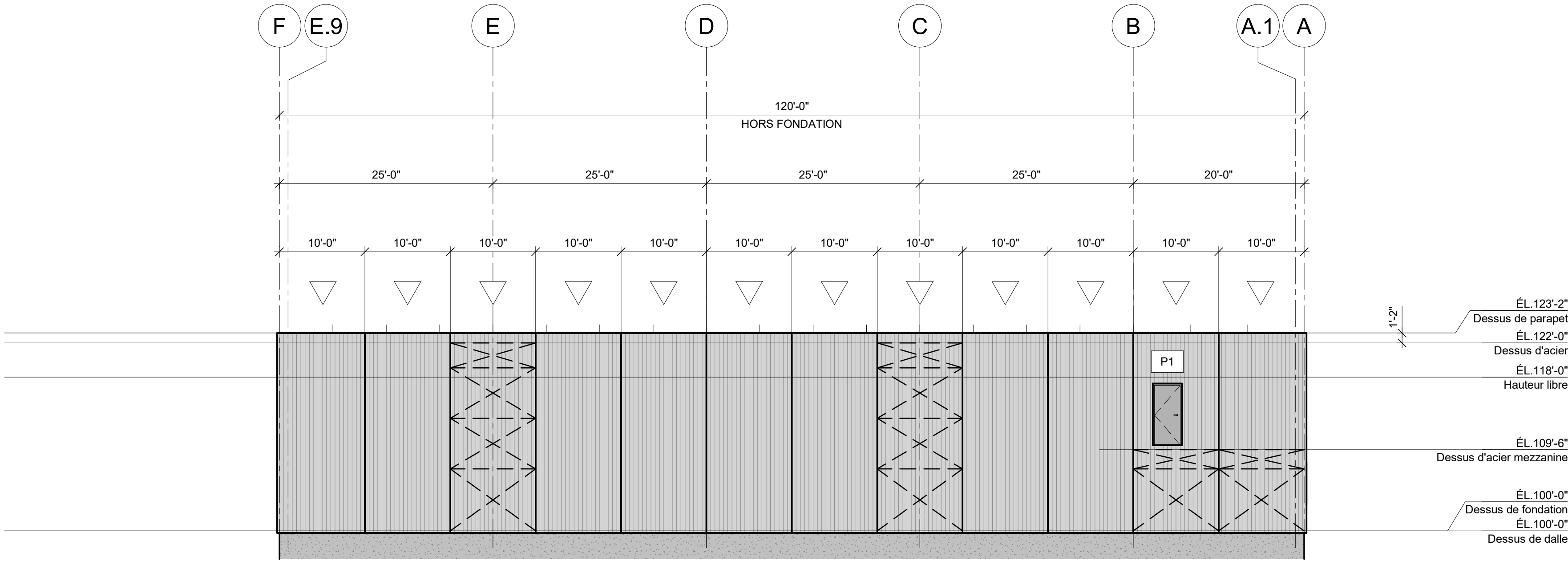
ÉLÉVATION AXE 1 (OUEST) 1" = 10'-0"
