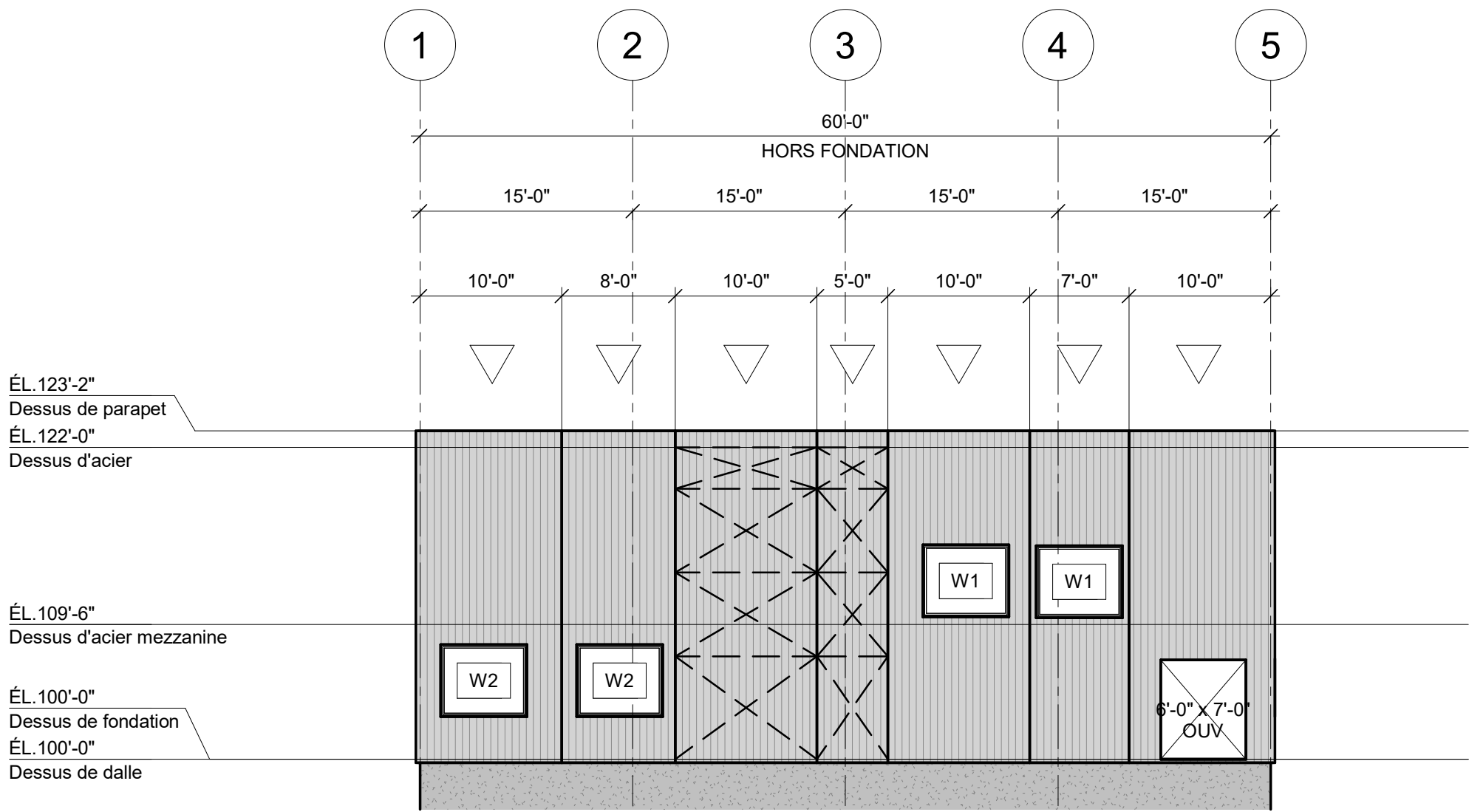
ÉLÉVATION AXE A (SUD) 1" = 10'-0"
