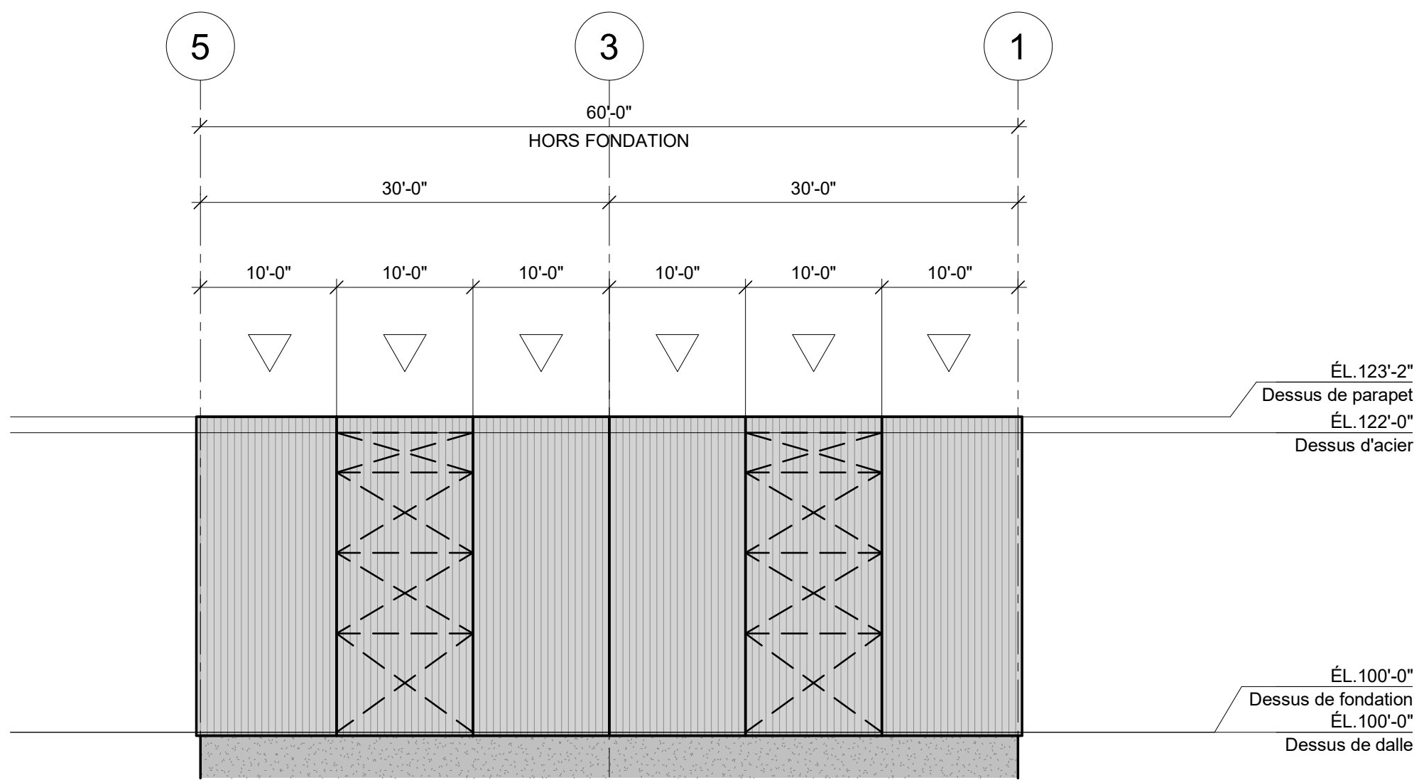
ÉLÉVATION AXE F (NORD) 1" = 10'-0"
