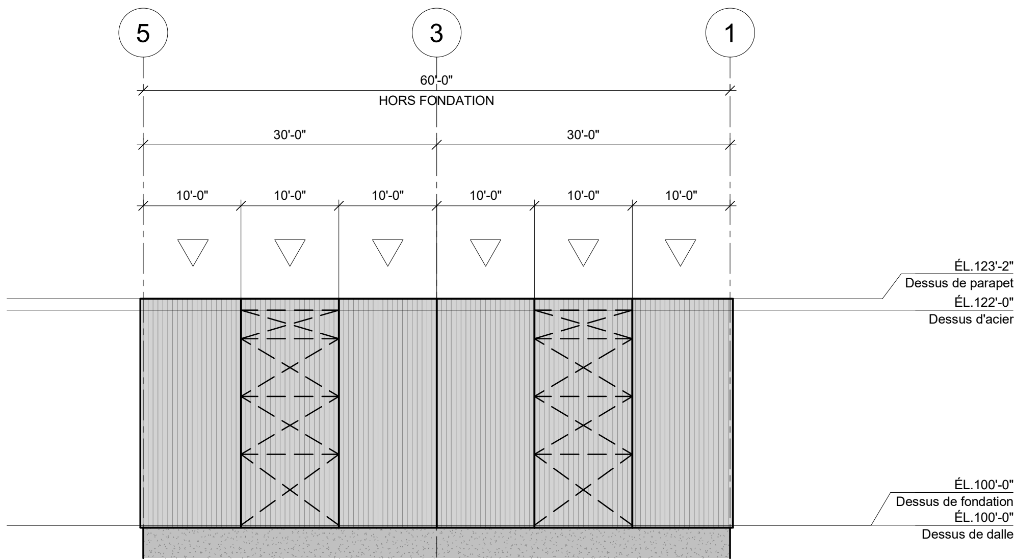
ÉLEVATION AXE F (NORD) 1" = 10'-0"
