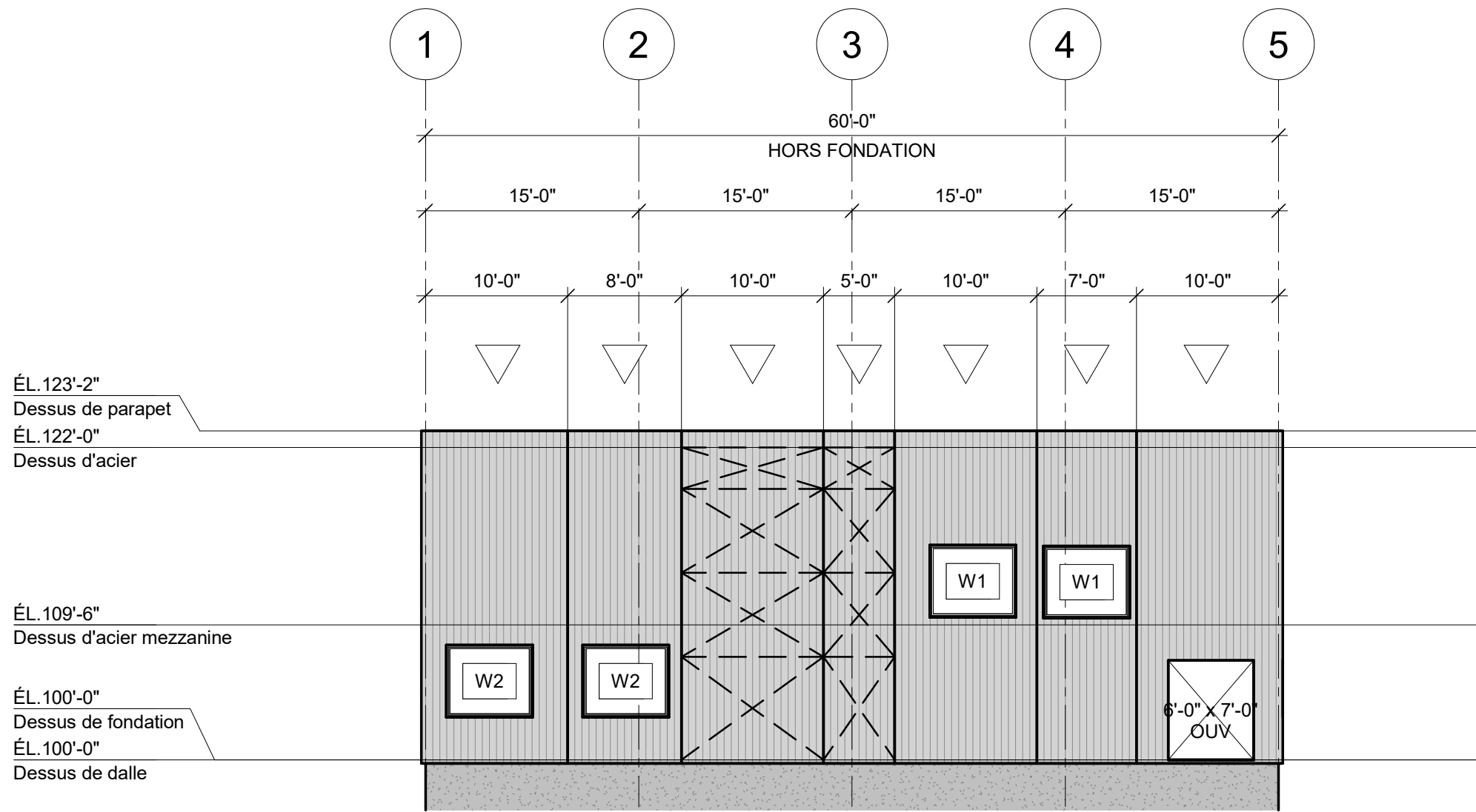
ÉLEVATION AXE A (SUD) 1" = 10'-0"
