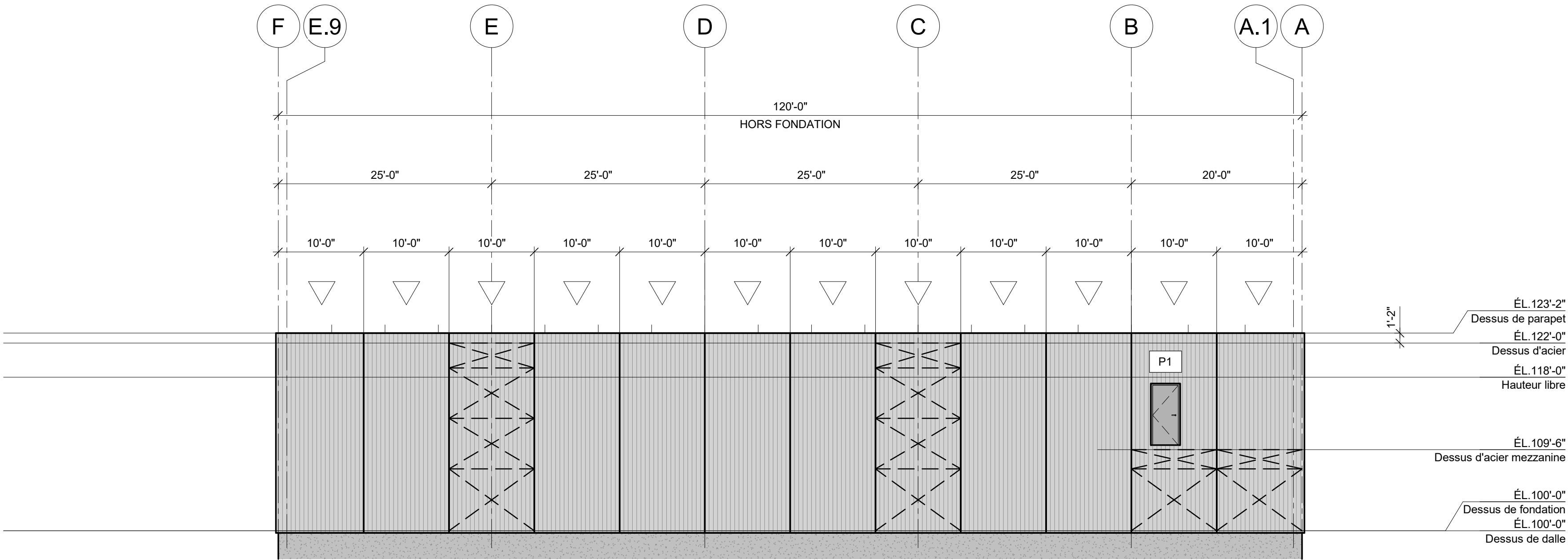
ÉLEVATION AXE 1 (OUEST) 1" = 10'-0"
