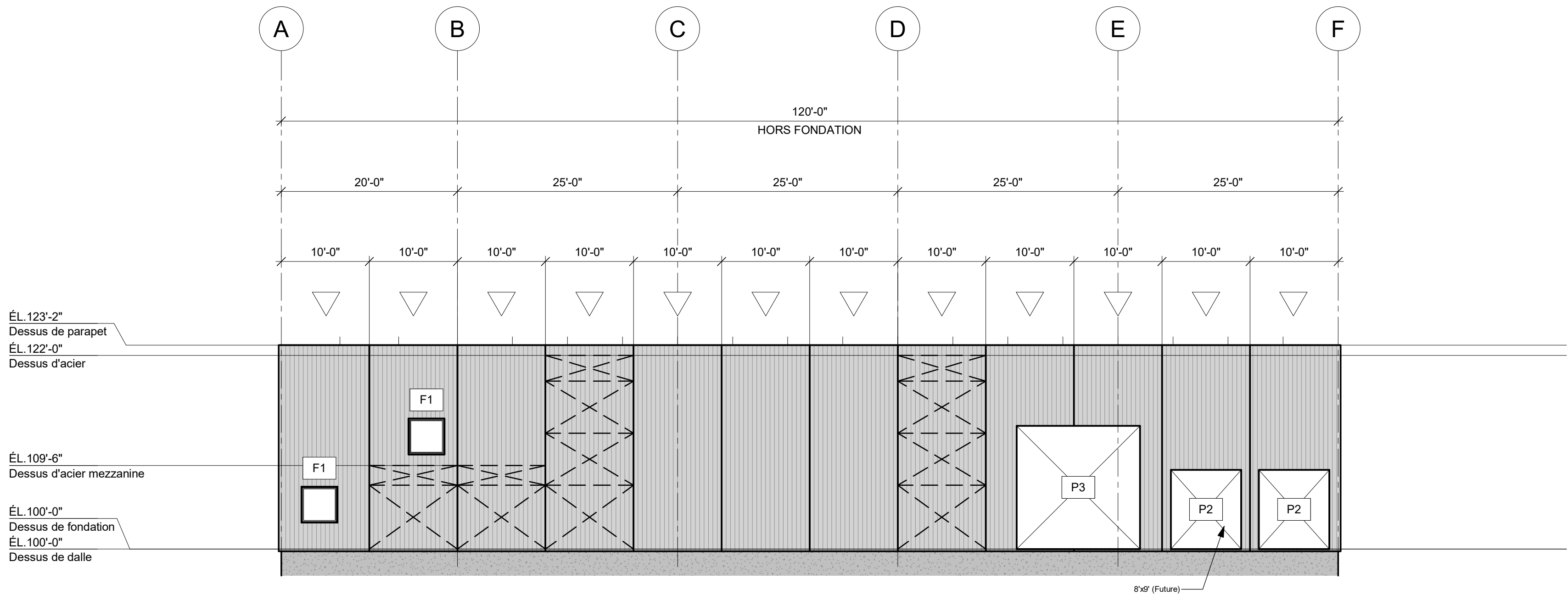
ÉLÉVATION AXE 5 (EST) 1" = 10'-0"
