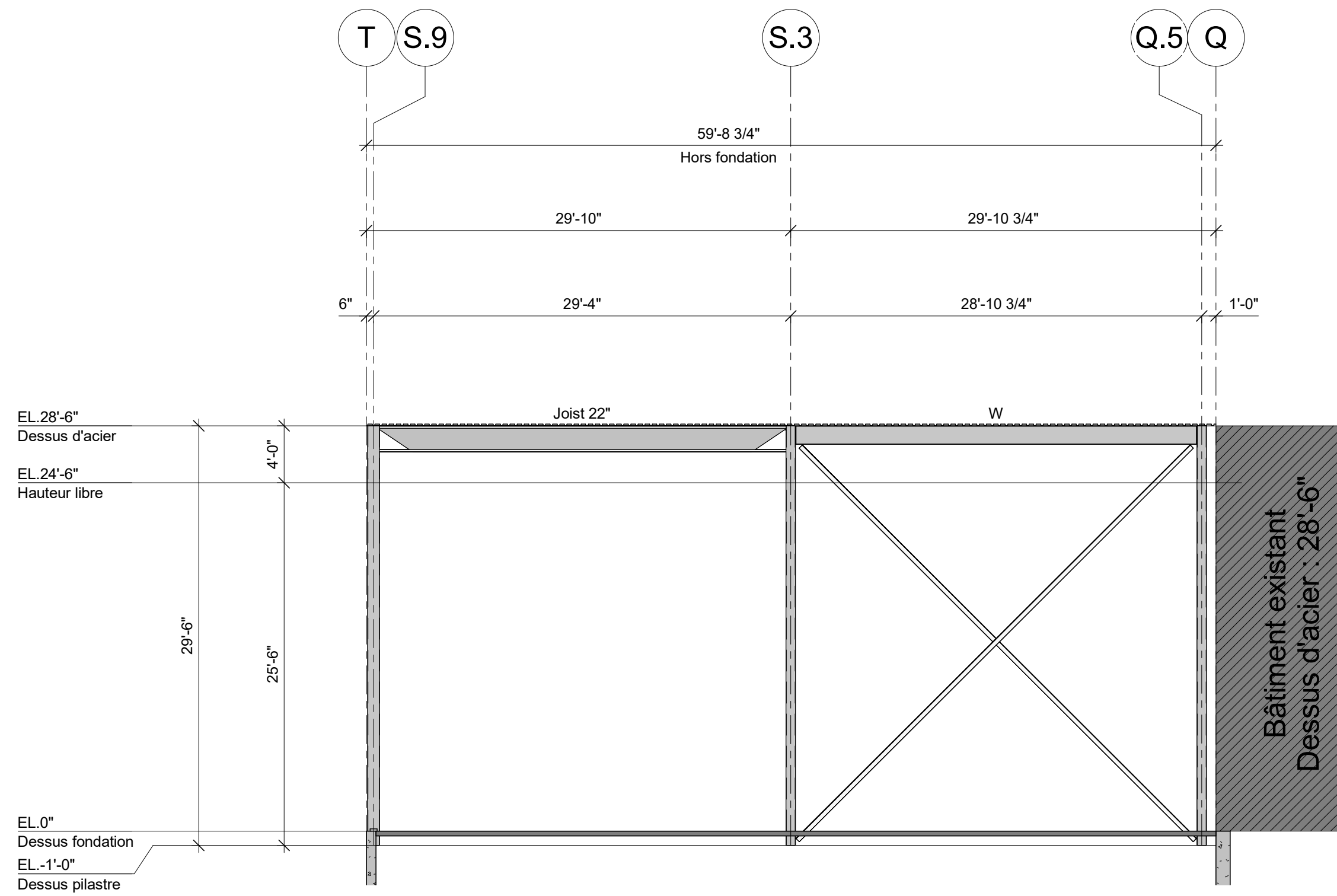
ELEVATION AXE 31.3 (OUEST) 1/8" = 1'-0"
