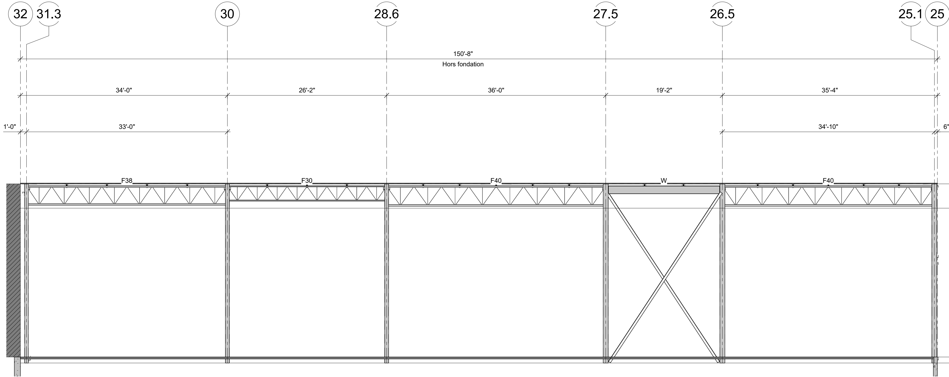
ELEVATION AXE Q.5 (SUD)
