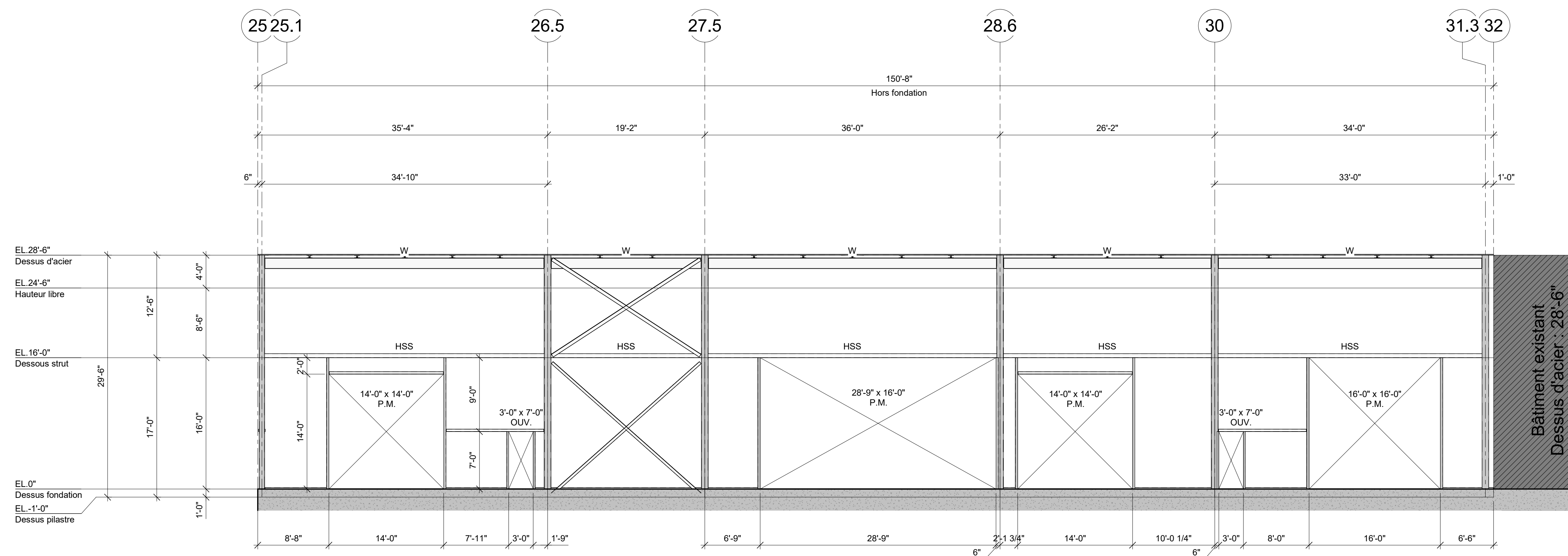
ELEVATION AXE T (NORD)
