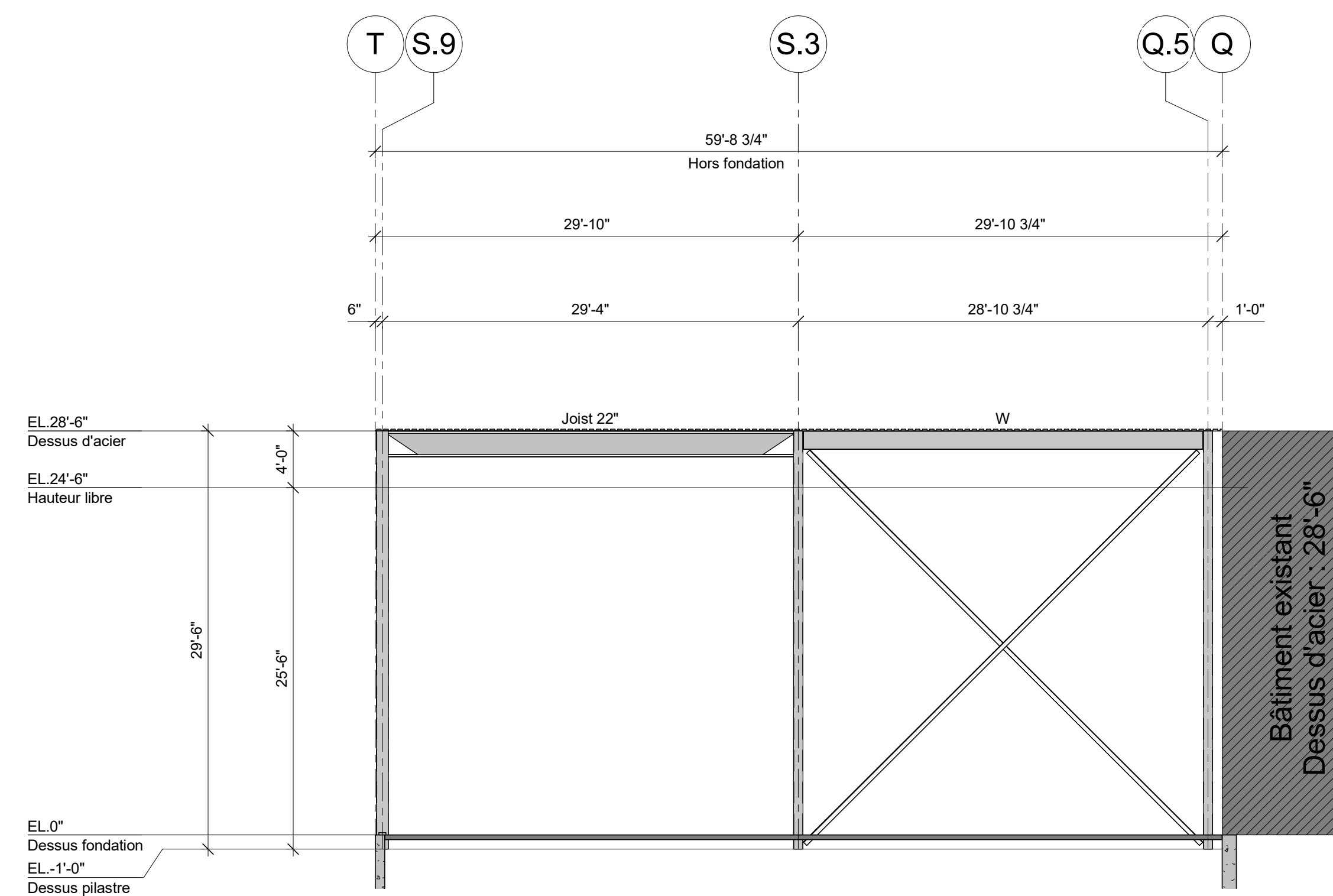
ELEVATION AXE 31.3 (OUEST)
