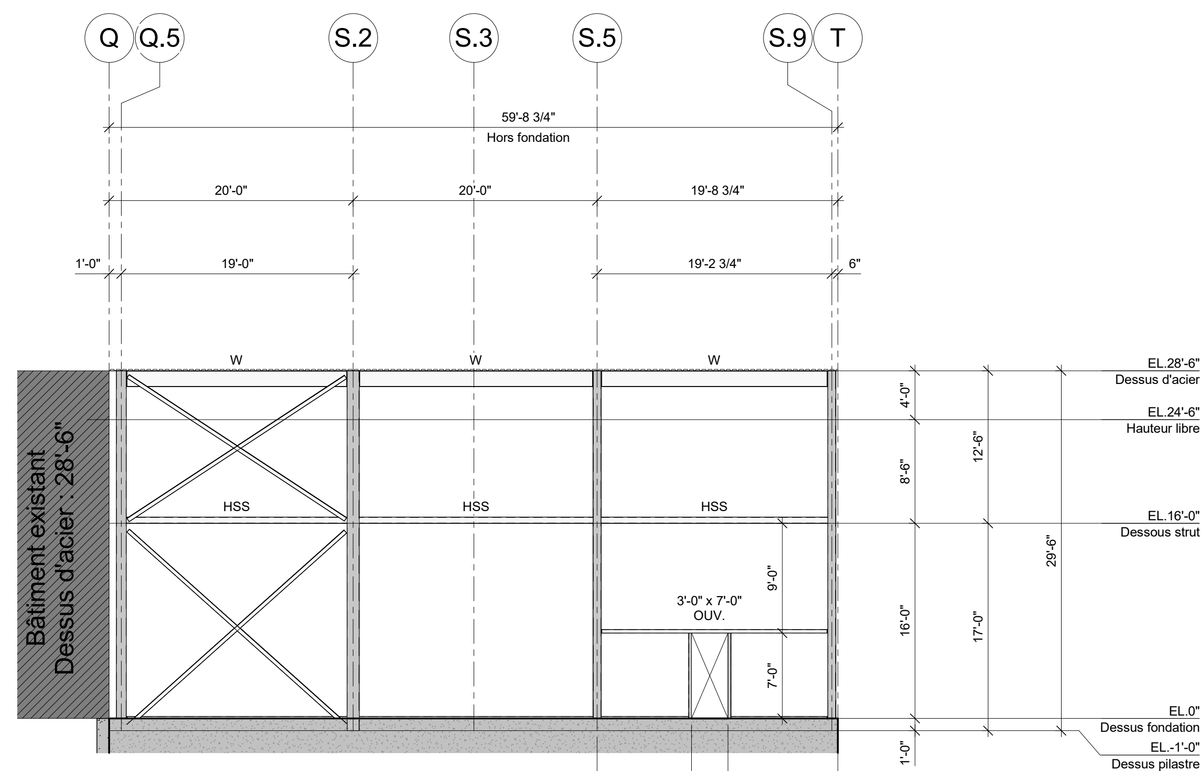
ELEVATION AXE 25 (EST)
