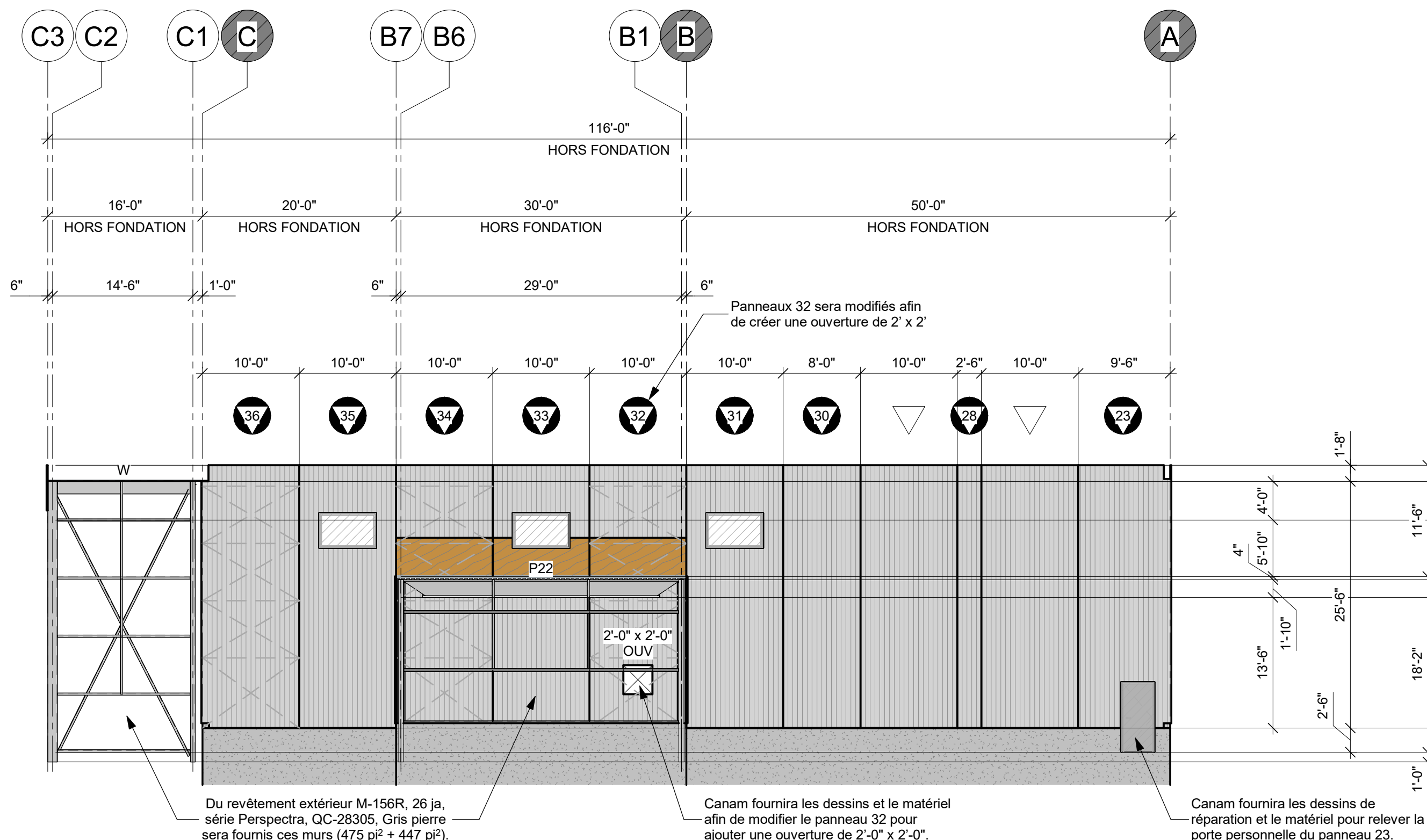
ÉLÉVATION AXE 2' & 1' (NORD) 3/32" = 1'-0"
