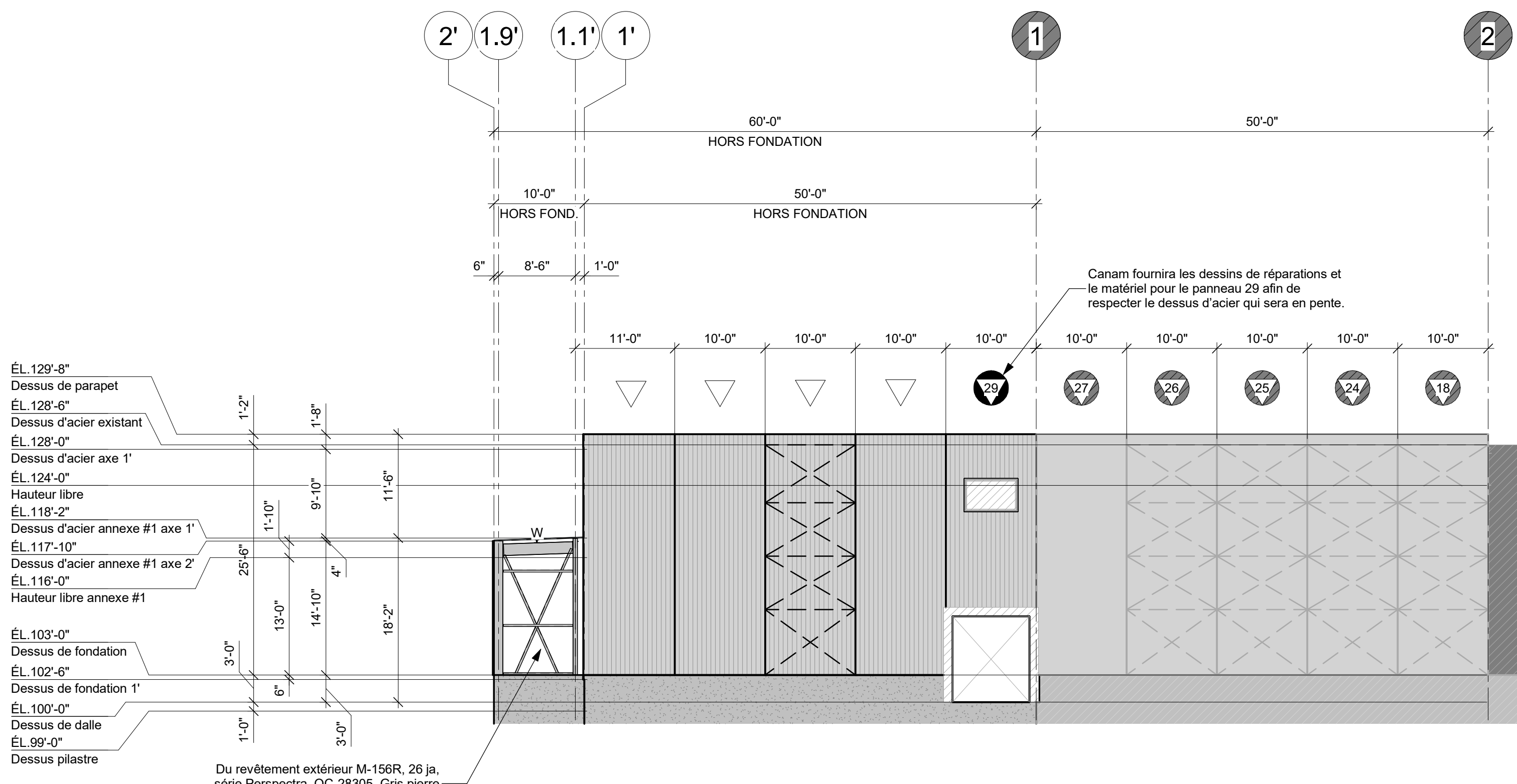
ÉLÉVATION AXE B & A (OUEST) 3/32" = 1'-0"
