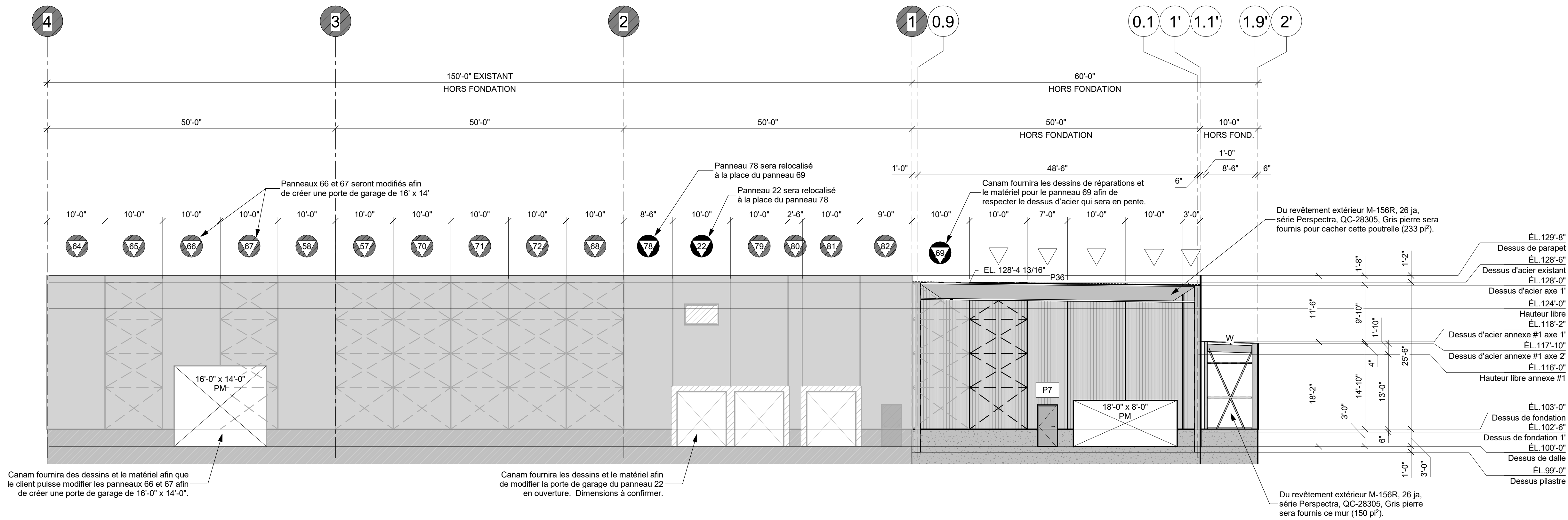
ÉLÉVATION AXE F, C & B7 (EST) 3/32" = 1'-0"
