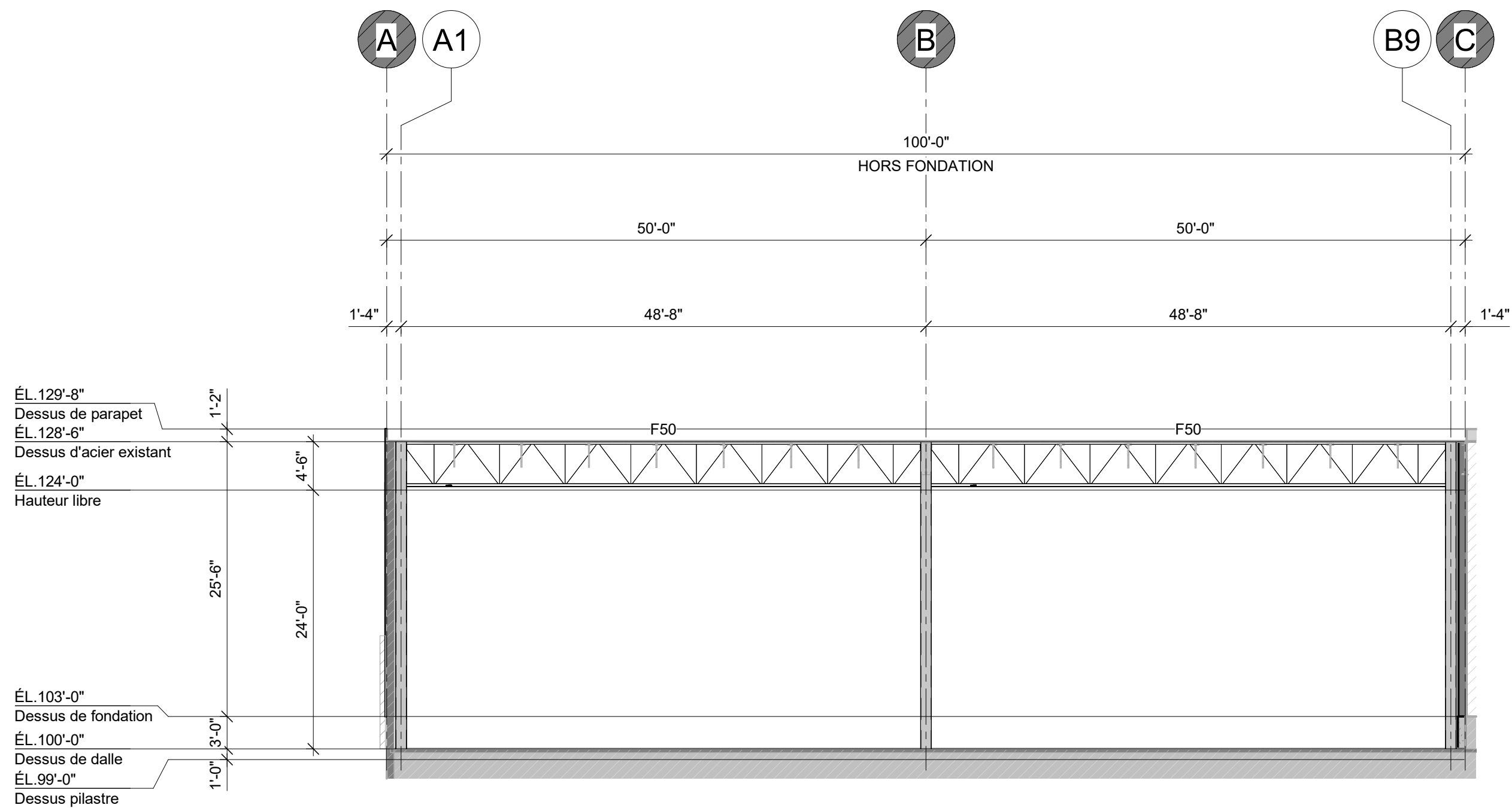
2 COUPE AXE 1 (SUD) 3/32" = 1'-0"
