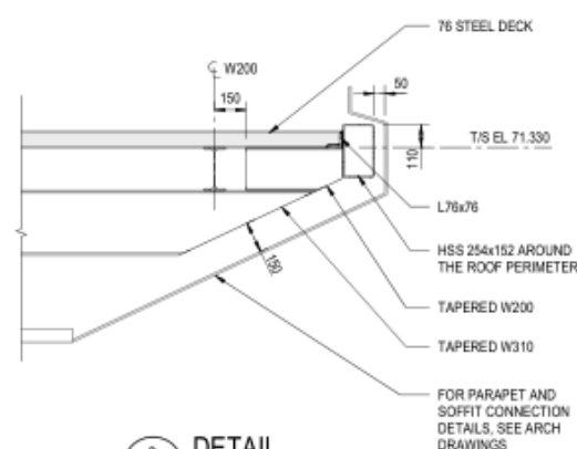
3 1230 DETAIL 1 : 20
