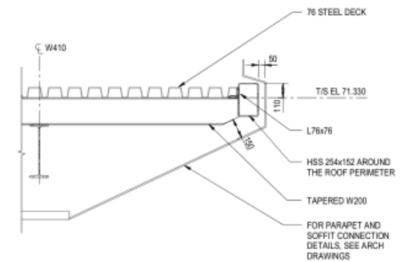
5 DETAIL 1230 1 : 20
