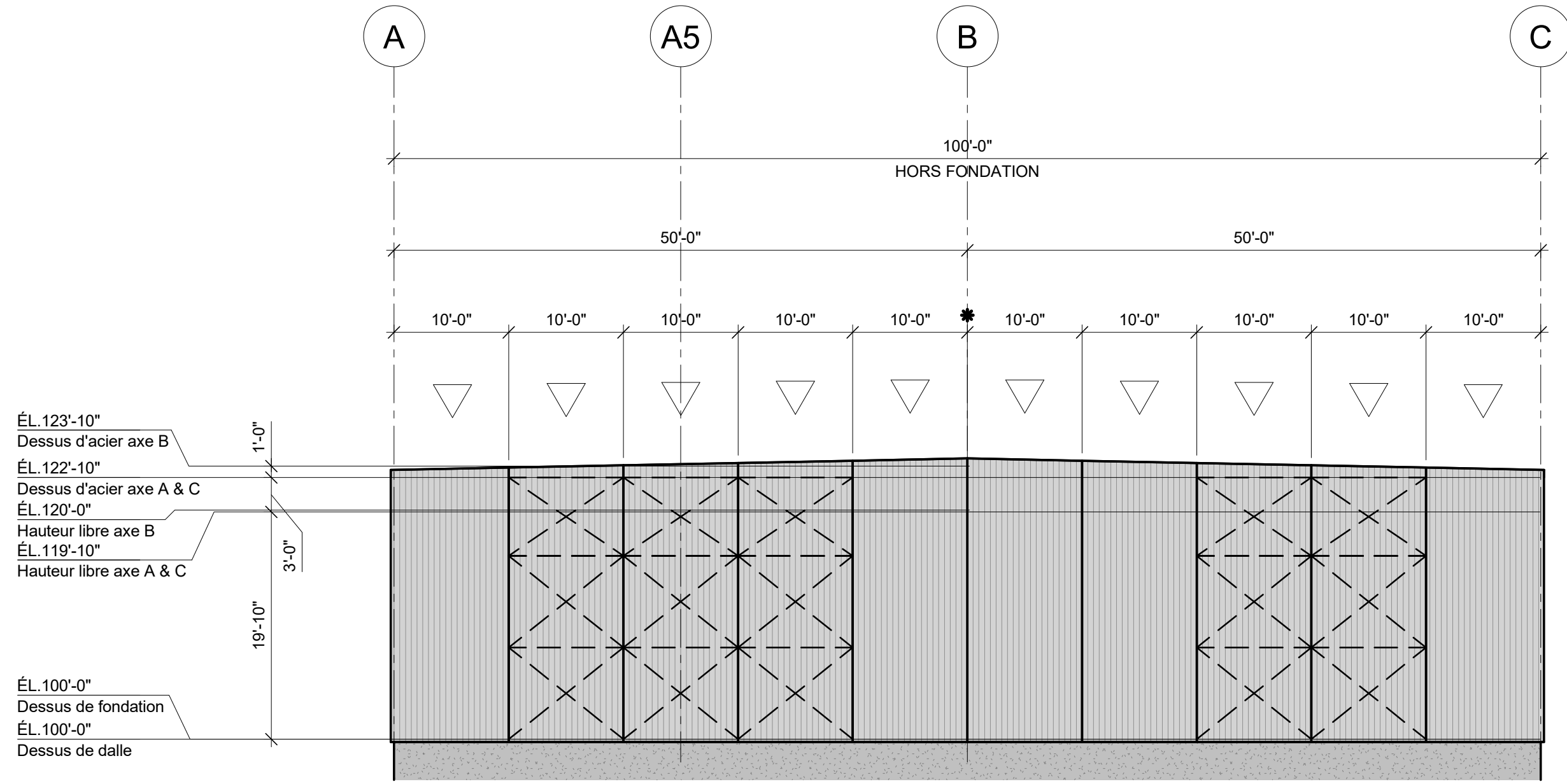
ÉLEVATION AXE 7 (SUD) 3/32" = 1'-0"
