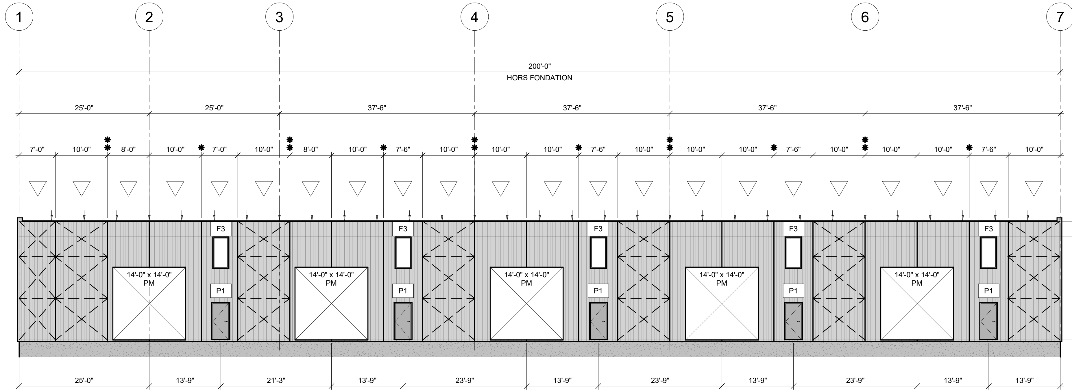
ÉLEVATION AXE A (OUEST) 3/32" = 1'-0"
