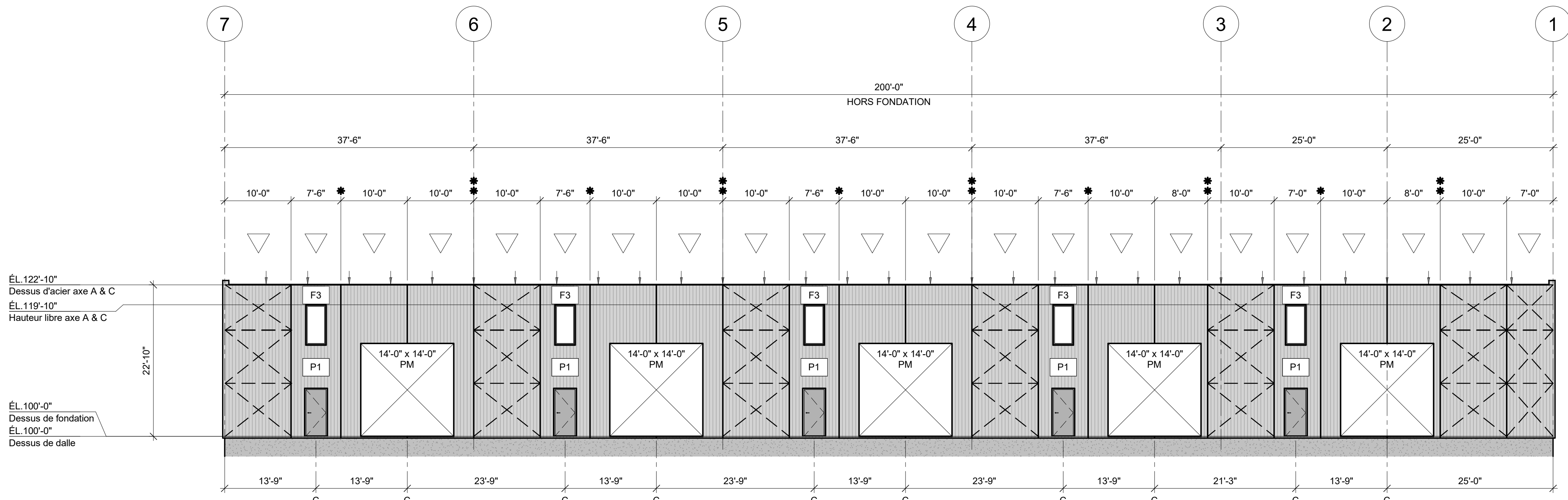
ÉLEVATION AXE C (EST) 3/32" = 1'-0"
