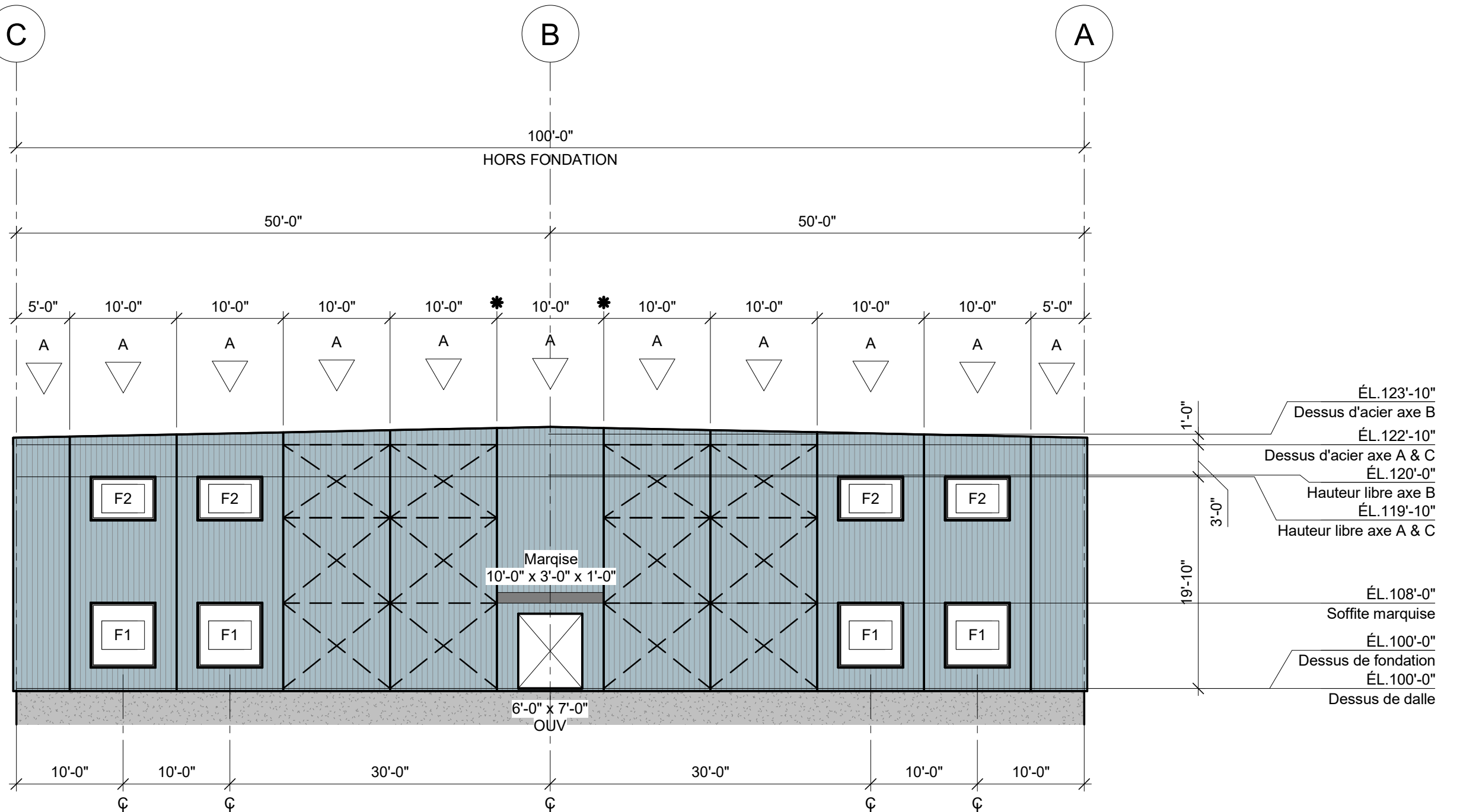
ÉLEVATION AXE 1 (NORD) 3/32" = 1'-0"
