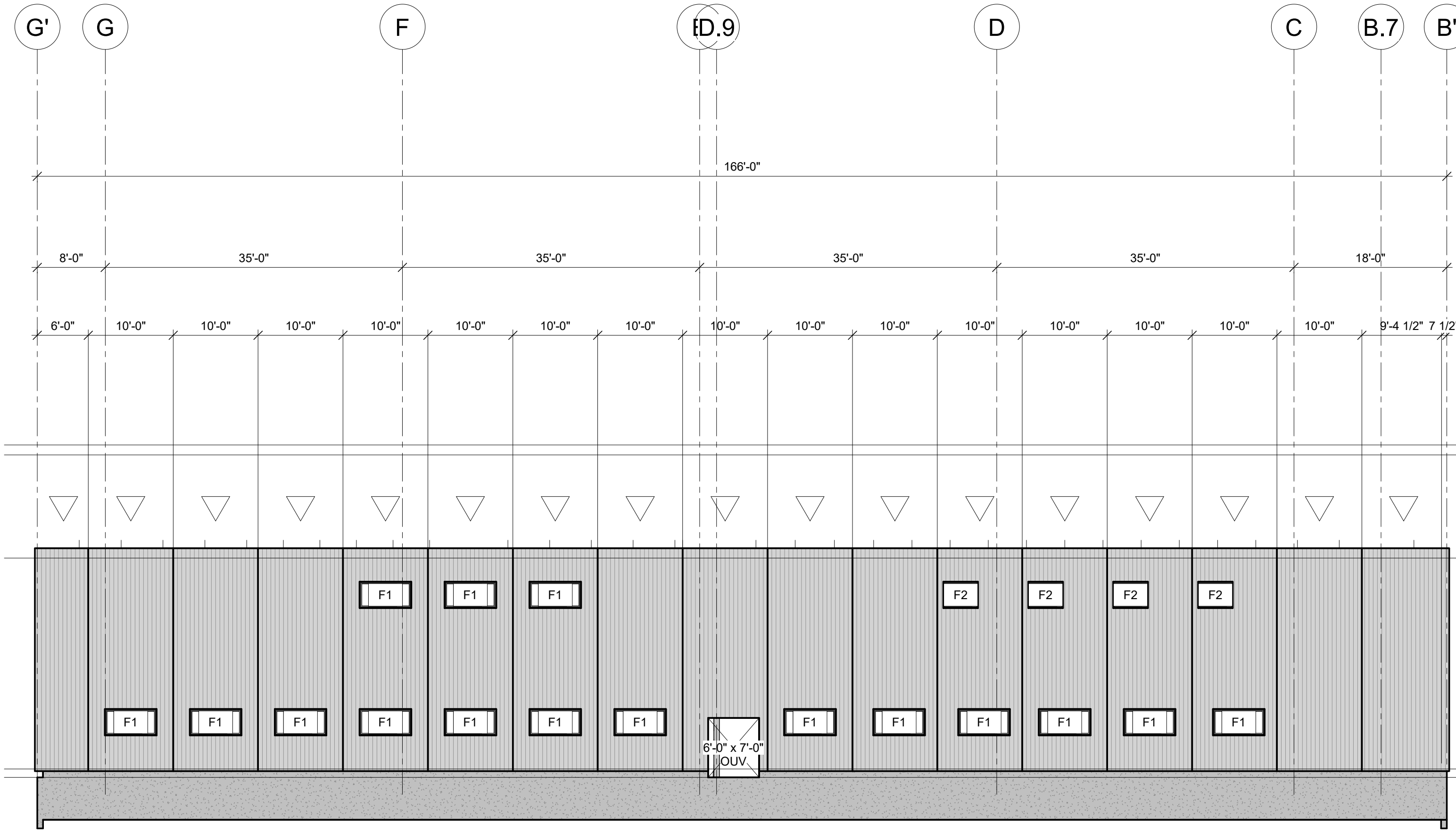
ÉLÉVATION AXE 1 (EST) 3/32" = 1'-0"
