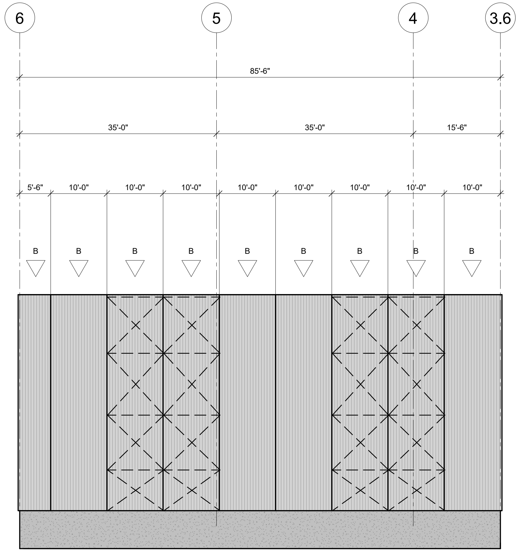
ÉLÉVATION AXE K (SUD) 3/32" = 1'-0"
