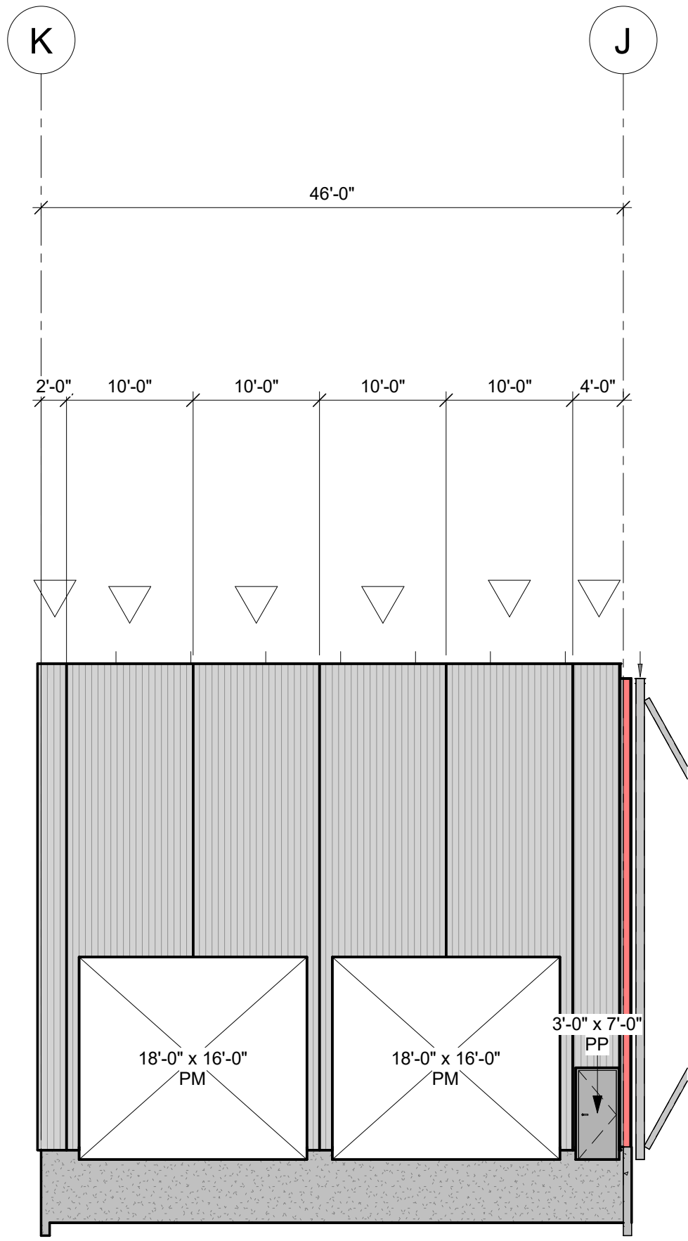
ÉLÉVATION AXE 3.6 (EST) 3/32" = 1'-0"
