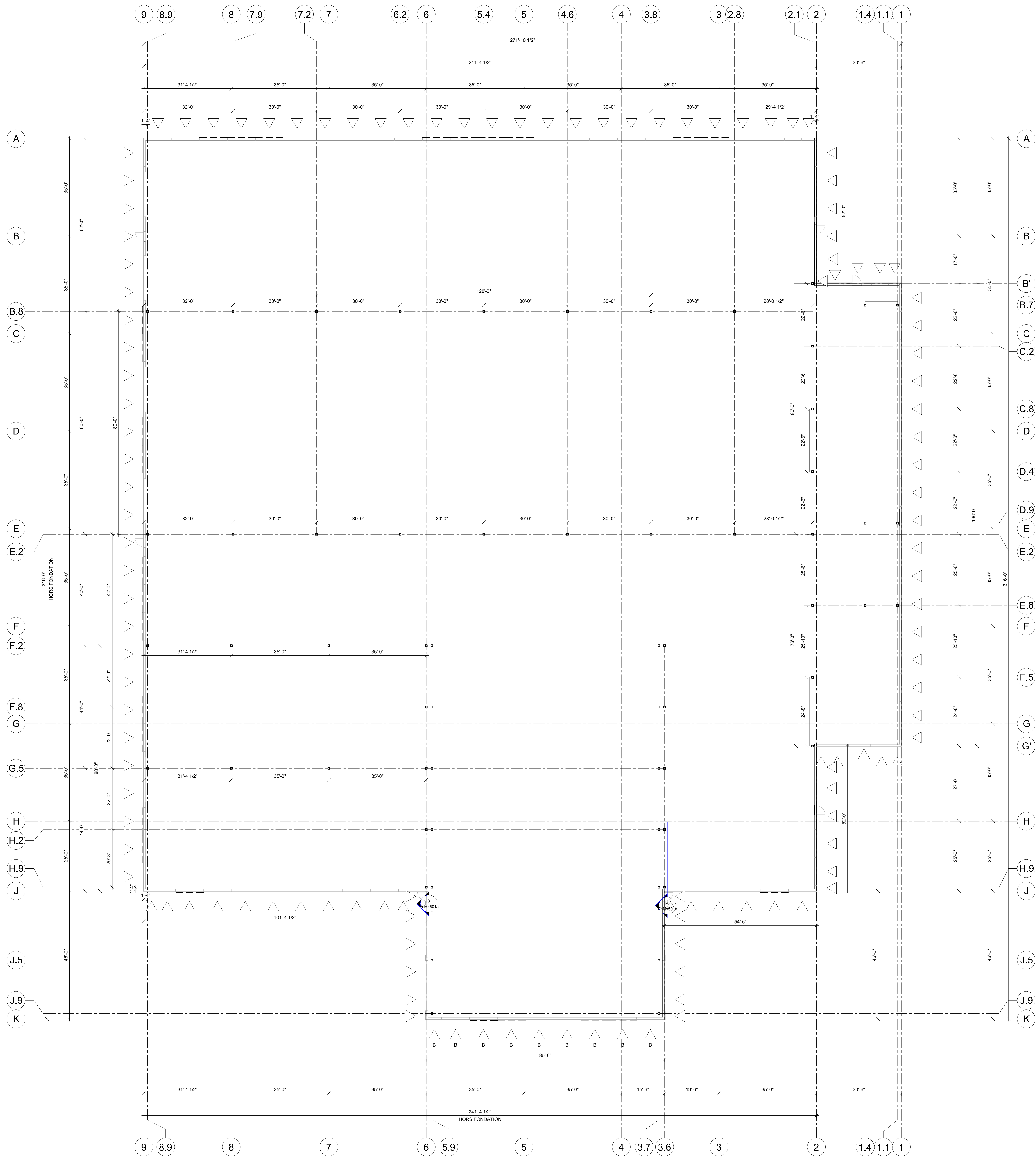
PLAN D'ANCRAGE
