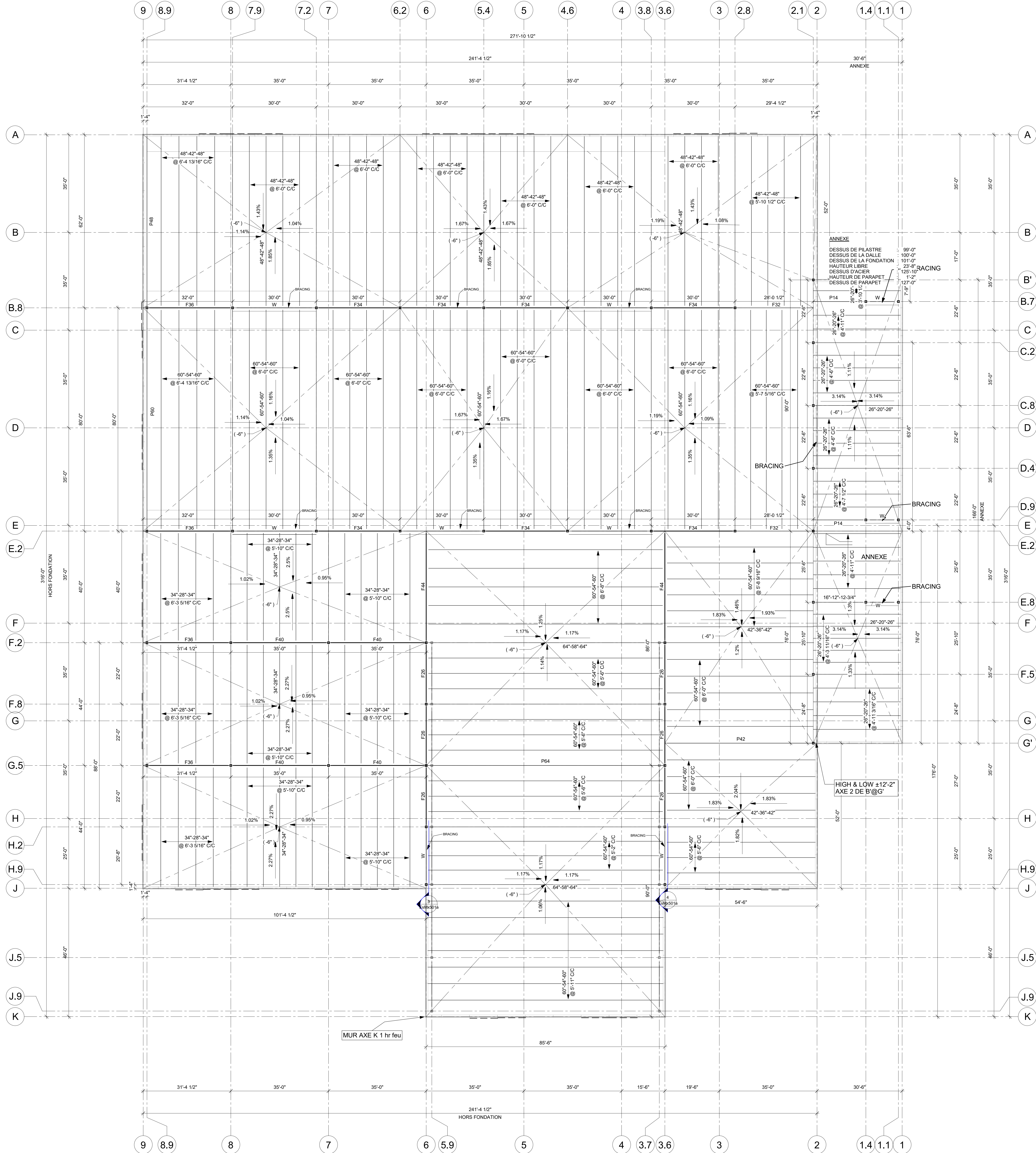
PLAN DE TOIT
