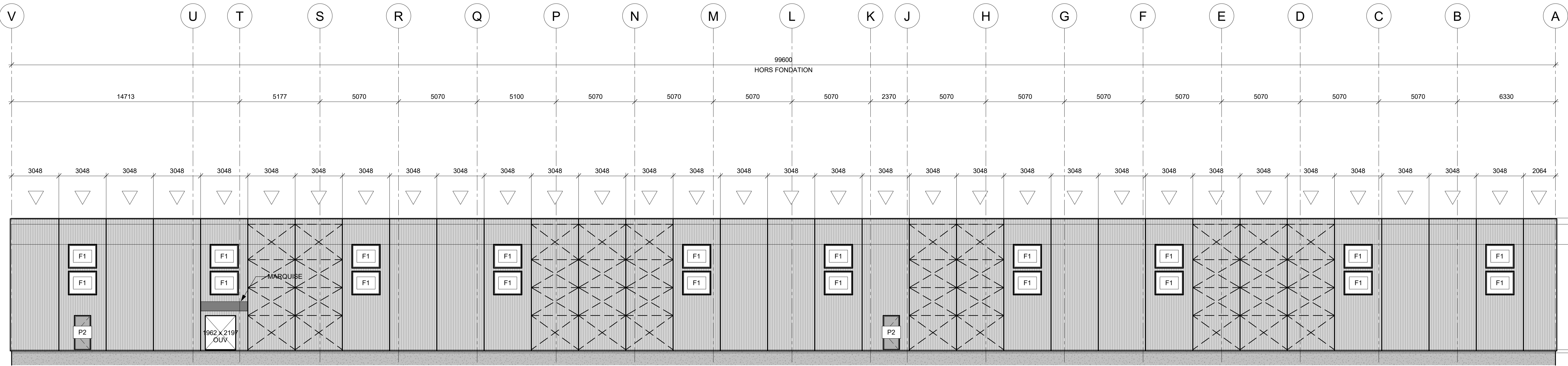
ÉLÉVATION AXE 1 (NORD) 1 : 125
