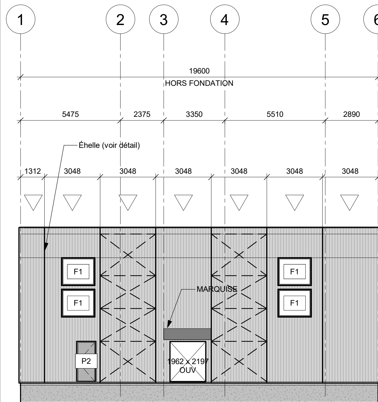
ÉLÉVATION AXE A (OUEST) 1 : 125
