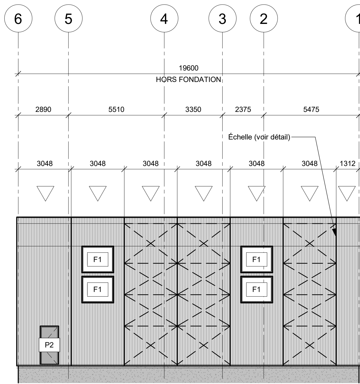
ÉLÉVATION AXE V (EST) 1 : 125
