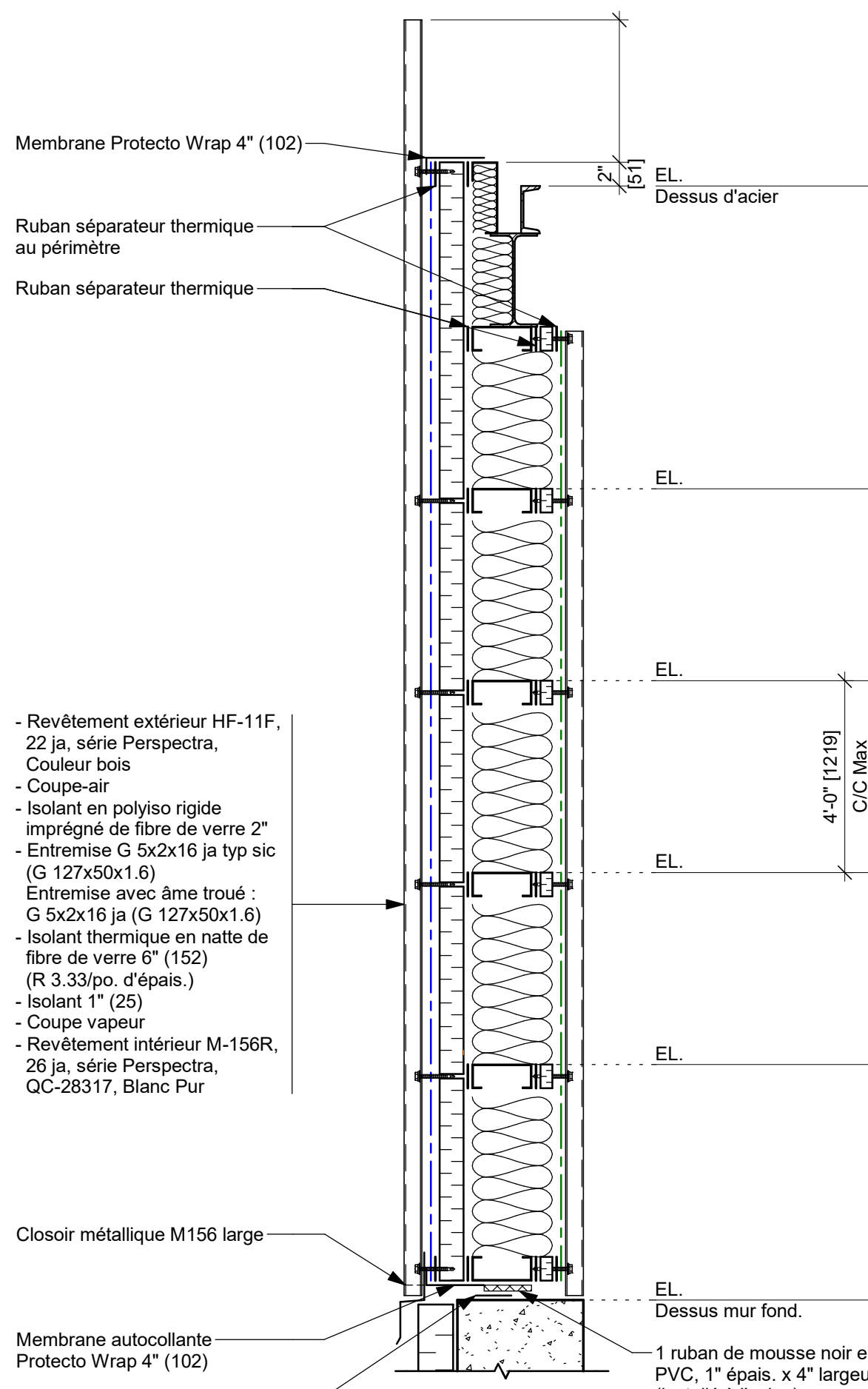
Panneaux Murox Ci R-25 Type "B"
