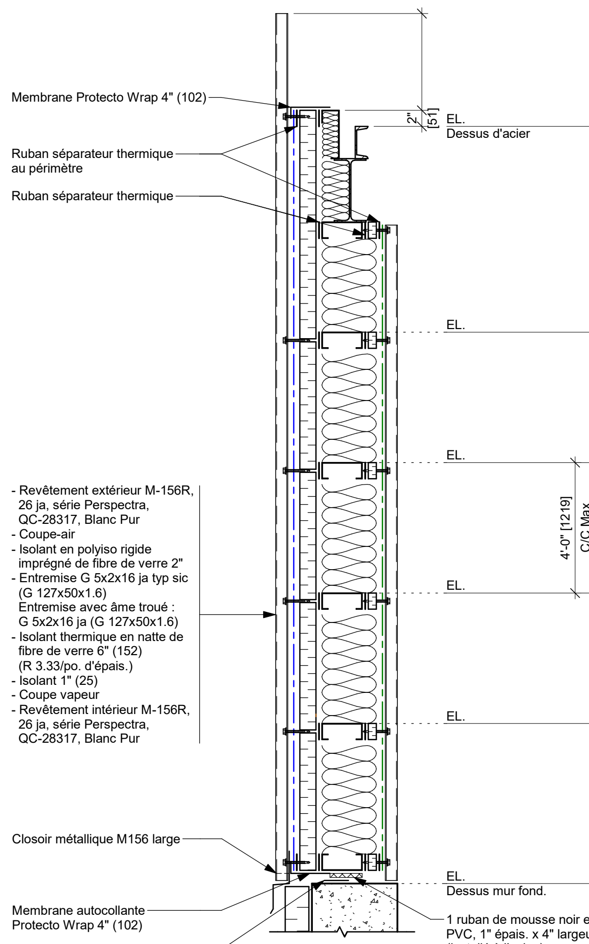
Panneaux Murox Ci R-25 Typique
