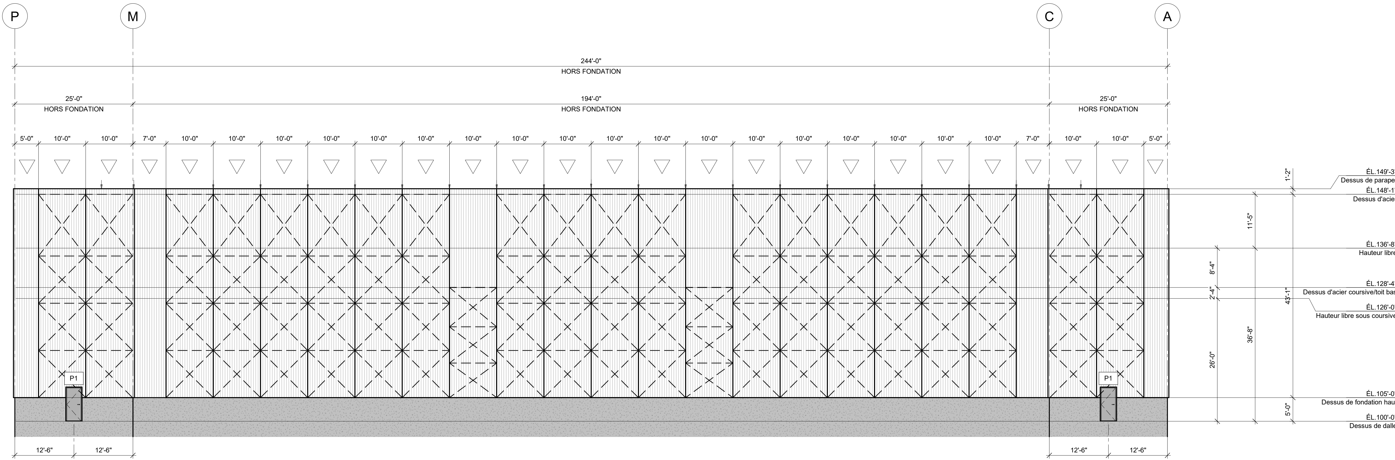
ÉLÉVATION AXE 1 & 2 (OUEST) 3/32" = 1'-0"
