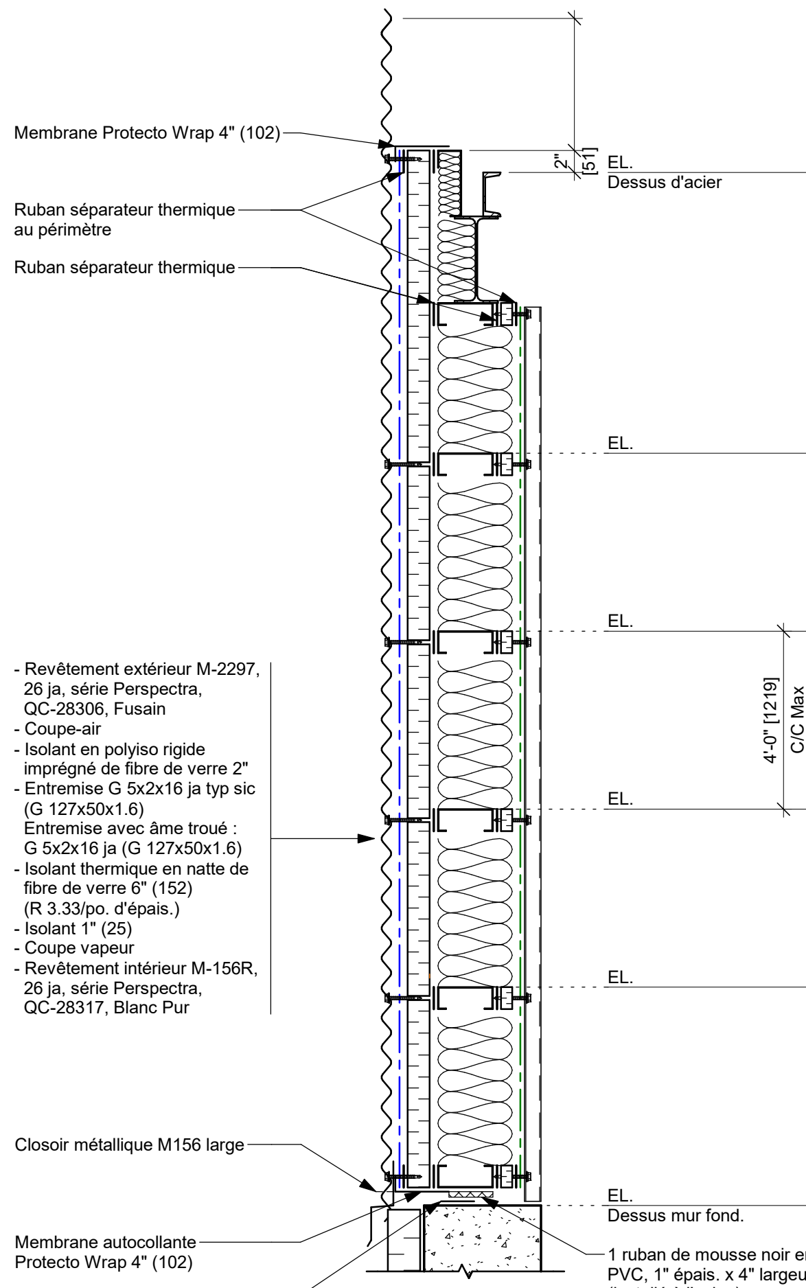
Panneaux Murox Ci R-25 Type "C"
