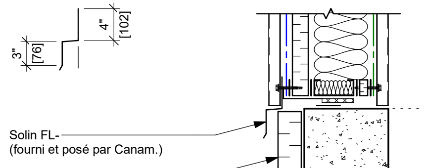
Panneau Murox "Standard" R-25 (base avec isolant)
