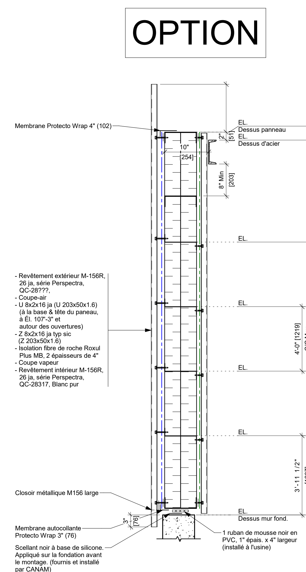
COUPE DE MUR EN OPTION 1" = 1'-0"
