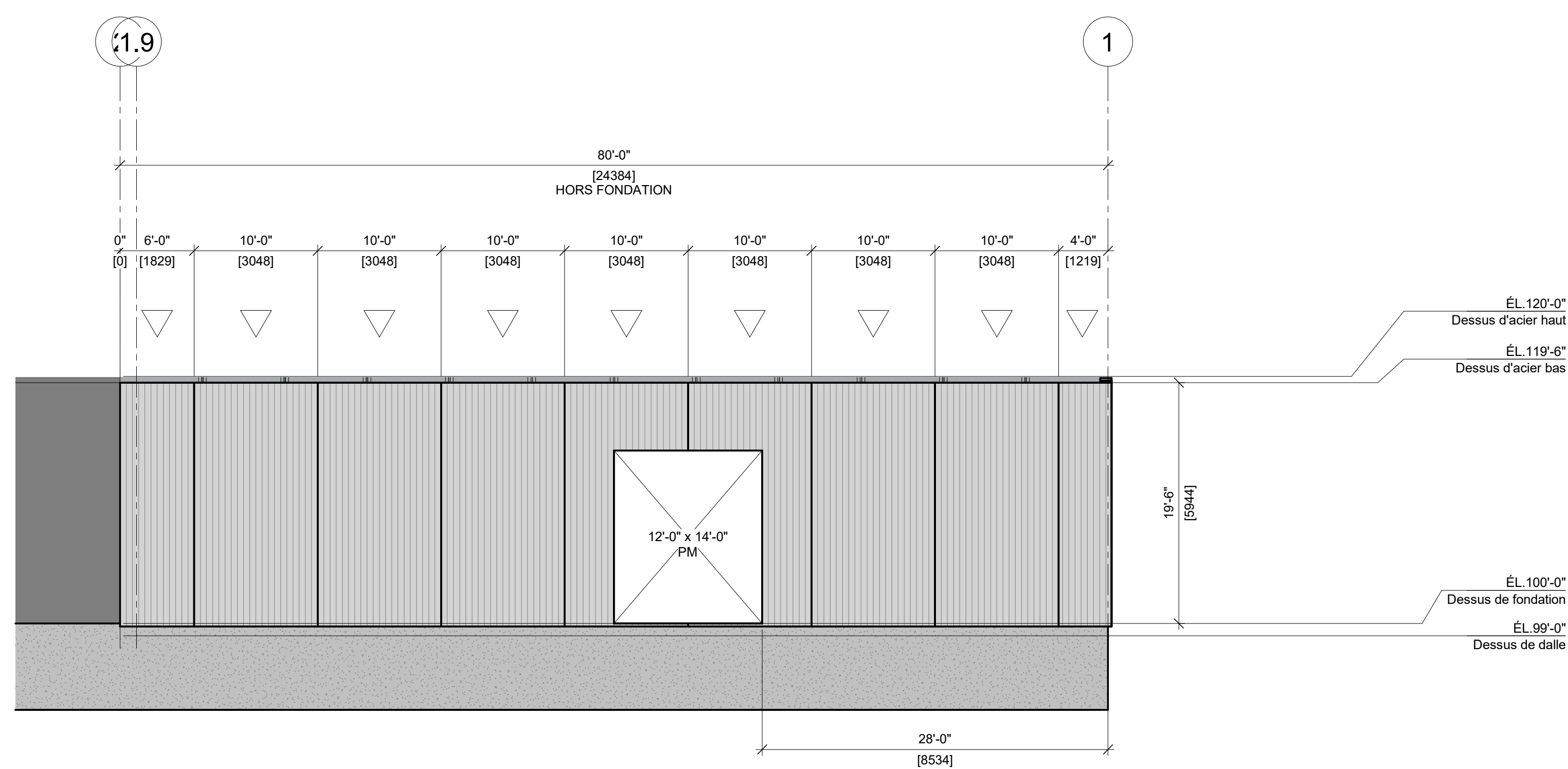
ÉLÉVATION AXE B (NORD) 1/8" = 1'-0"
