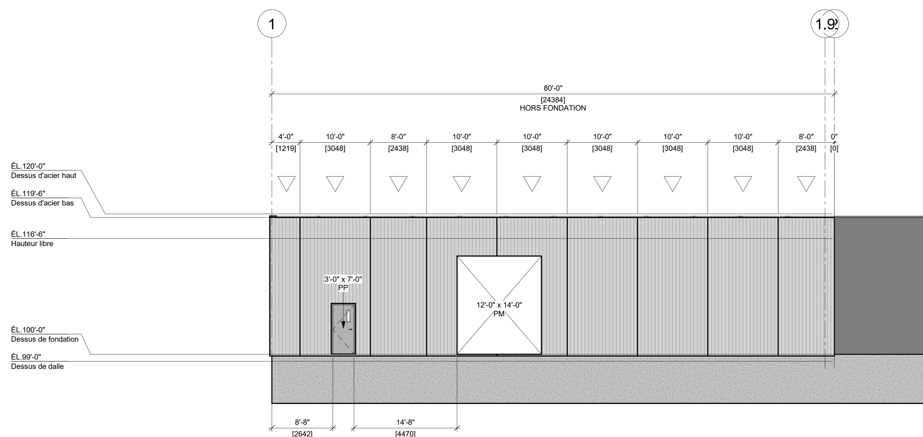
ÉLÉVATION AXE A (SUD) 1/8" = 1'-0"
