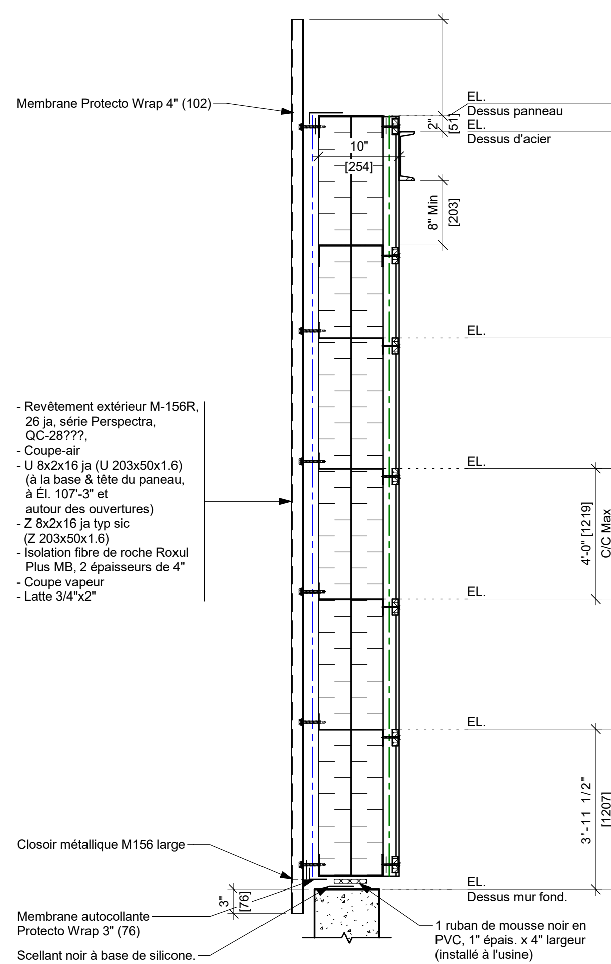
COUPE DE MUR PROPOSÉE 1" = 1'-0"
