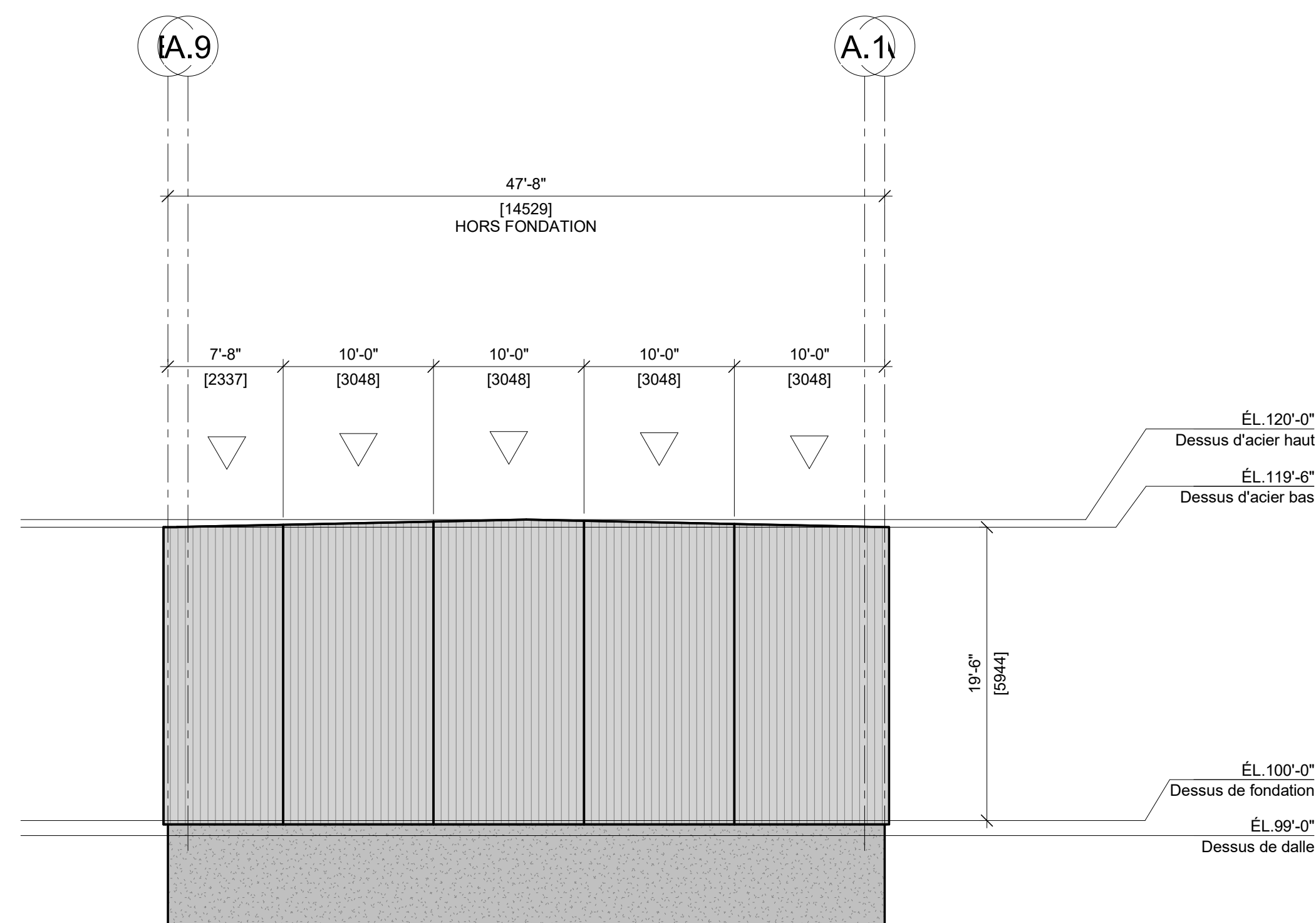
ÉLÉVATION AXE 1 (OUEST) 1/8" = 1'-0"
