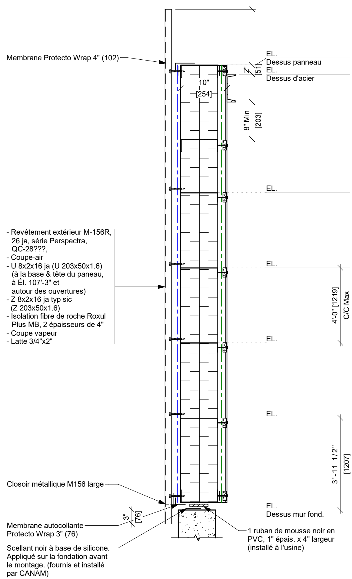
COUPE DE MUR PROPOSÉE 1" = 1'-0"
