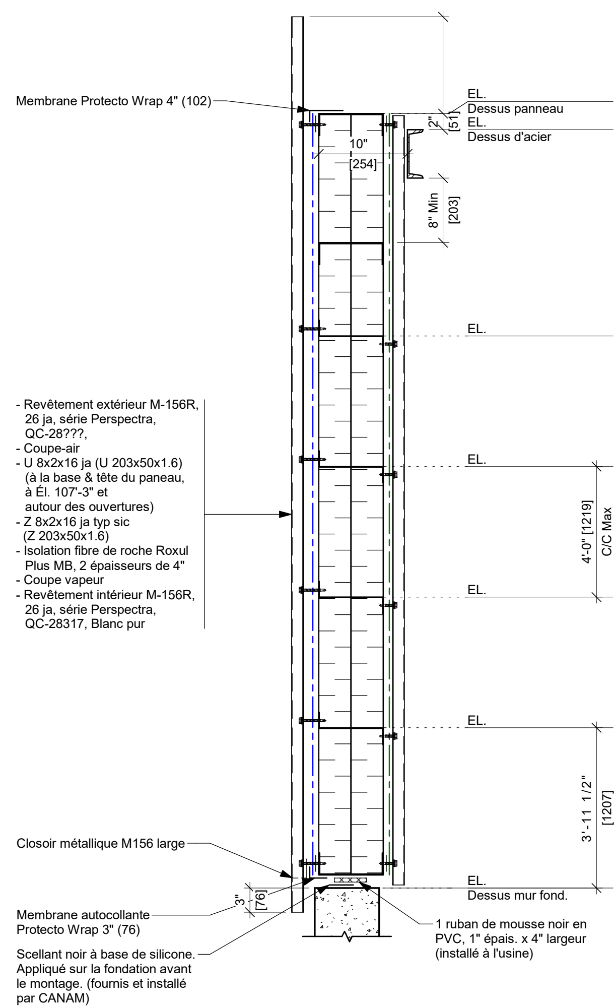
COUPE DE MUR EN OPTION 1" = 1'-0"
