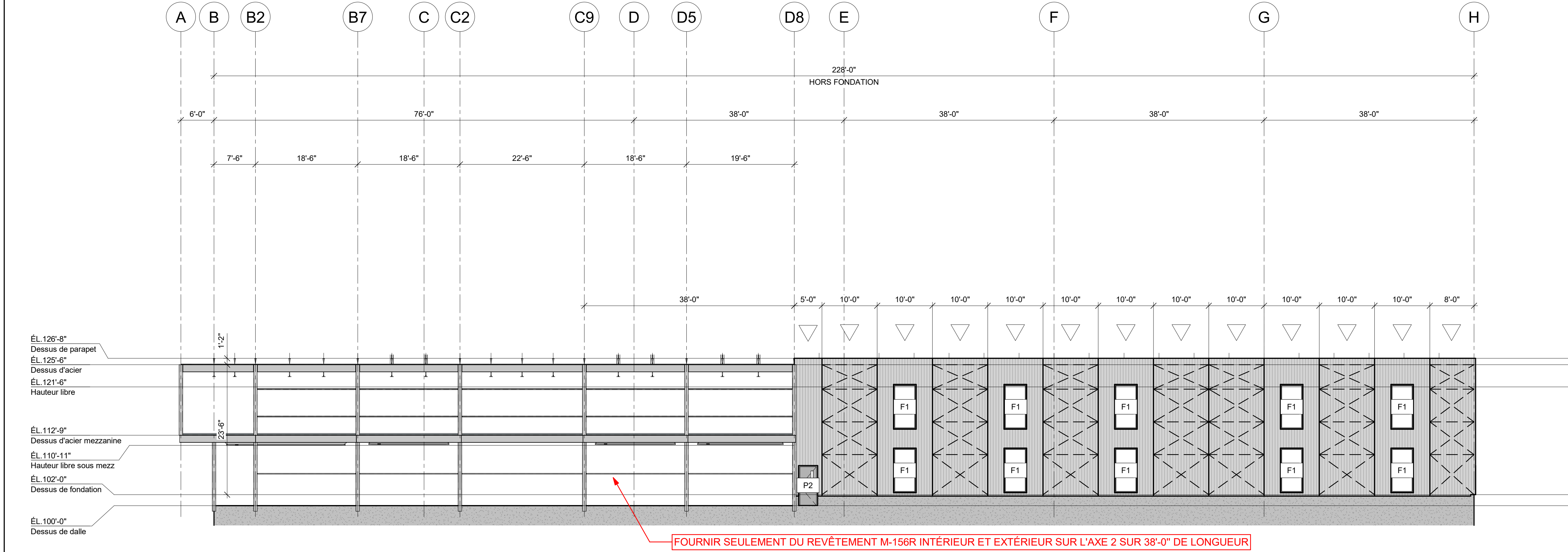
ÉLÉVATION AXE 1 & 2 (SUD) 3/32" = 1'-0"
