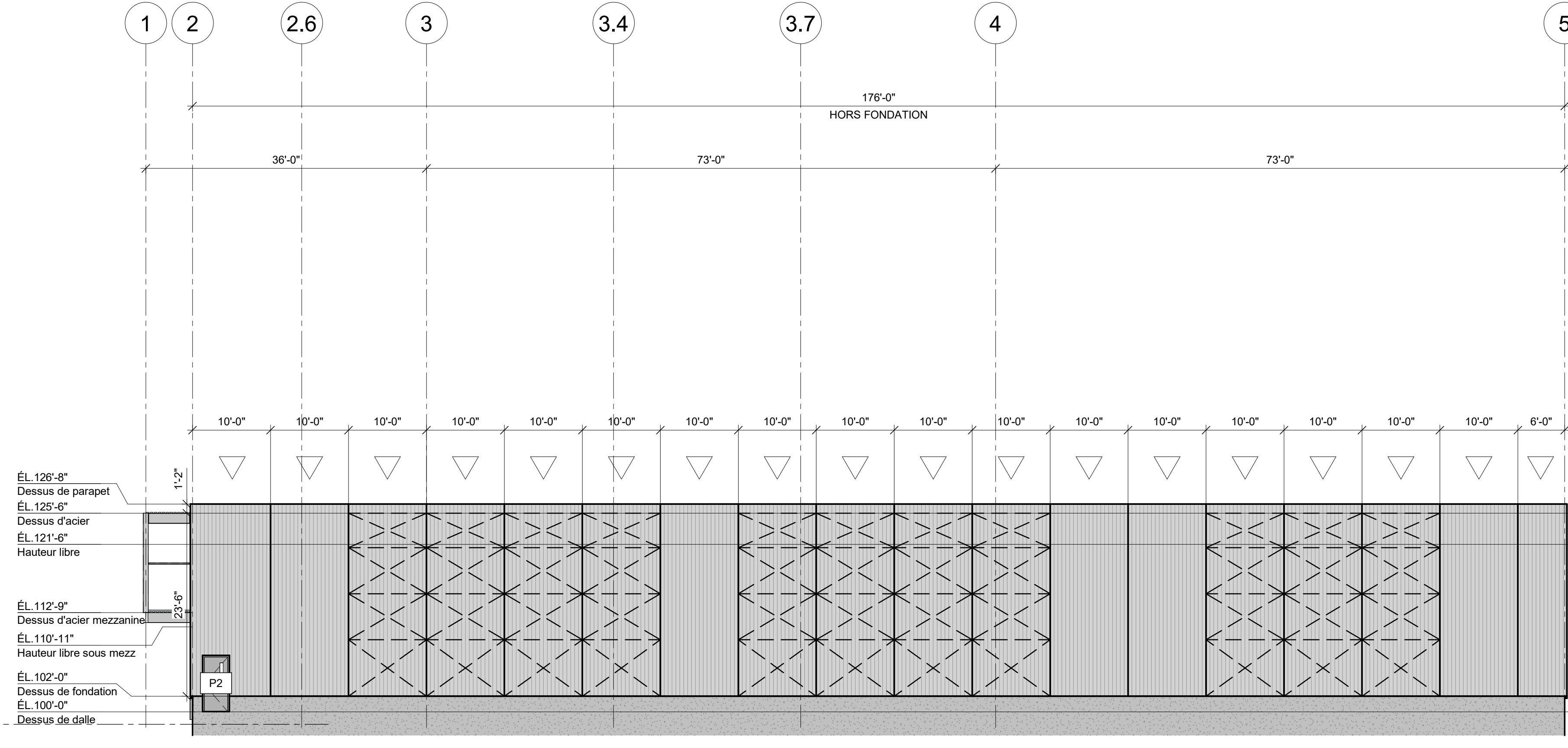
ÉLEVATION AXE D8 & H (EST) 3/32" = 1'-0"
