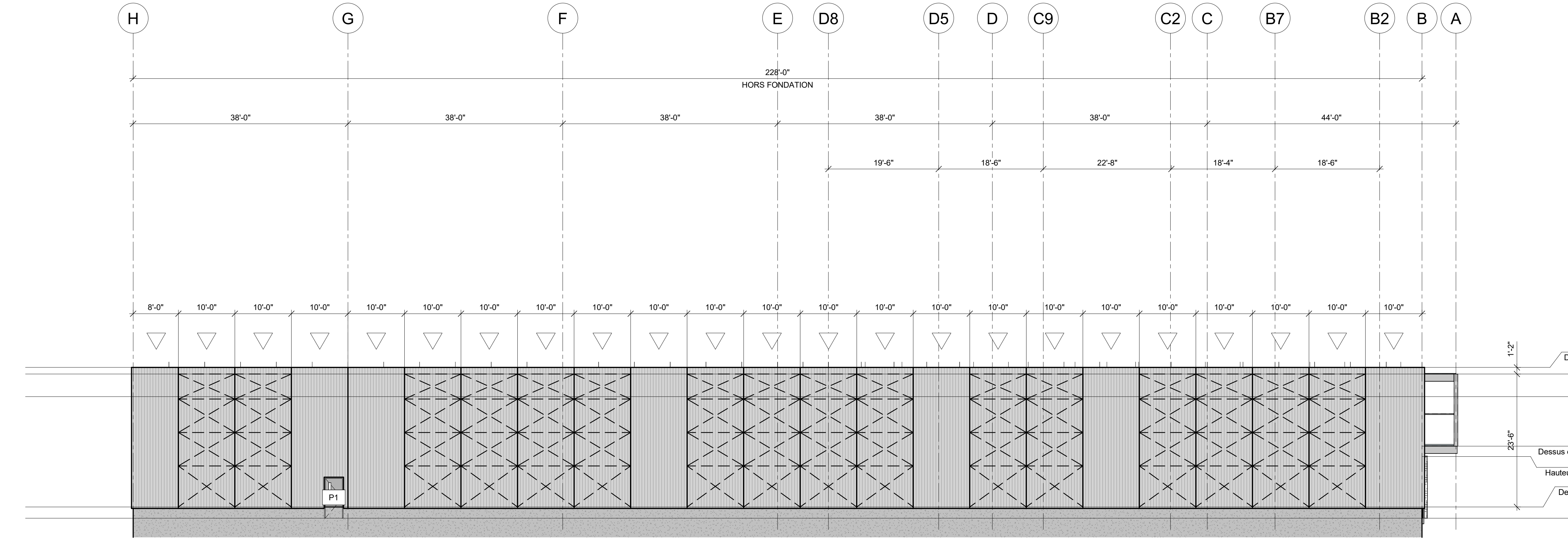
ÉLEVATION AXE 3 & 5 (NORD) 3/32" = 1'-0"
