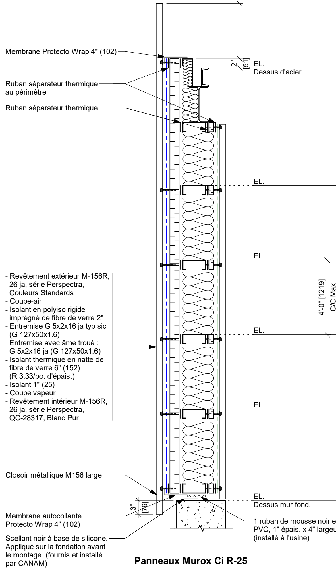
COUPE DE MUR - TYPE 1" = 1'-0"
