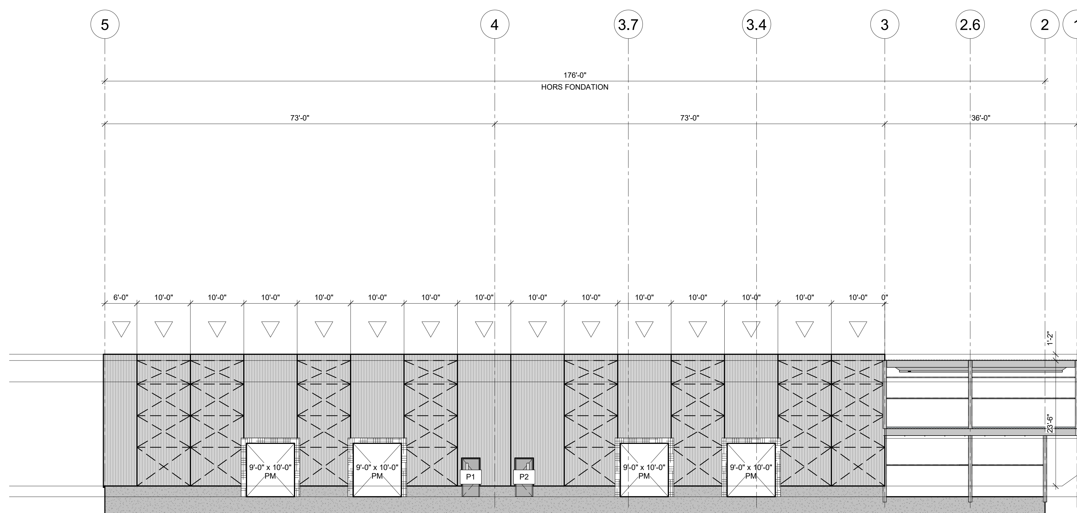
ÉLEVATION AXE 1 & 2 (SUD) 3/32" = 1'-0"
