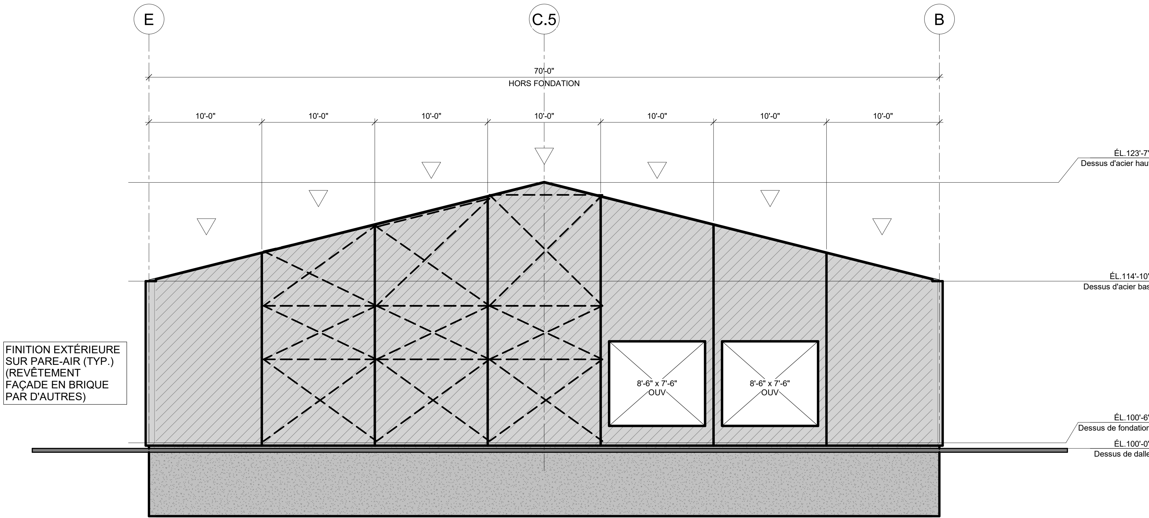
ÉLEVATION AXE 1 (OUEST) 3/16" = 1'-0"
