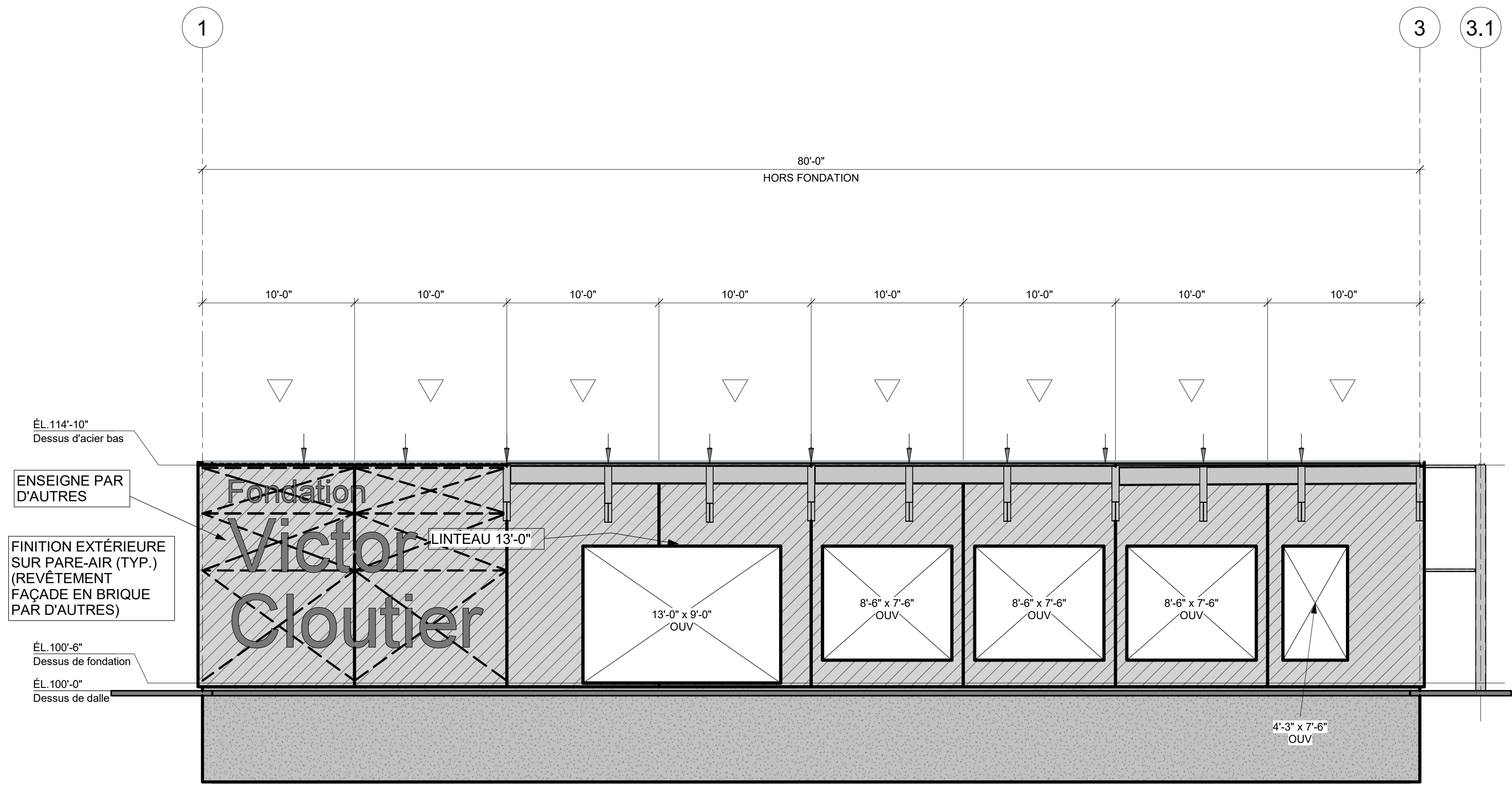
ÉLEVATION AXE B (SUD) 3/16" = 1'-0"
