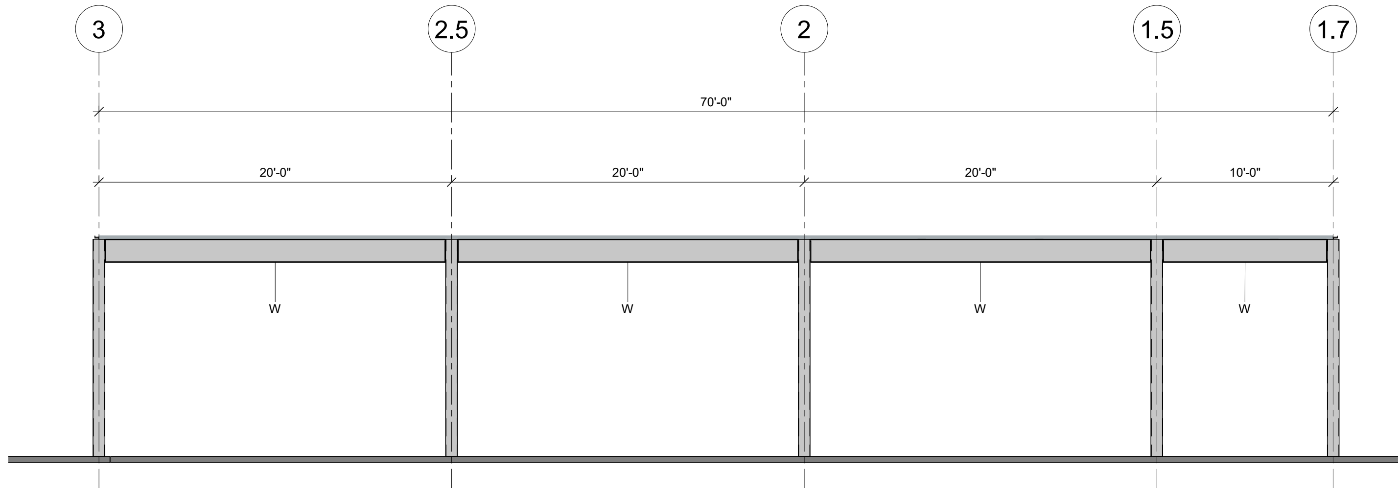
ÉLEVATION AXE E.1 (STRUCTURE BALCON #2) 3/16" = 1'-0"
