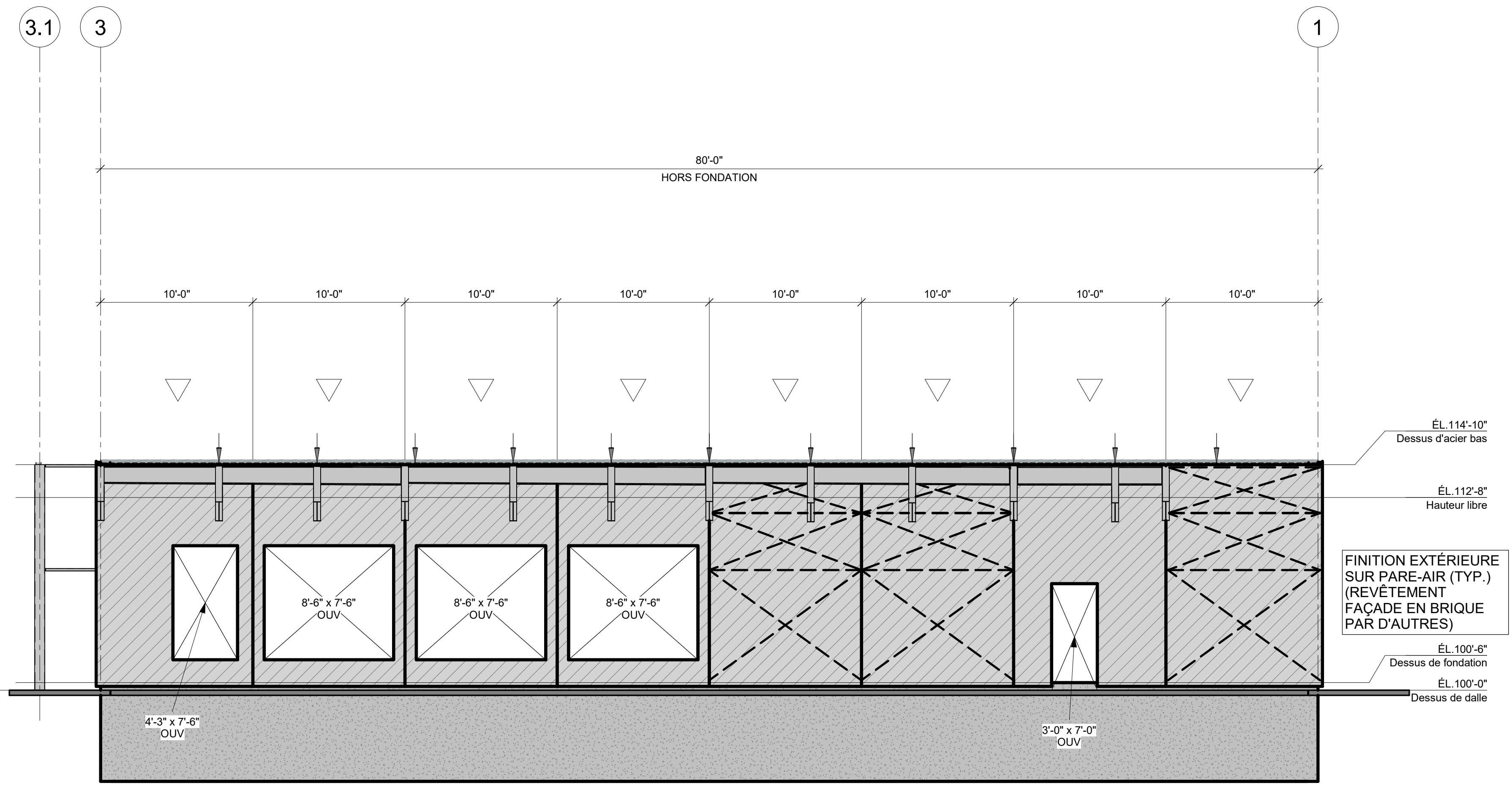
ÉLEVATION AXE E (NORD) 3/16" = 1'-0"
