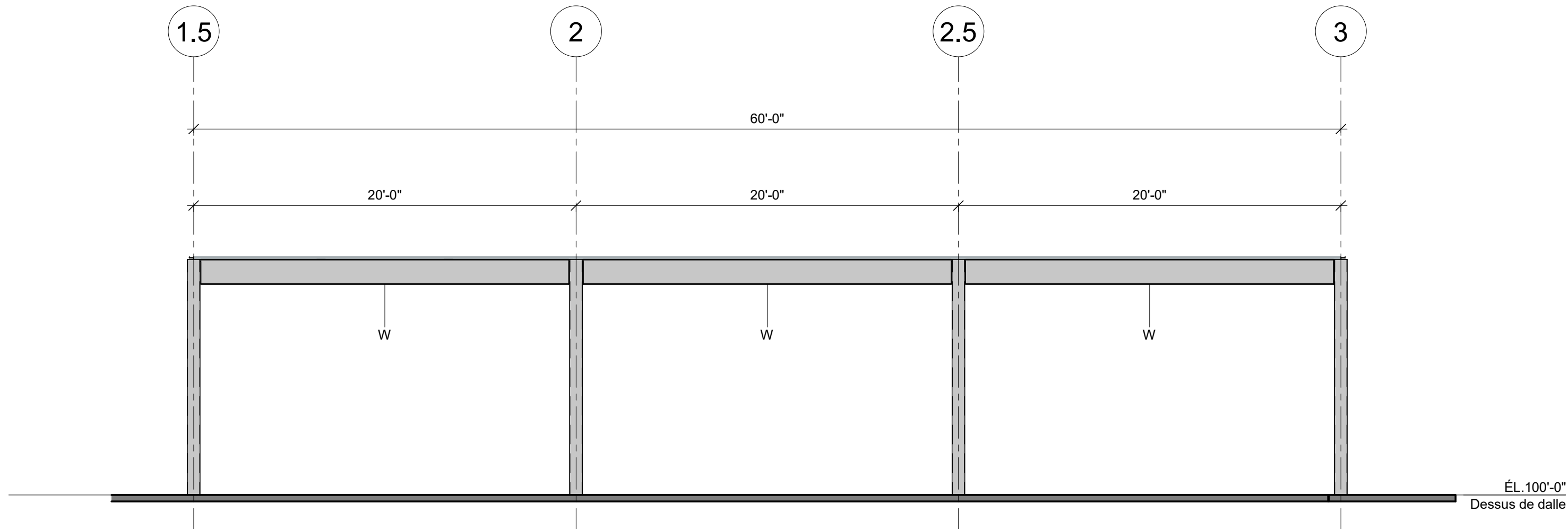
ÉLEVATION AXE A (STRUCTURE BALCON #1) 3/16" = 1'-0"
