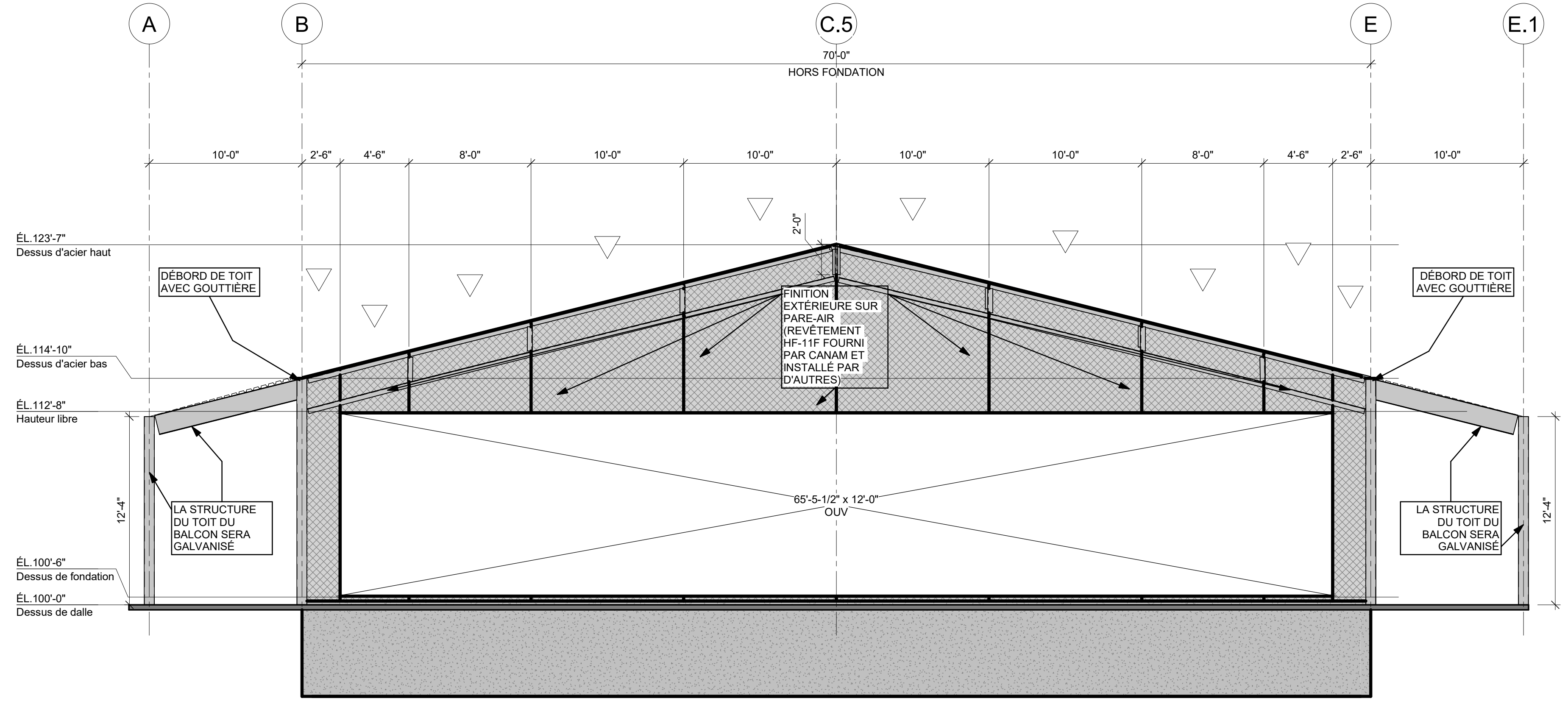
ÉLEVATION AXE 3 (EST) 3/16" = 1'-0"
