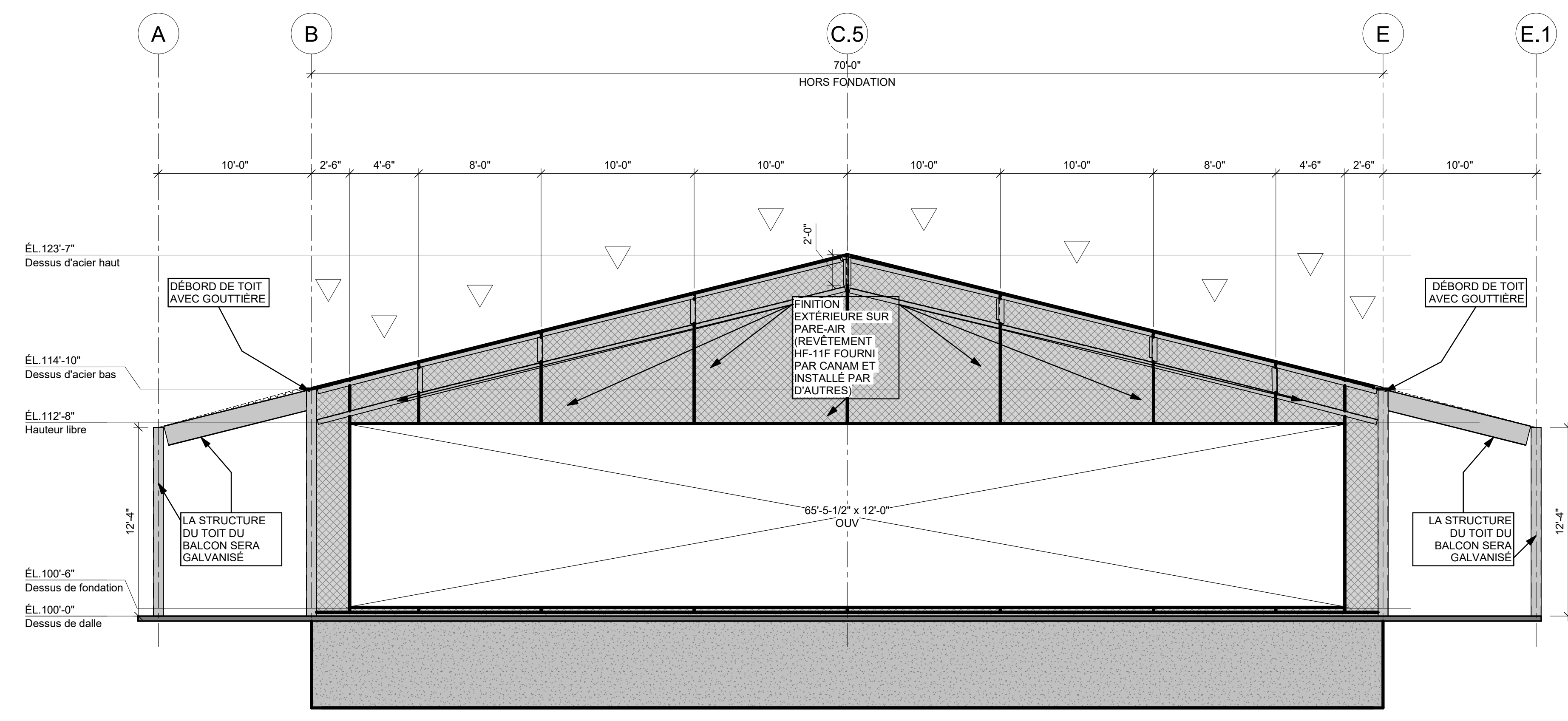
ÉLEVATION AXE 3 (EST) 3/16" = 1'-0"
