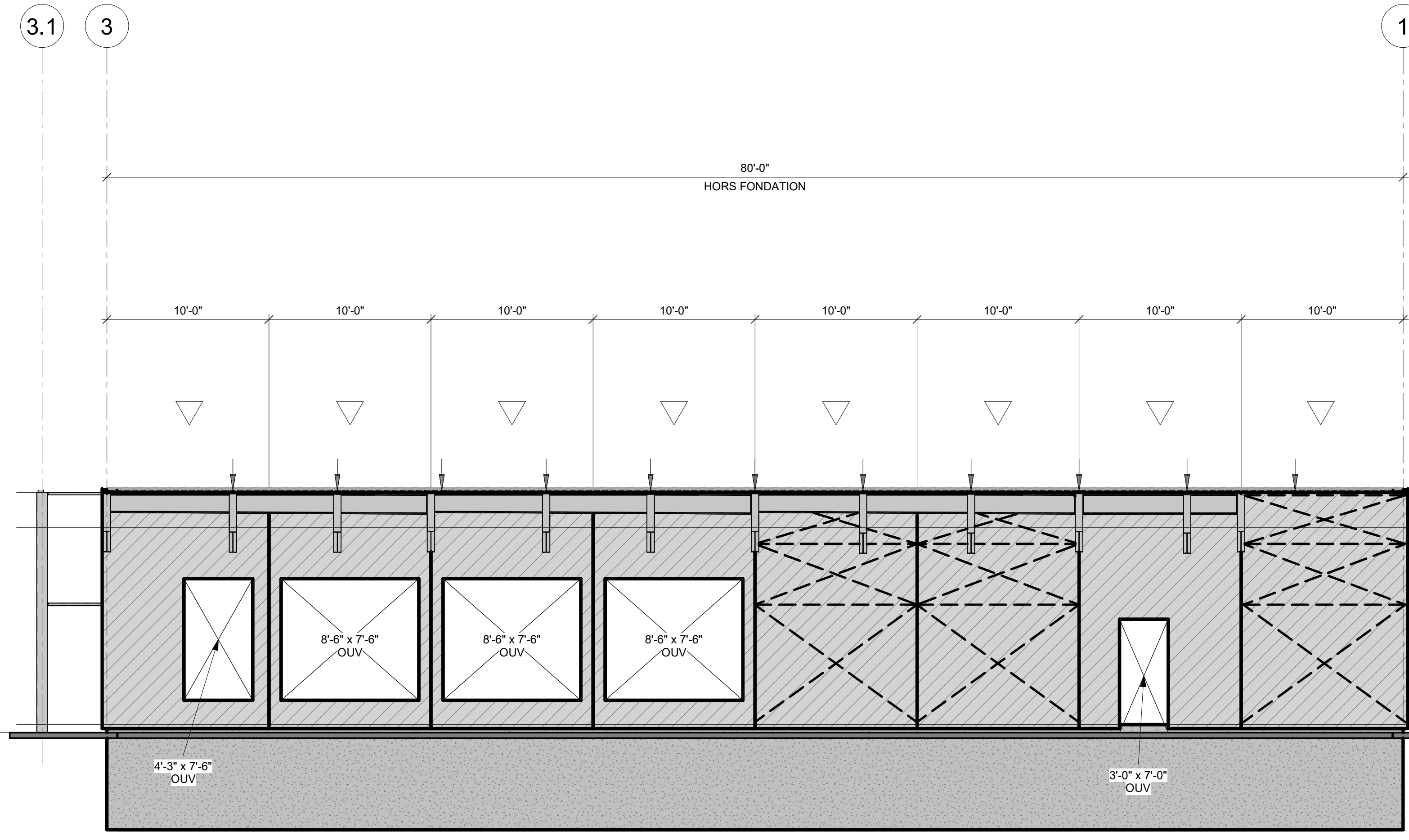
ÉLEVATION AXE E (NORD) 3/16" = 1'-0"
