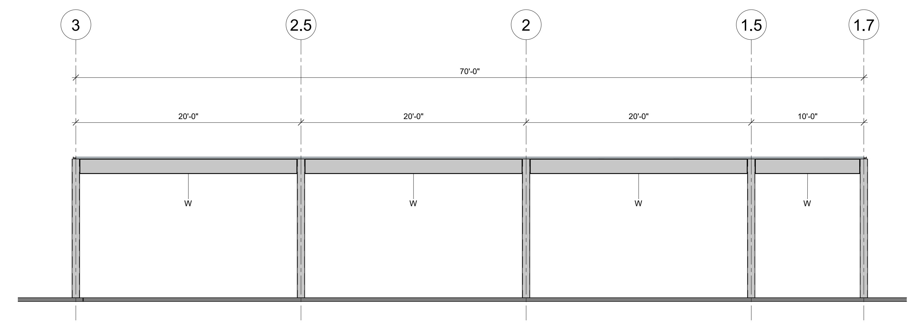
ÉLEVATION AXE E.1 (STRUCTURE BALCON #2) 3/16" = 1'-0"
