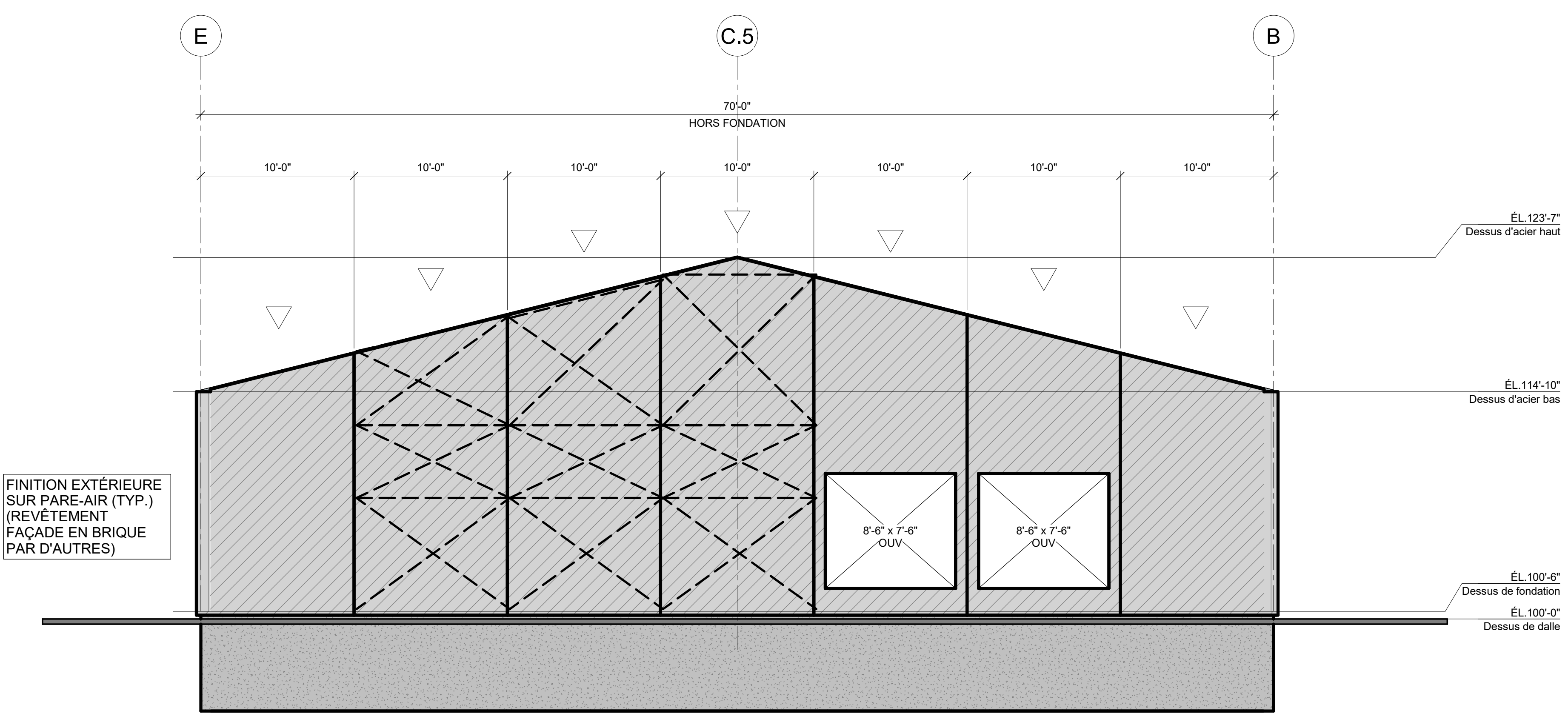
ÉLEVATION AXE 1 (OUEST) 3/16" = 1'-0"
