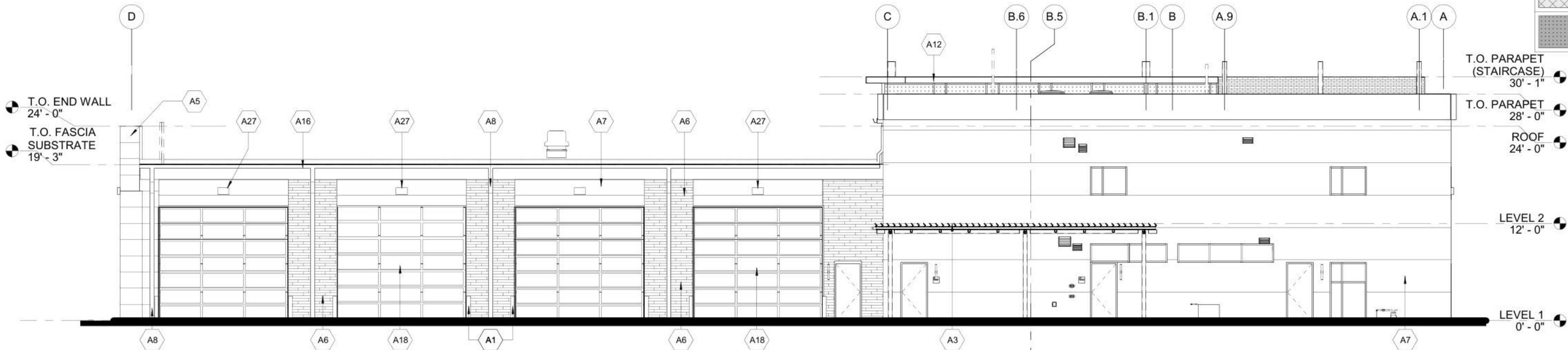
A1 NORTH ELEVATION SCALE: 1/8" = 1'-0"
