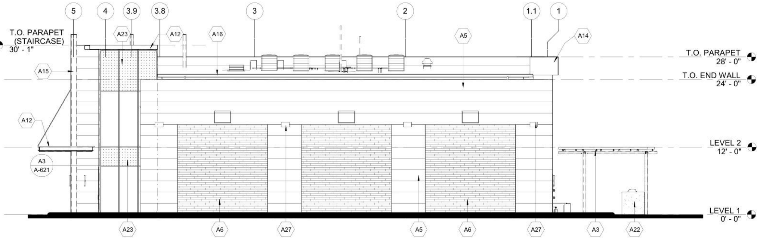
C1 EAST ELEVATION SCALE: 1/8" = 1'-0"
