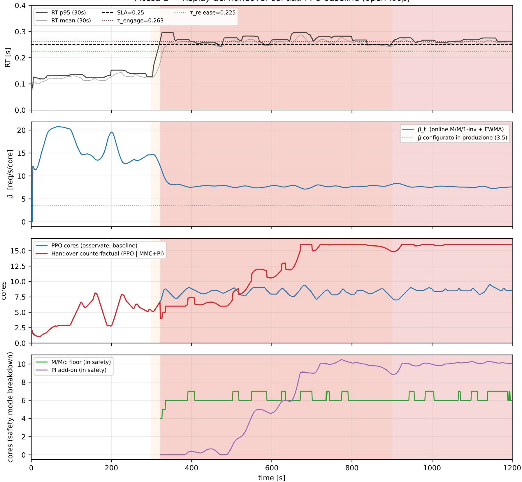
Mossa 1 — Replay del handover sui dati PPO baseline (open-loop)
