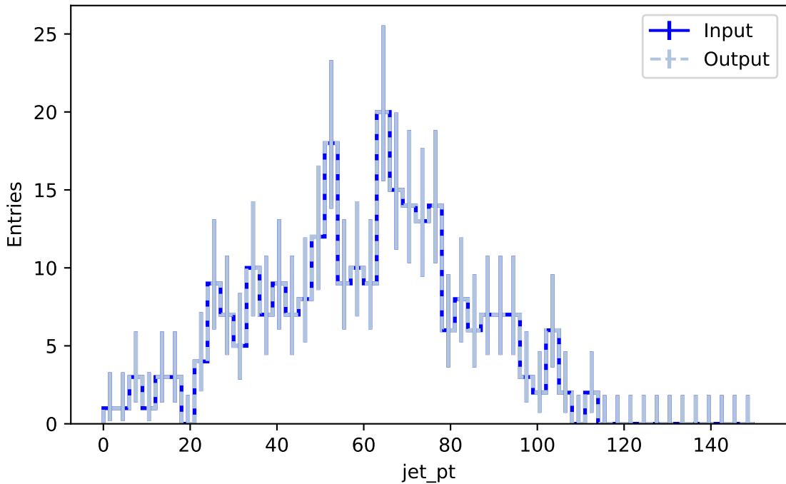
jet_pt
