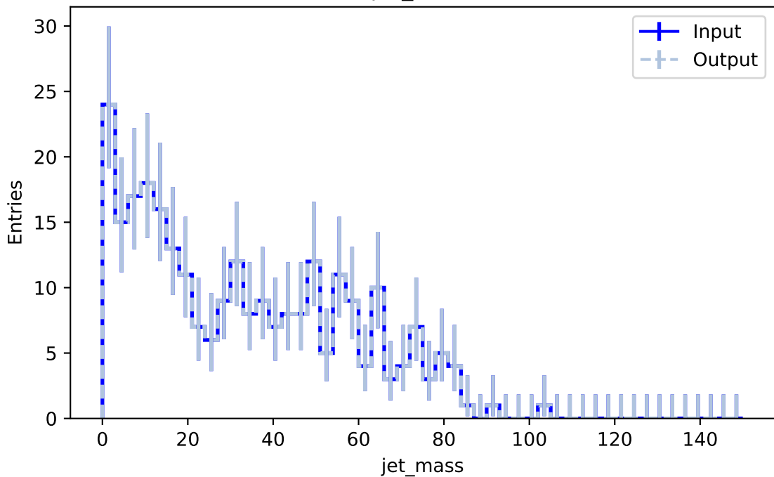
jet_mass
