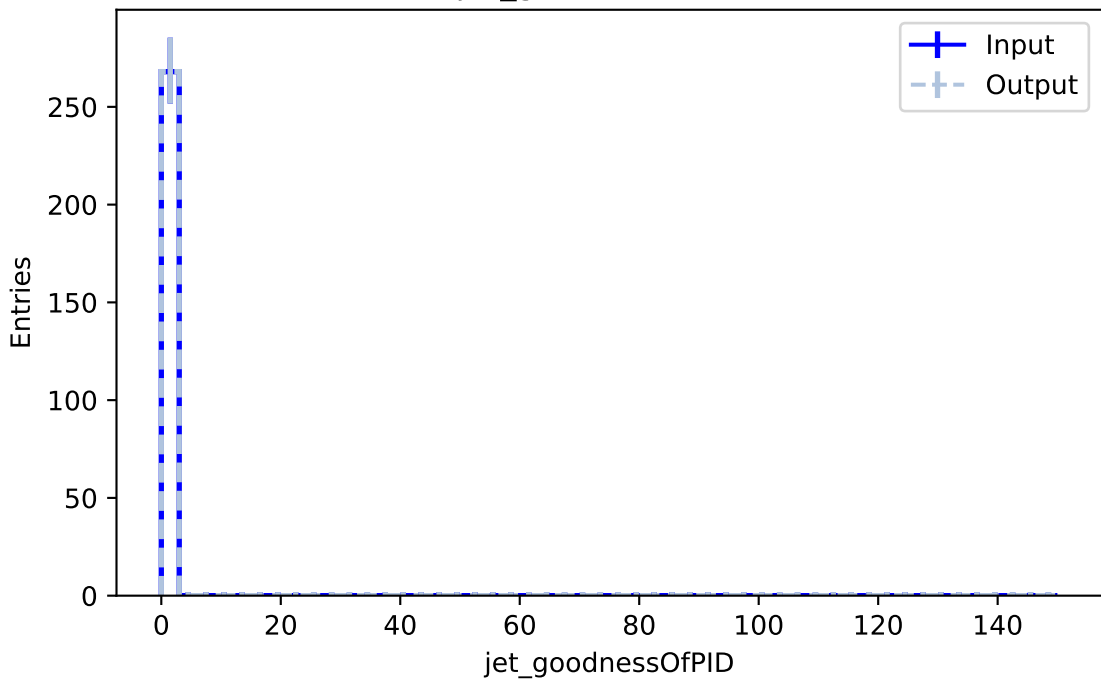
jet_goodnessOfPID
