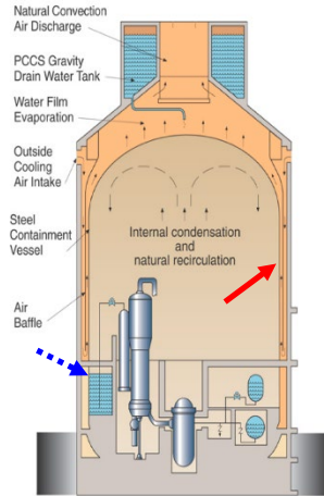
AP1000 PCCS
