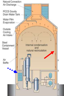
AP1000 PCCS
