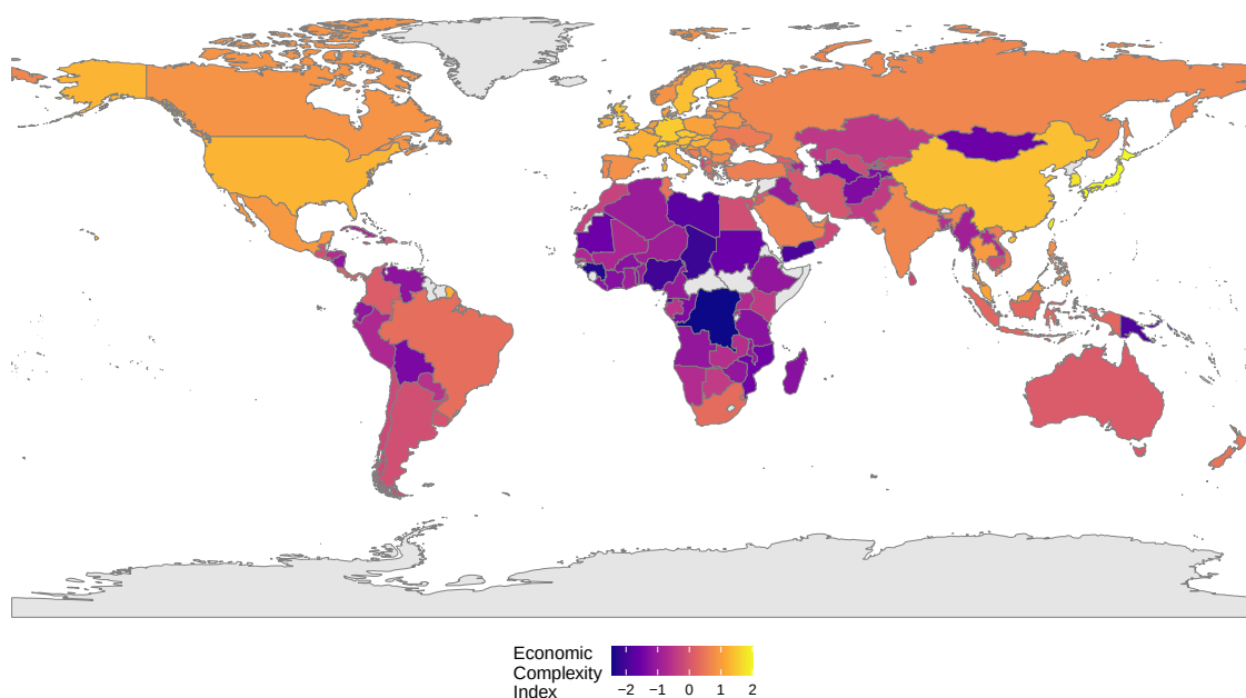
Figura A.16: Distribución global del Índice de Complejidad Económica (ECI).
