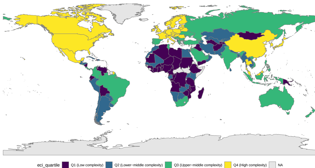
Figura A.17: Distribución global del Índice de Complejidad Económica (ECI) por cuartiles.
