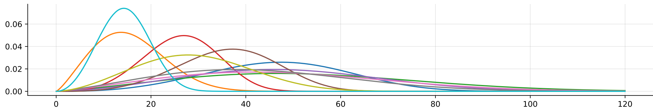
Bateman
