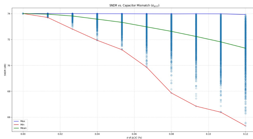
Figura 6: Mismatch entre os condensadores e influência na SNDR.
