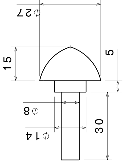
Shaft Scale: 1:1
