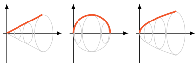
Rys. 2. Stożek, sfera i paraboloida eliptyczna. W każdym z tych przypadków mamy f(0) = 0 , co oznacza, że powierzchnia się „zamyka” – jak widać, da się to nawet zrobić gładko
